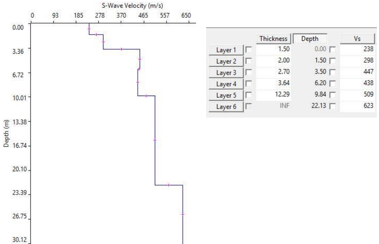
Fig. 6.16 Profilo Vs – MASW.02 – SCOPPIO 2
