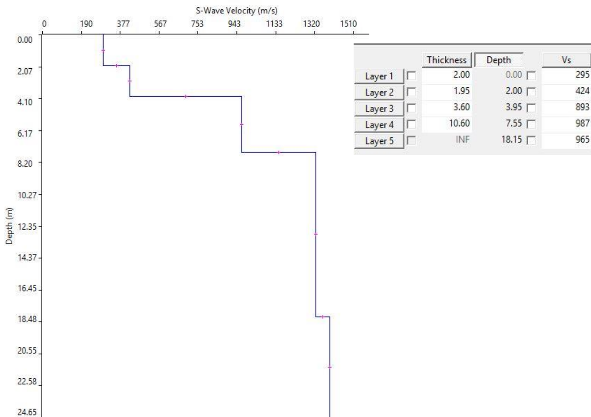
Fig. 6.8 Profilo Vs – MASW.01 – SCOPPIO 2
