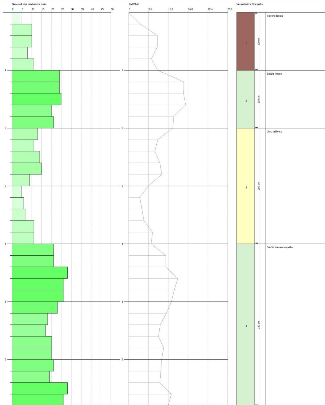
Fig. 6.18 Grafico di interpretazione stratigrafica – DPSH.02
