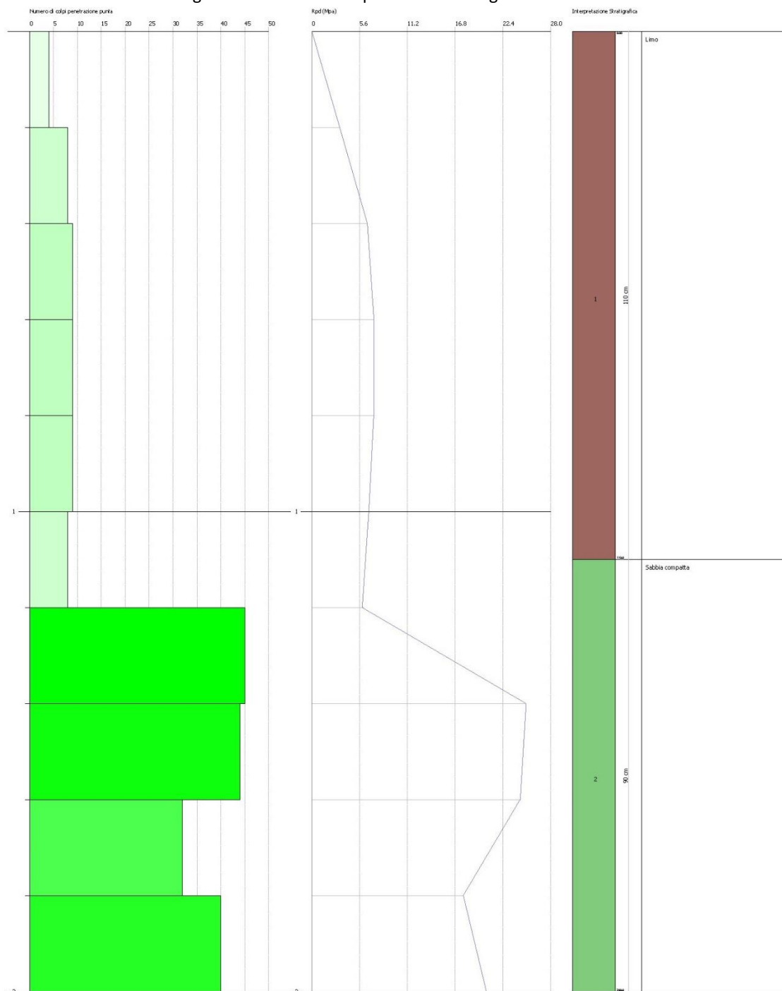
Fig. 6.17 Grafico di interpretazione stratigrafica – DPSH.01
