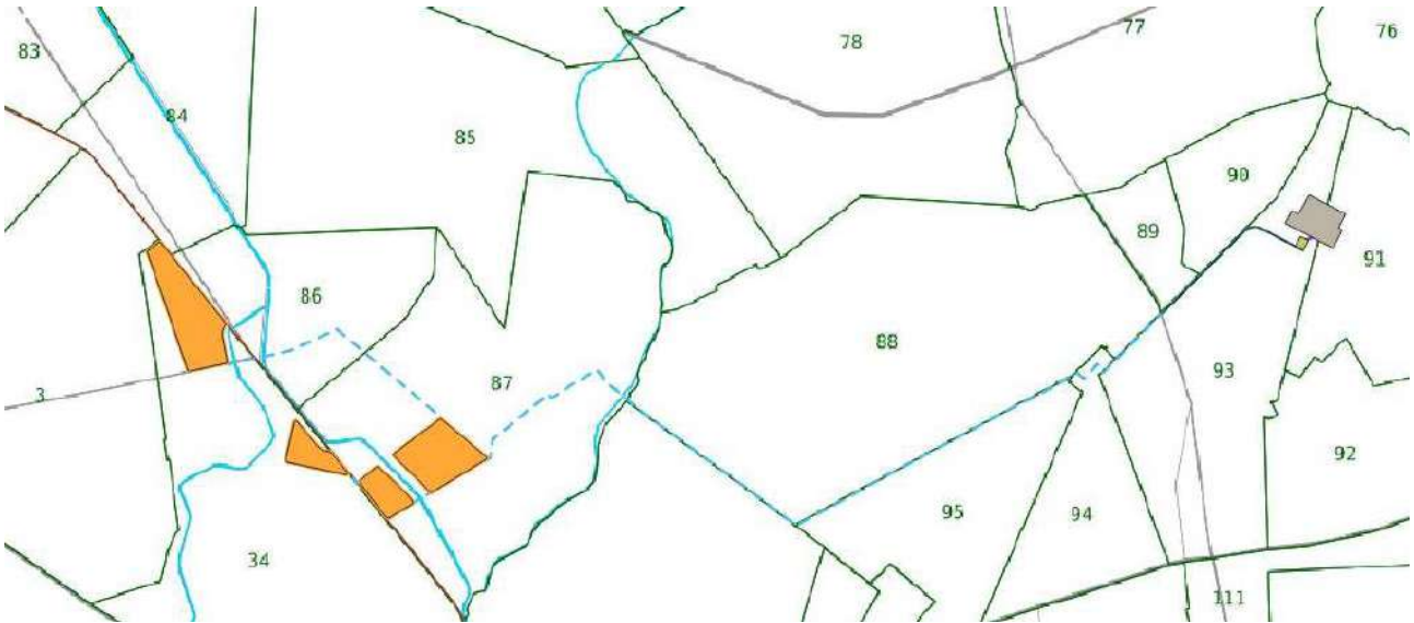
Figura 2: Inquadramento area di installazione impianto agrivoltaico
