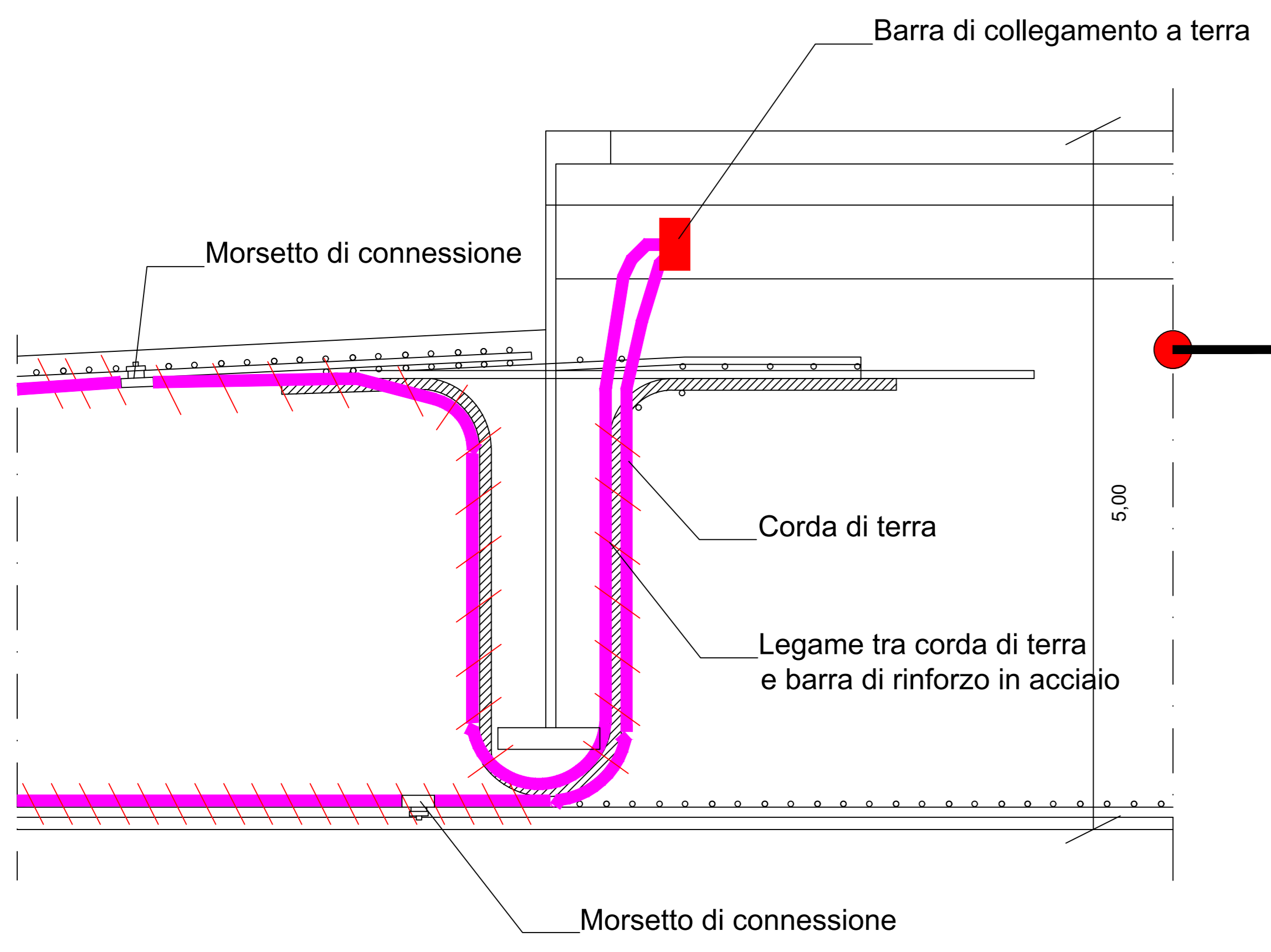
Dettaglio 1_Scala 1:30
