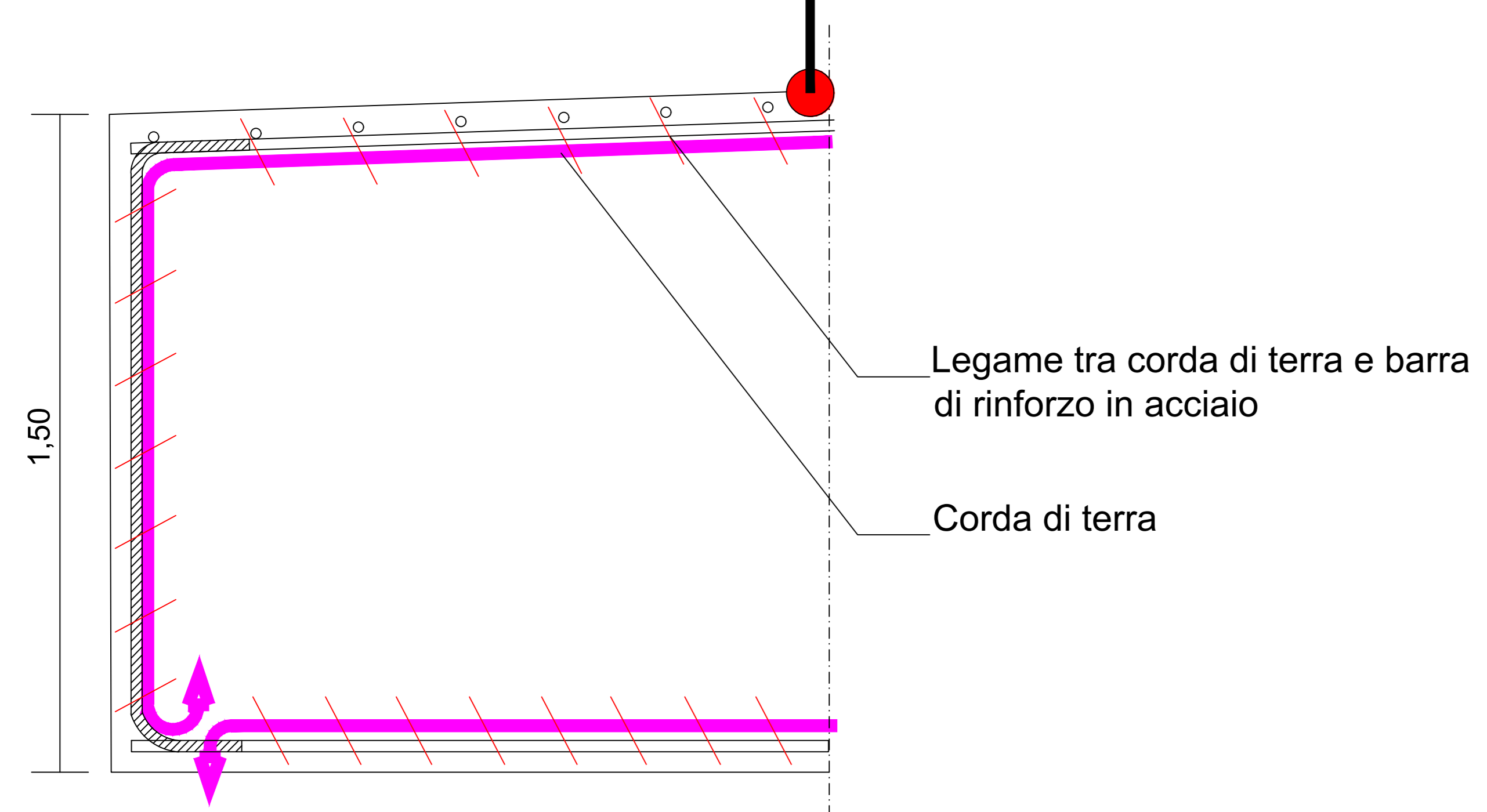
Dettaglio 2_Scala 1:10
