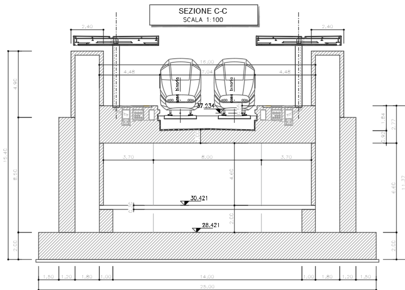
Figura 2.2 Sezione tipo nella parte centrale scale-ascensori
