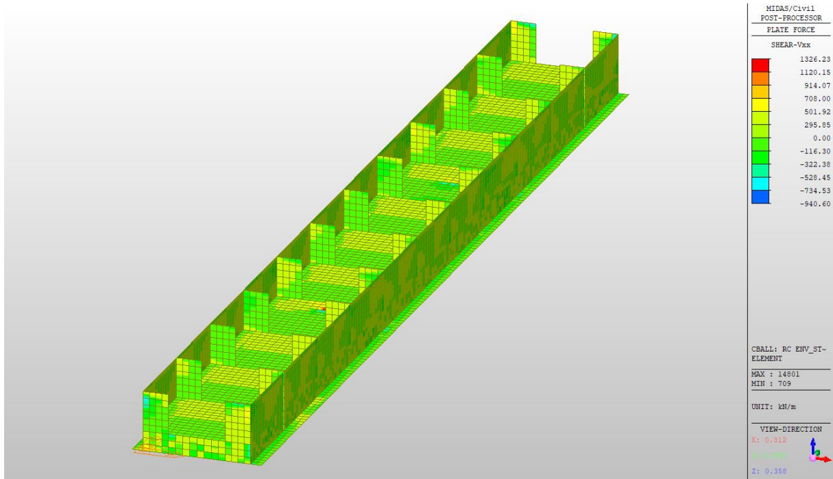
Figura 10.12: Involuppo SLU-SLV Vxx in evidenza piedritti interni, pareti e soletta inferiore
