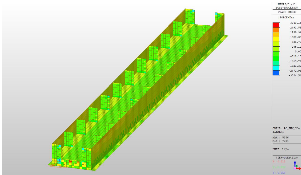
Figura 10.21: Involuppo SLE-Rara Fxx in evidenza piedritti interni, pareti e soletta inferiore
