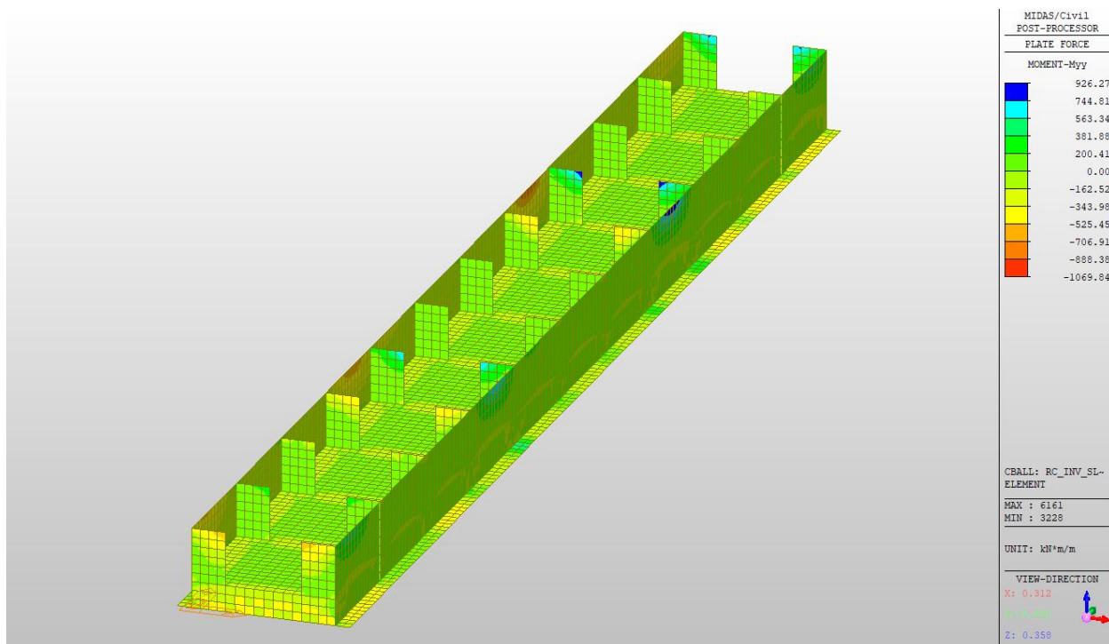
Figura 10.20: Involuppo SLE-Rara Myy in evidenza piedritti interni, pareti e soletta inferiore
