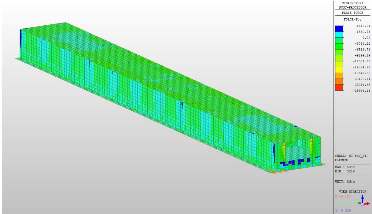
Figura 10.5: Involuppo SLU-SLV Fyy per tutta la struttura
