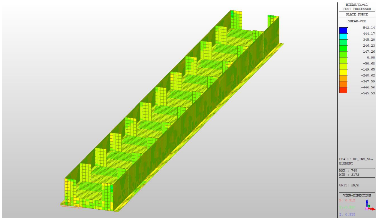
Figura 10.35: Involuppo SLE-QuasiPermanente Vxx in evidenza piedritti interni, pareti e soletta inferiore
