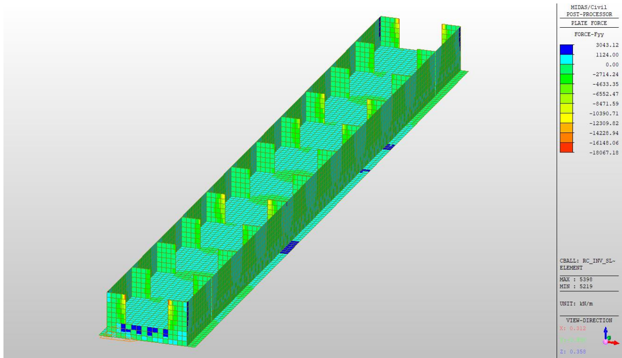
Figura 10.22: Involuppo SLE-Rara Fyy in evidenza piedritti interni, pareti e soletta inferiore
