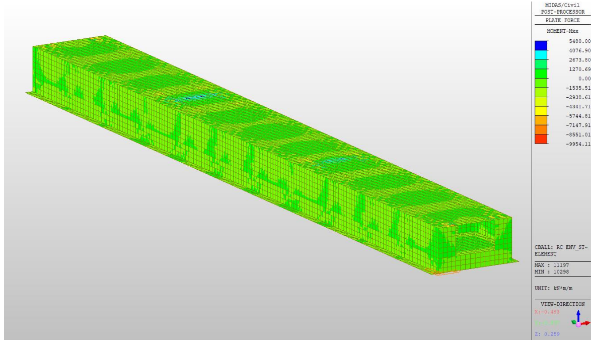
Figura 10.2: Involuppo SLU-SLV Mxx per tutta la struttura
