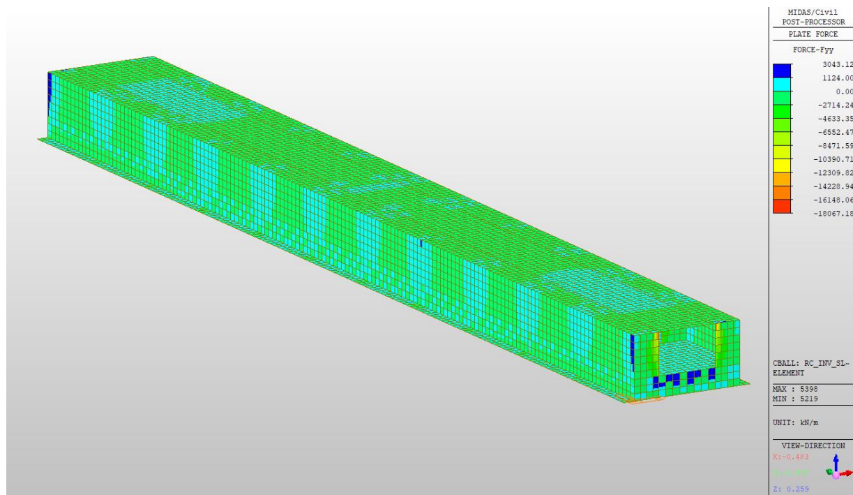
Figura 10.17: Involuppo SLE-Rara Fyy per tutta la struttura
