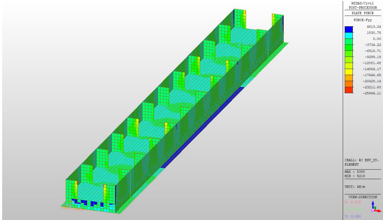
Figura 10.11: Involuppo SLU-SLV Fyy in evidenza piedritti interni, pareti e soletta inferiore
