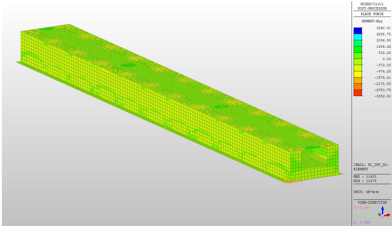
Figura 10.26: Involuppo SLE-QuasiPermanente Myy per tutta la struttura
