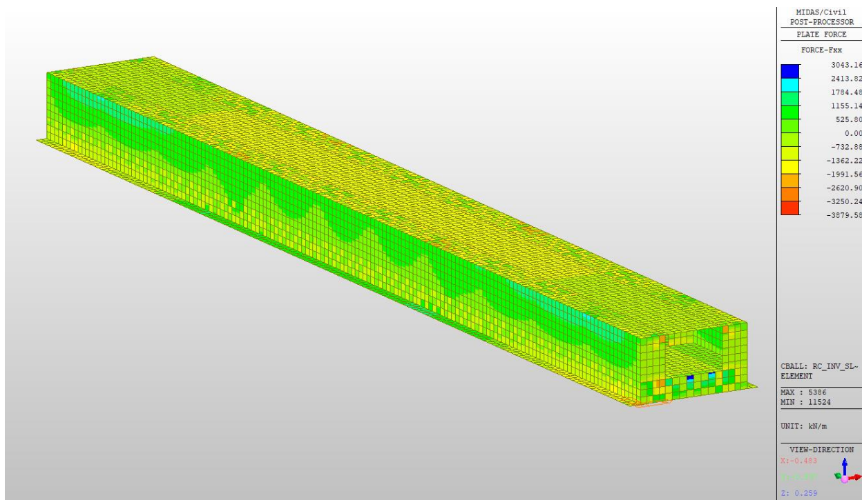
Figura 10.16: Involuppo SLE-Rara Fxx per tutta la struttura
