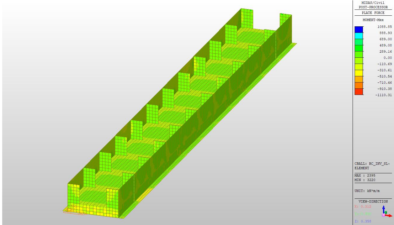
Figura 10.19: Involuppo SLE-Rara Mxx in evidenza piedritti interni, pareti e soletta inferiore
