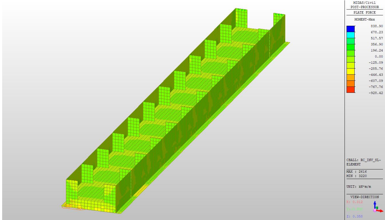
Figura 10.31: Involuppo SLE-QuasiPermanente Mxx in evidenza piedritti interni, pareti e soletta inferiore
