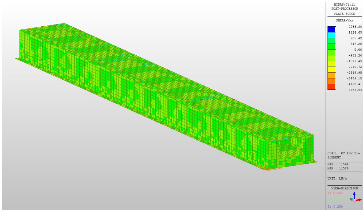
Figura 10.29: Involuppo SLE-QuasiPermanente Vxx per tutta la struttura
