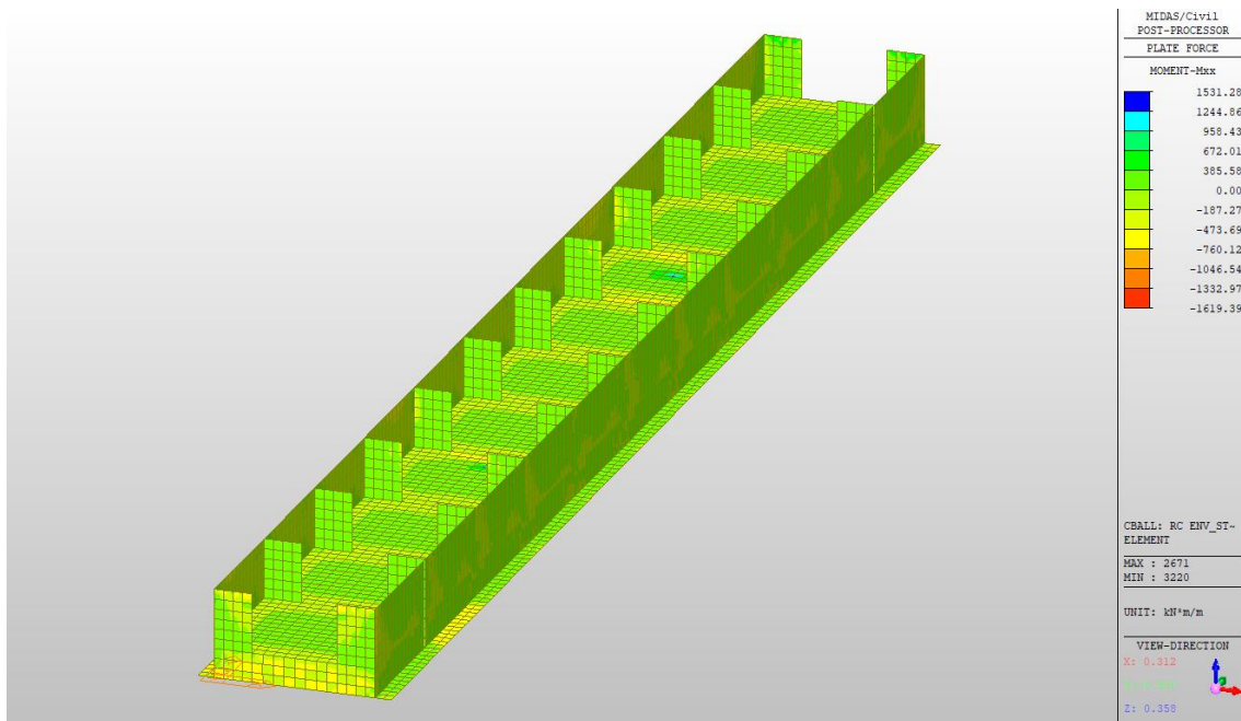
Figura 10.8: Inviluppo SLU-SLV Mxx in evidenza piedritti interni, pareti e soletta inferiore
