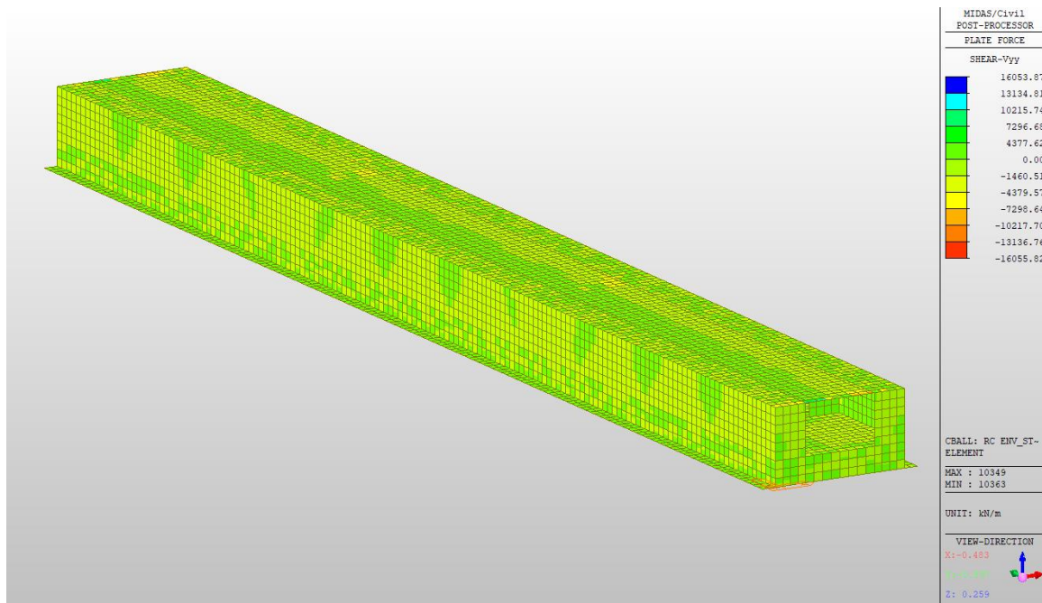
Figura 10.7: Involuppo SLU-SLV Vyy per tutta la struttura
