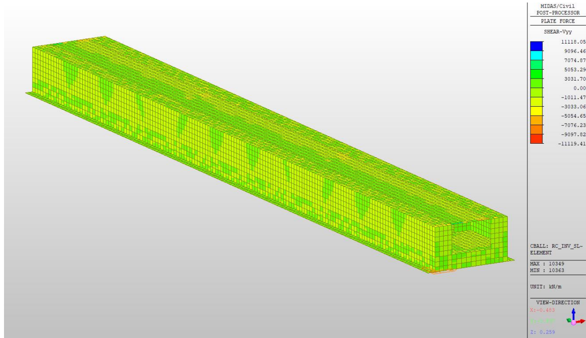
Figura 10.18: Involuppo SLE-Rara Vyy per tutta la struttura
