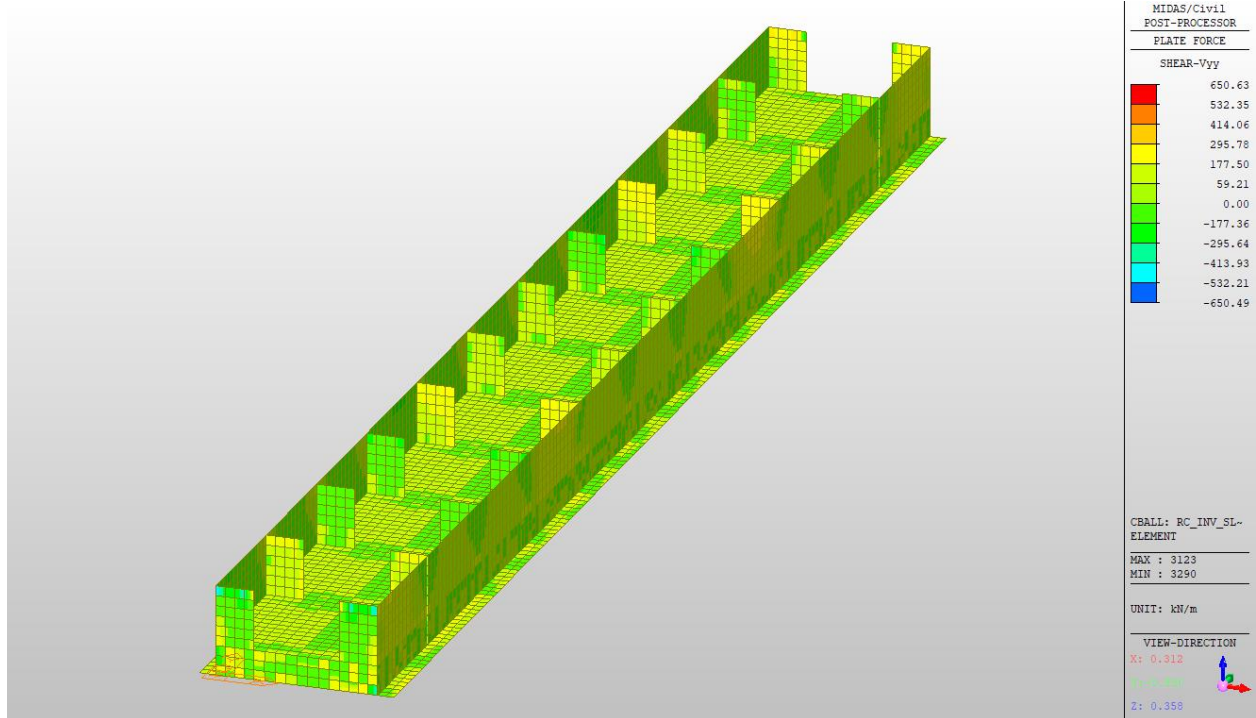
Figura 10.24: Involuppo SLE-Rara Vyy in evidenza piedritti interni, pareti e soletta inferiore
