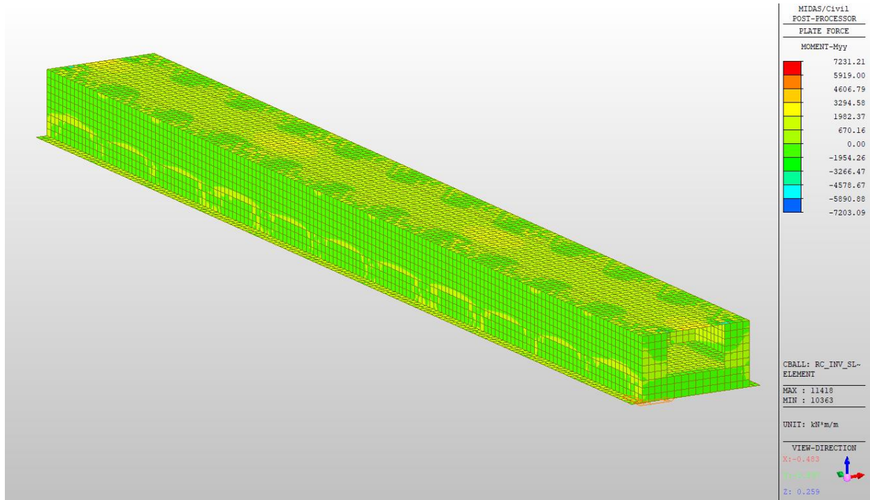
Figura 10.15: Involuppo SLE-Rara Myy per tutta la struttura
