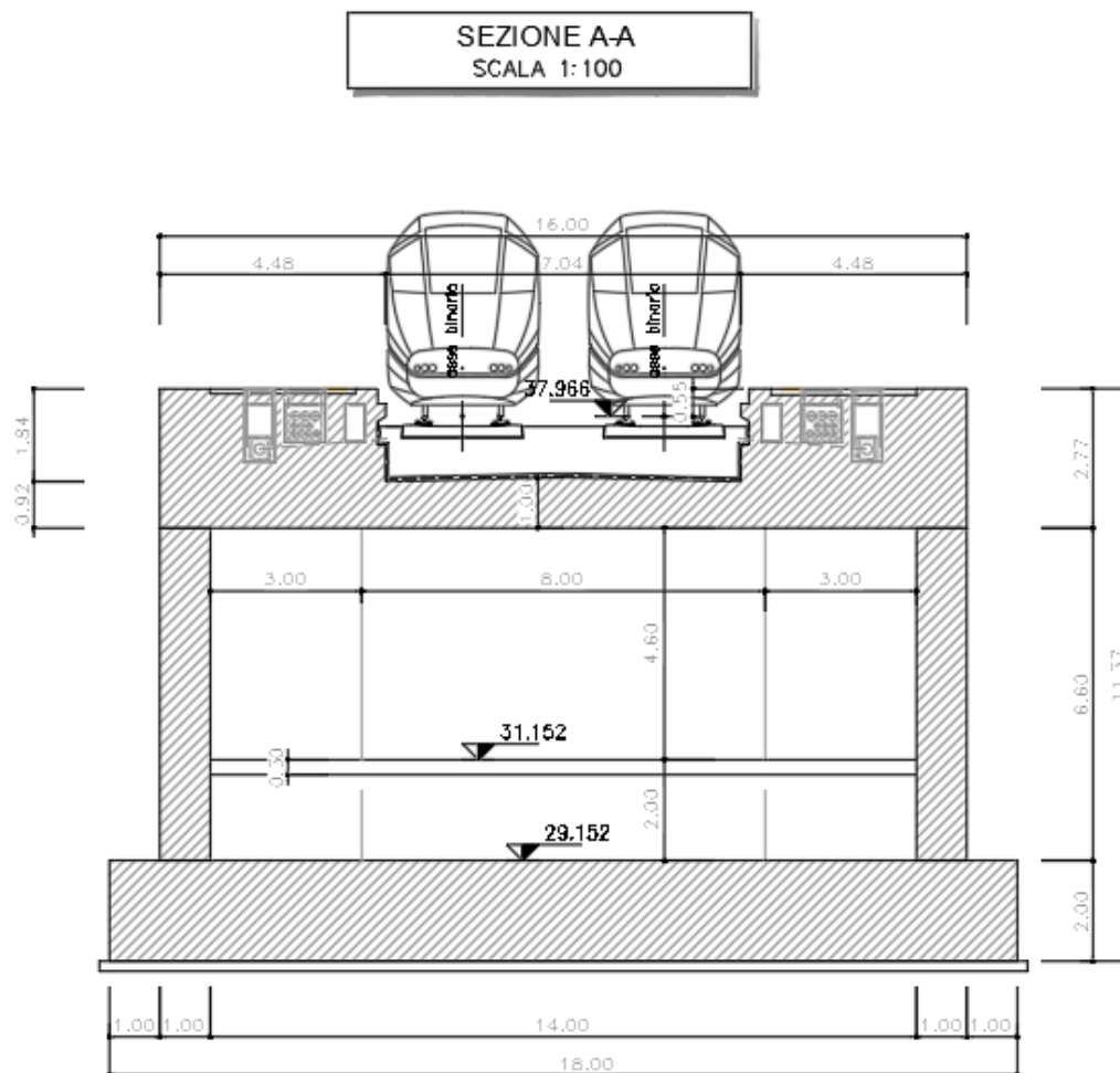
Figura 2.1 Sezione tipo nella parte iniziale e finale
