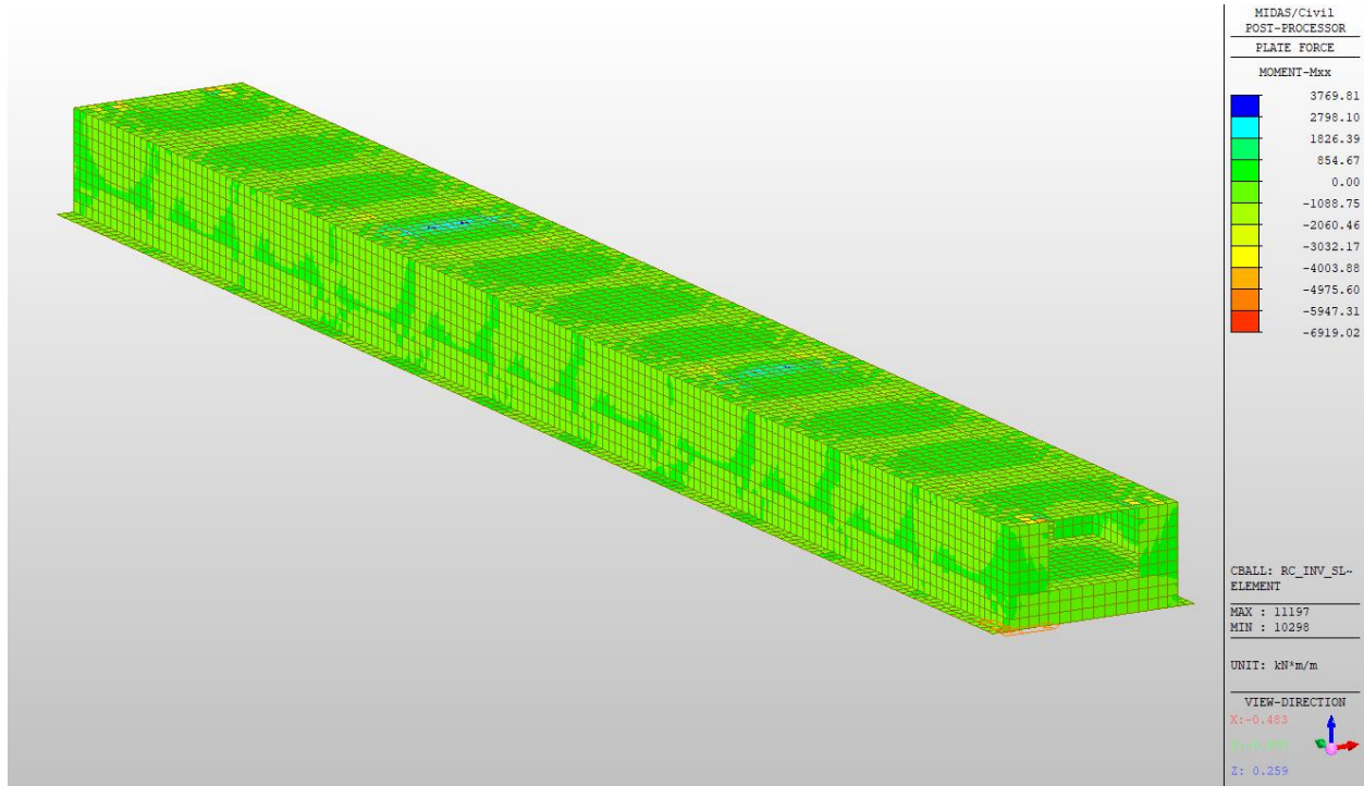
Figura 10.14: Involuppo SLE-Rara Mxx per tutta la struttura
