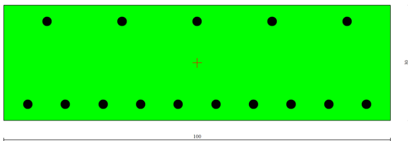
Figura 11.6: Geometria sezione e armatura solaio intermedio
