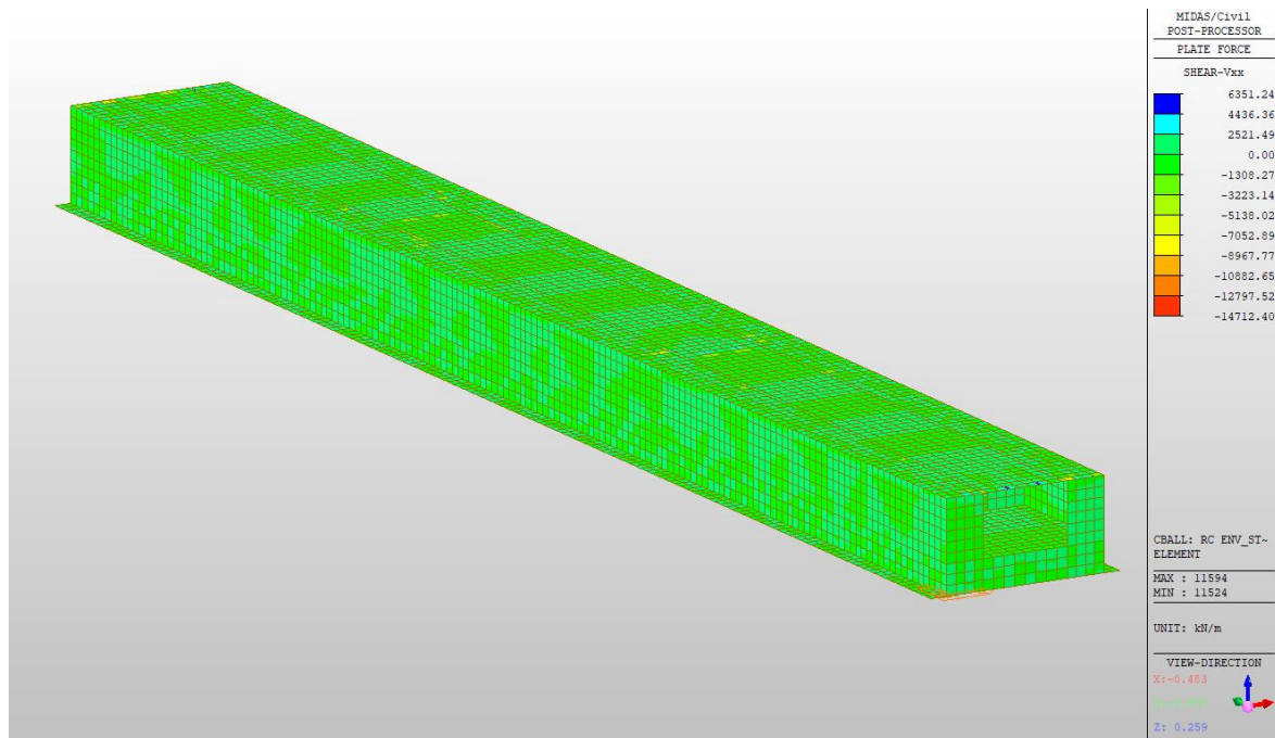
Figura 10.6: Involuppo SLU-SLV Vxx per tutta la struttura
