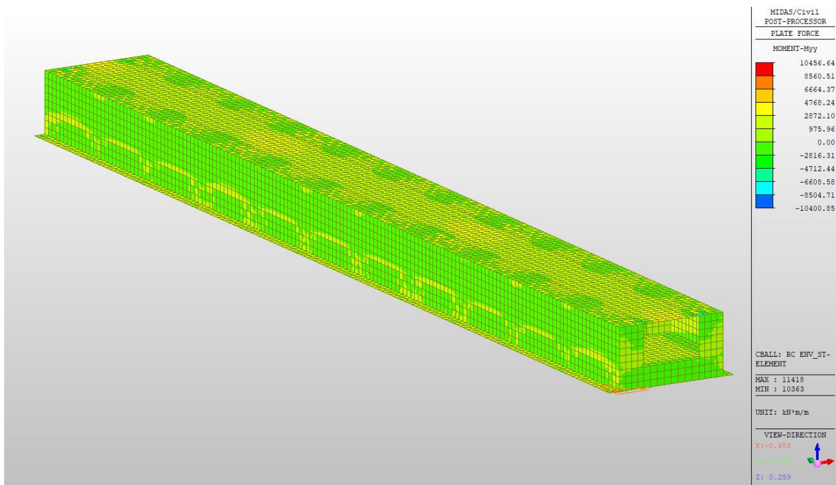
Figura 10.9: Inviluppo SLU-SLV Myy in evidenza piedritti interni, pareti e soletta inferiore
