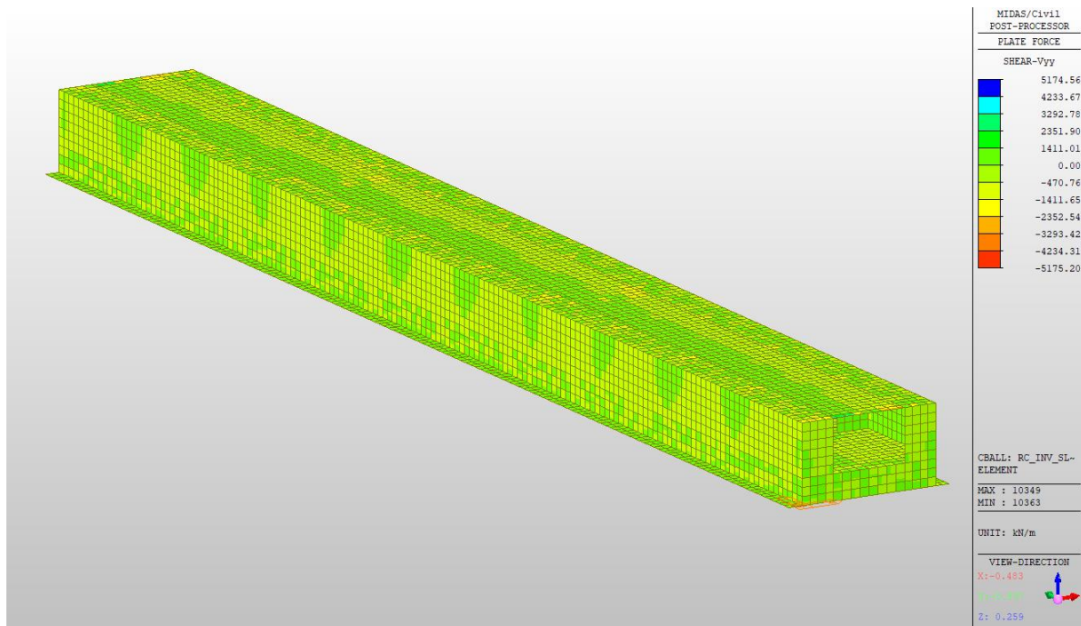
Figura 10.30: Involuppo SLE-QuasiPermanente Vyy per tutta la struttura
