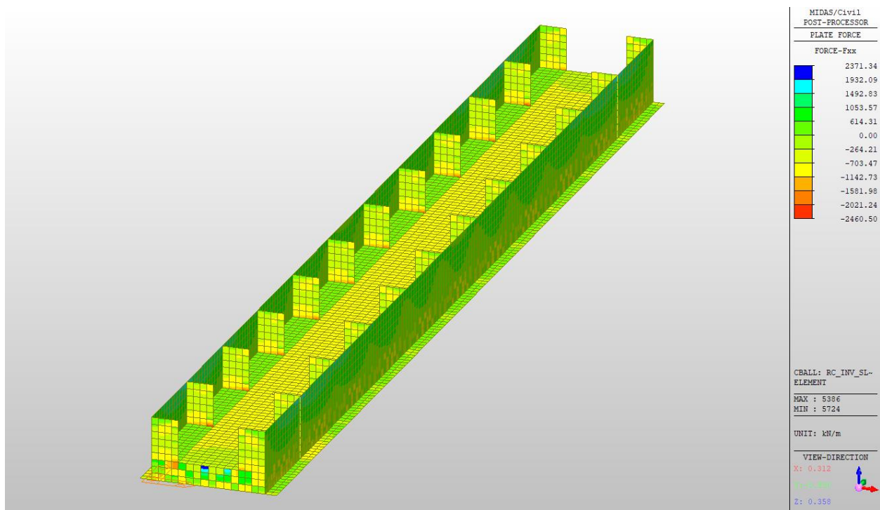
Figura 10.33: Involuppo SLE-QuasiPermanente Fxx in evidenza piedritti interni, pareti e soletta inferiore
