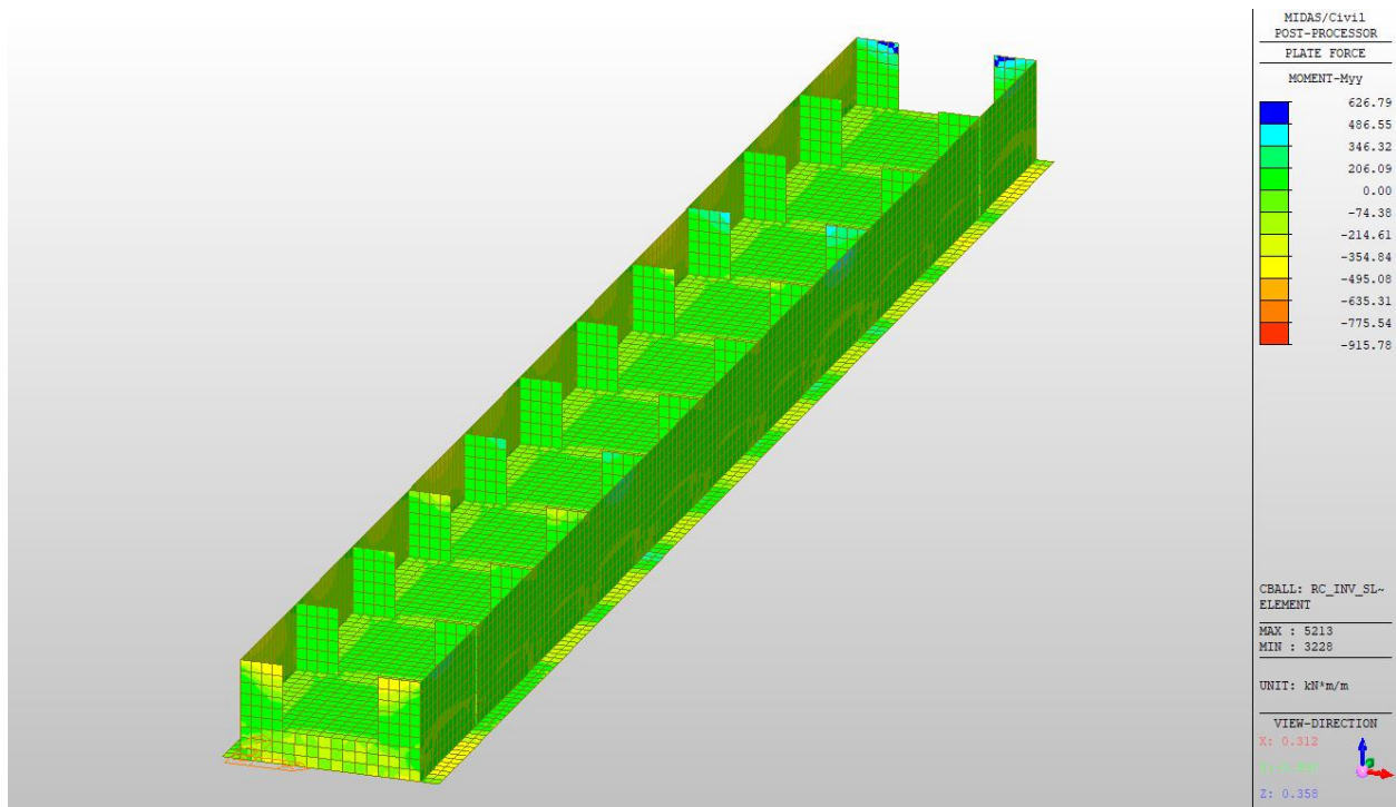
Figura 10.32: Involuppo SLE-QuasiPermanente Myy in evidenza piedritti interni, pareti e soletta inferiore
