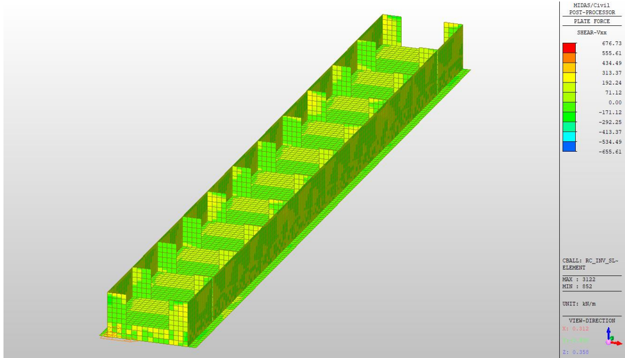
Figura 10.23: Involuppo SLE-Rara Vxx in evidenza piedritti interni, pareti e soletta inferiore
