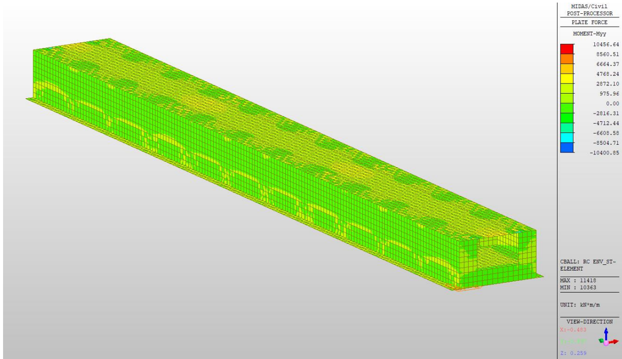
Figura 10.3: Involuppo SLU-SLV Myy per tutta la struttura
