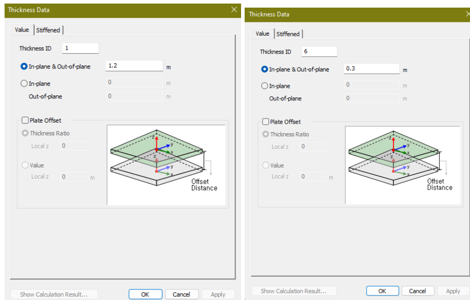
Figura 7.2 Elementi bidimensionali
