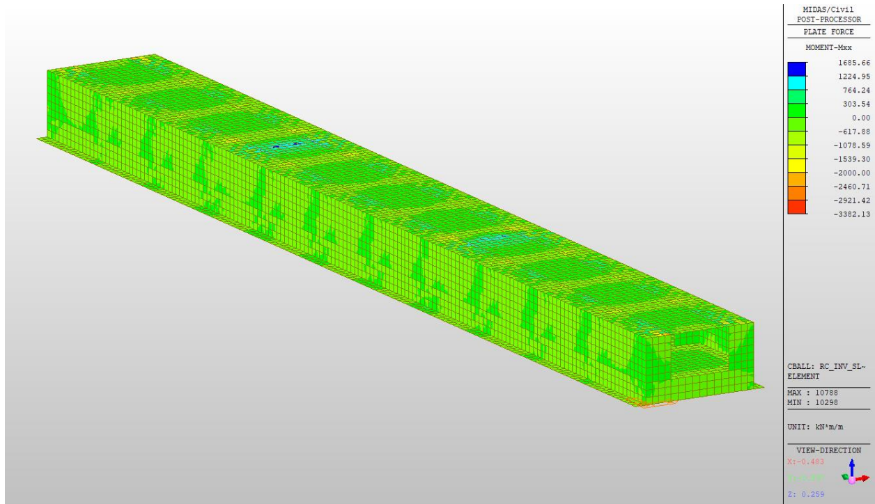
Figura 10.25: Involuppo SLE-QuasiPermanente Mxx per tutta la struttura
