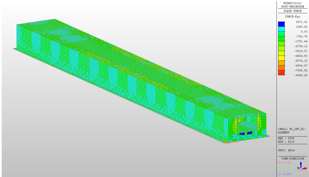
Figura 10.28: Involuppo SLE-QuasiPermanente Fyy per tutta la struttura
