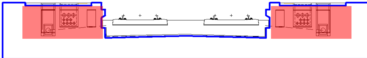
Figura 8.2 Sezione non resistente della soletta superiore
