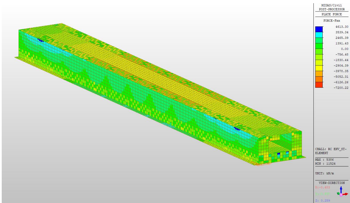
Figura 10.4: Involuppo SLU-SLV Fxx per tutta la struttura
