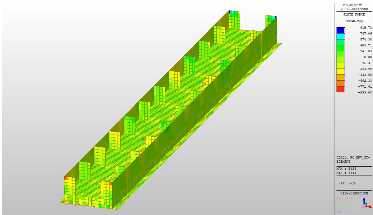
Figura 10.13: Involuppo SLU-SLV Vyy in evidenza piedritti interni, pareti e soletta inferiore
