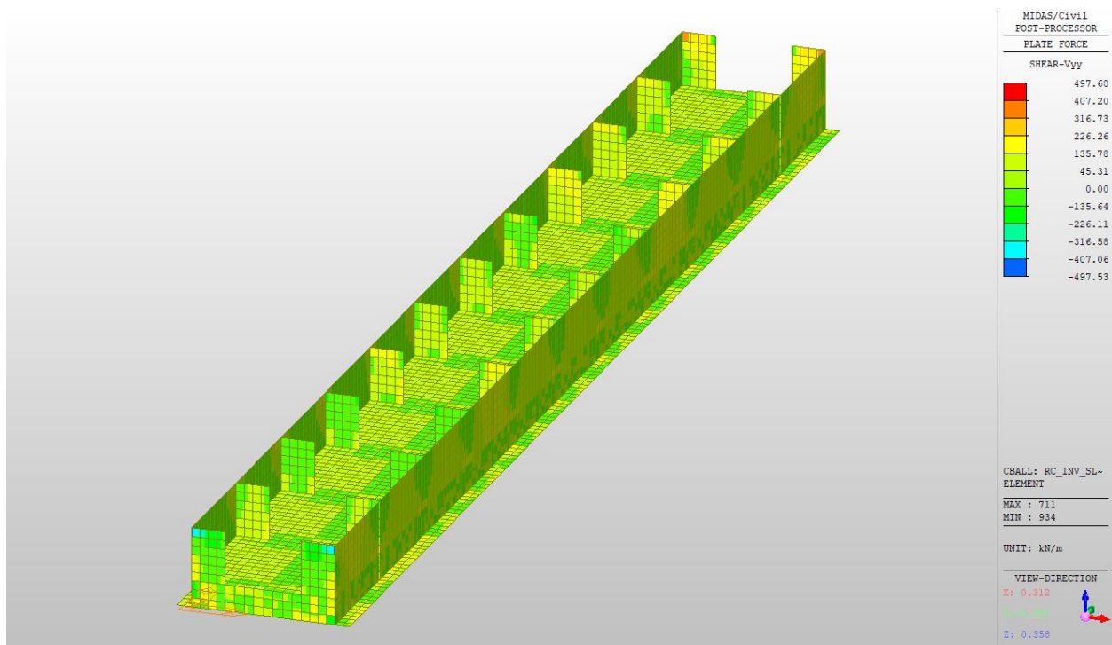
Figura 10.36: Involuppo SLE-QuasiPermanente Vyy in evidenza piedritti interni, pareti e soletta inferiore
