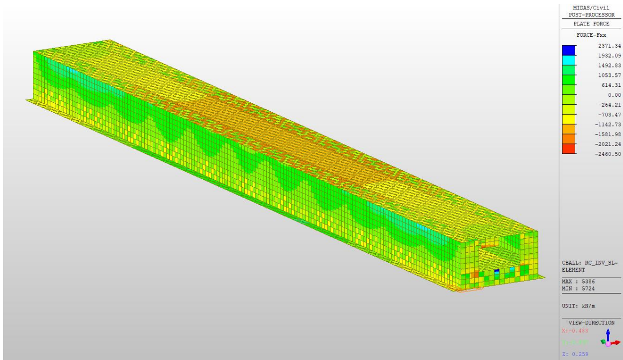
Figura 10.27: Involuppo SLE-QuasiPermanente Fxx per tutta la struttura
