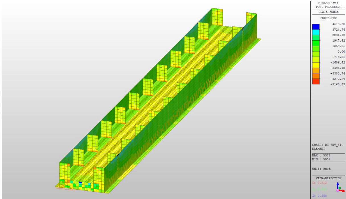
Figura 10.10: Inviluppo SLU-SLV Fxx in evidenza piedritti interni, pareti e soletta inferiore
