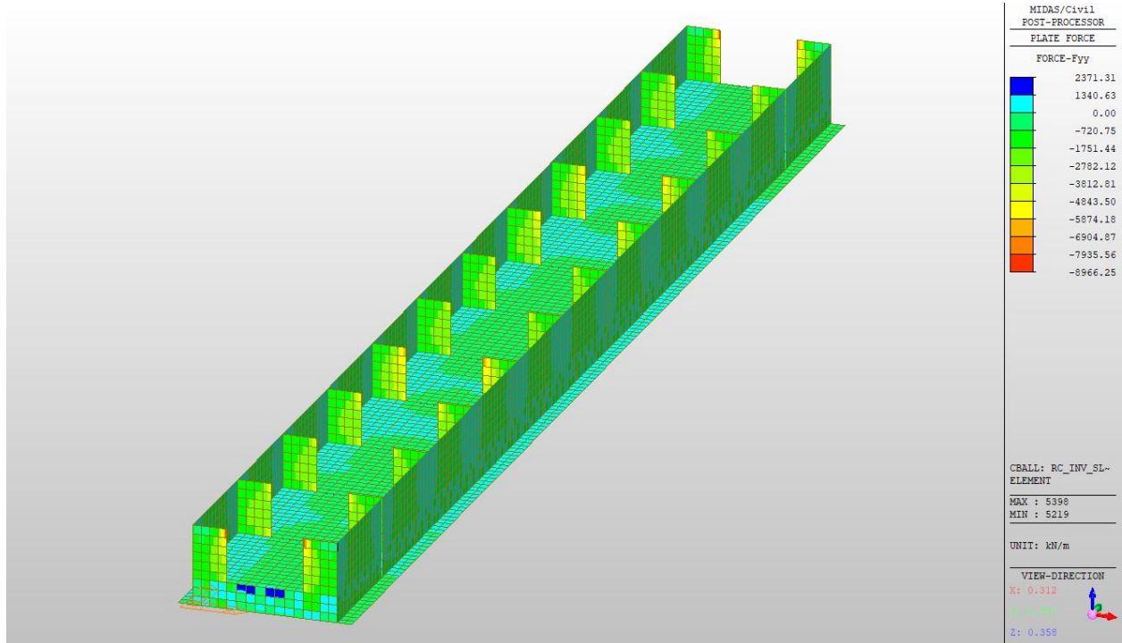
Figura 10.34: Involuppo SLE-QuasiPermanente Fyy in evidenza piedritti interni, pareti e soletta inferiore
