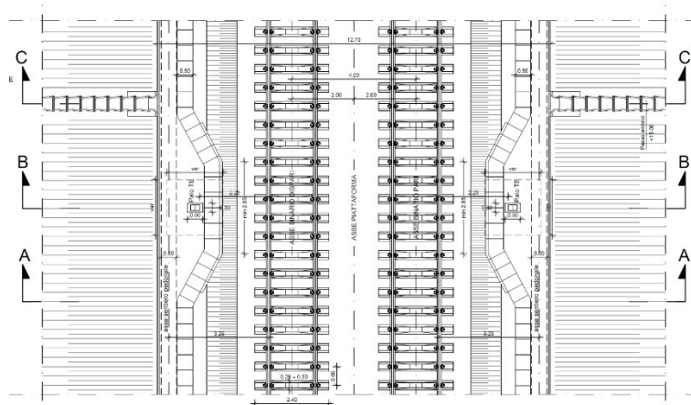
Figura 20 - Stralcio planimetrico con sezione tipo ferroviaria in rilevato a doppio binario in rettilo
