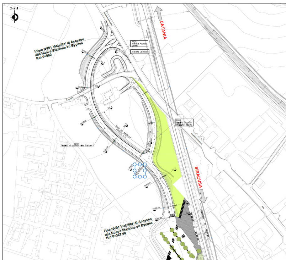
Figura 34 – NV01, viabilità si accesso alla stazione
