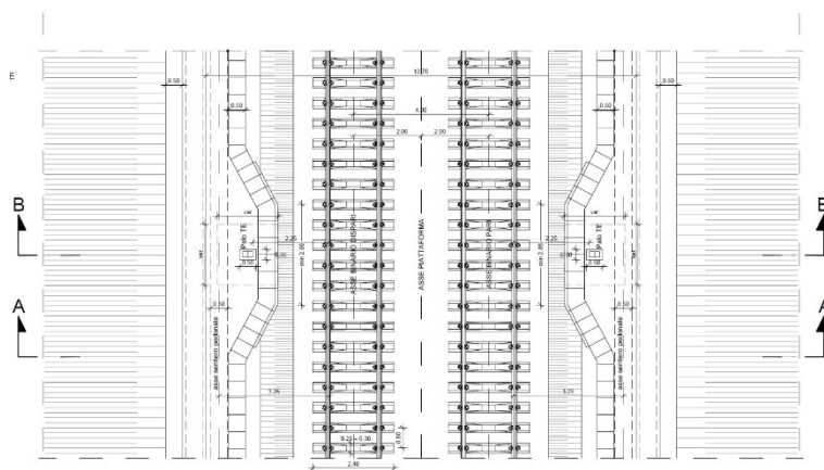
Figura 26 - Stralcio planimetrico con sezione tipo ferroviaria in trincea a doppio binario in rettilineo
