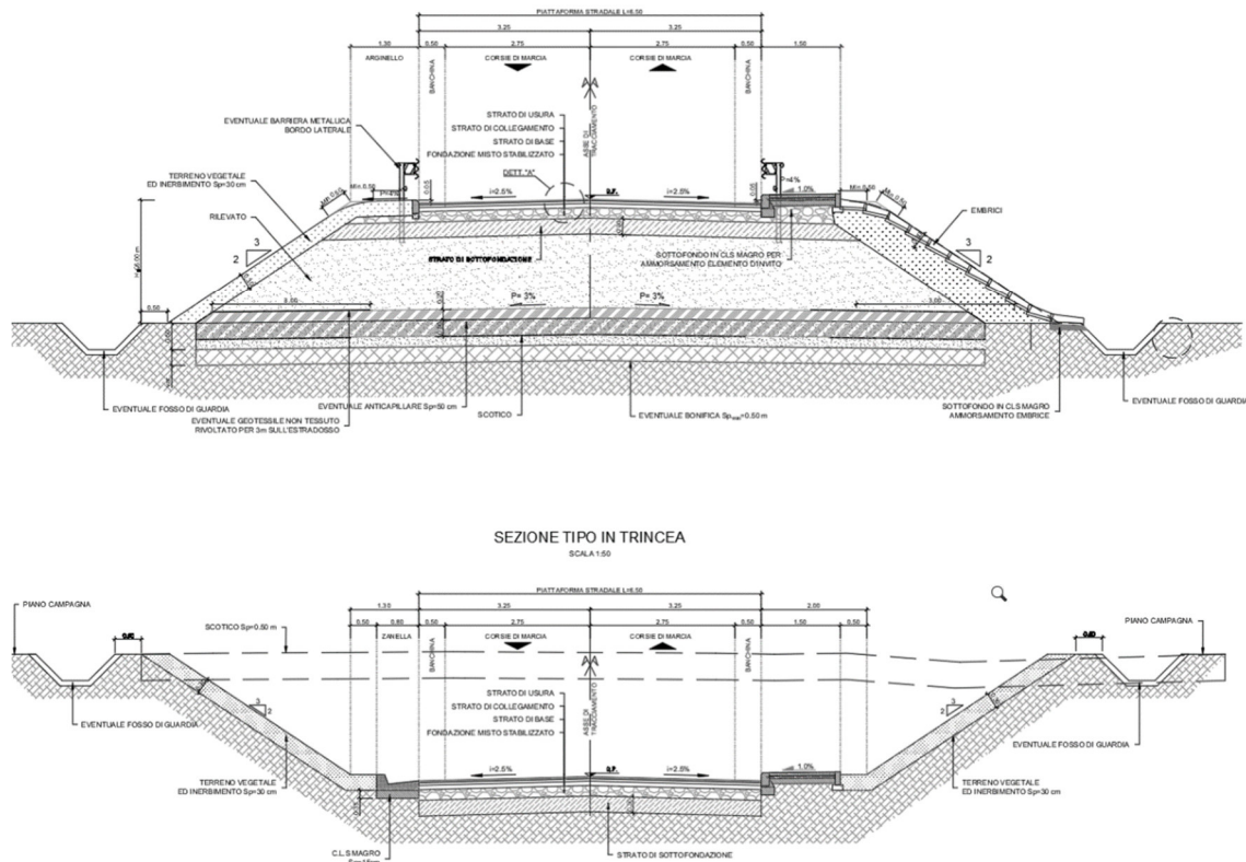
Figura 29 - Sezione tipo NV03
