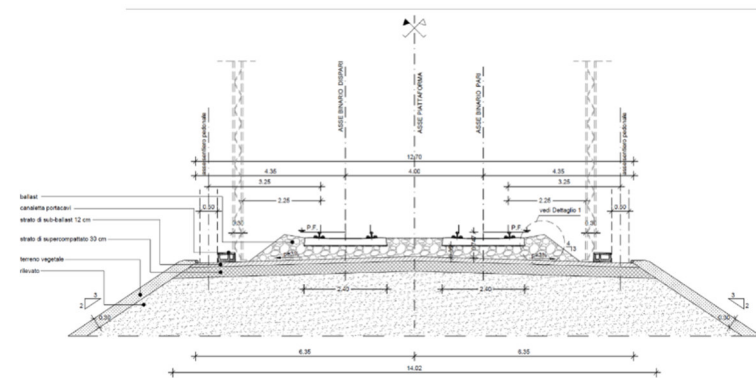
Figura 19 - Sezione tipo ferroviaria in rilevato a doppio binario in rettilo
