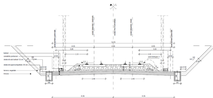
Figura 25 - Sezione tipo ferroviaria in trincea a doppio binario in rettifilo
