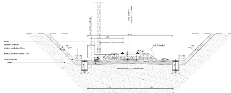
Figura 23 - Sezione tipo ferroviaria in trincea a singolo binario in rettifilo
