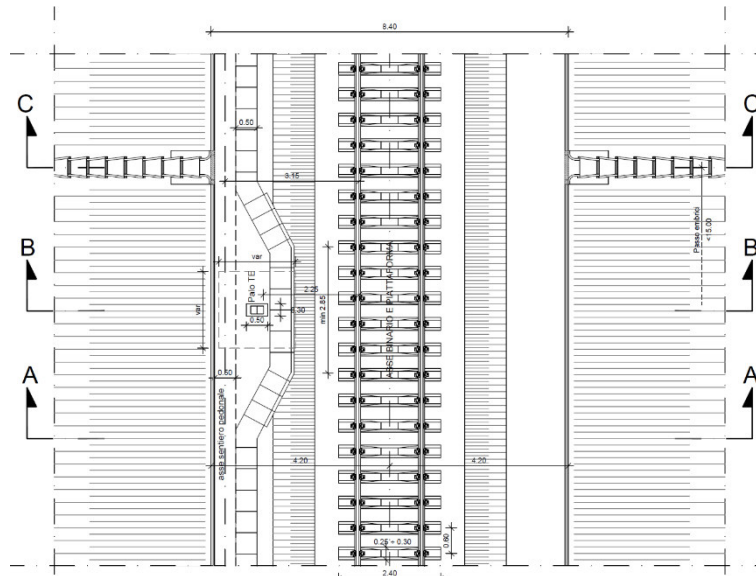
Figura 18 - Stralcio planimetrico con sezione tipo ferroviaria in rilevato a singolo binario in rettilo
