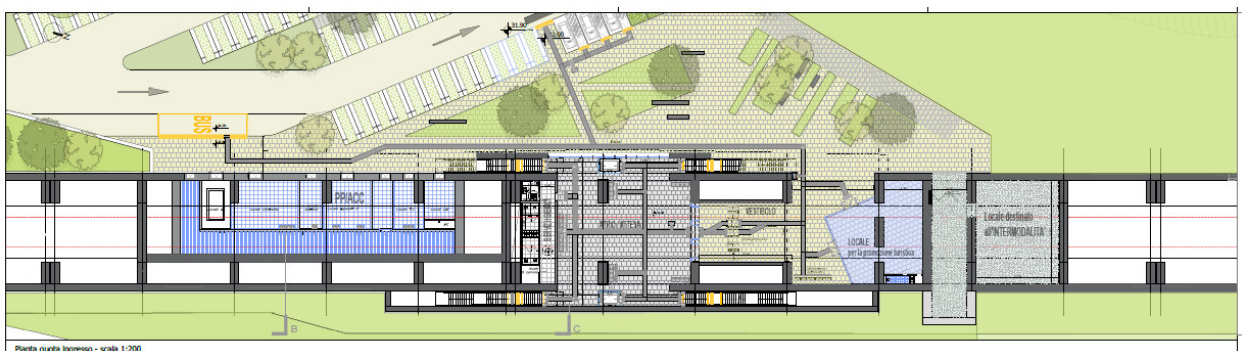
Figura 32 - Layout Stazione quota ingresso (Interno opera scatolare)
