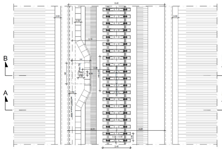
Figura 24 - Stralcio planimetrico con sezione tipo ferroviaria in trincea a singolo binario in rettifilo
