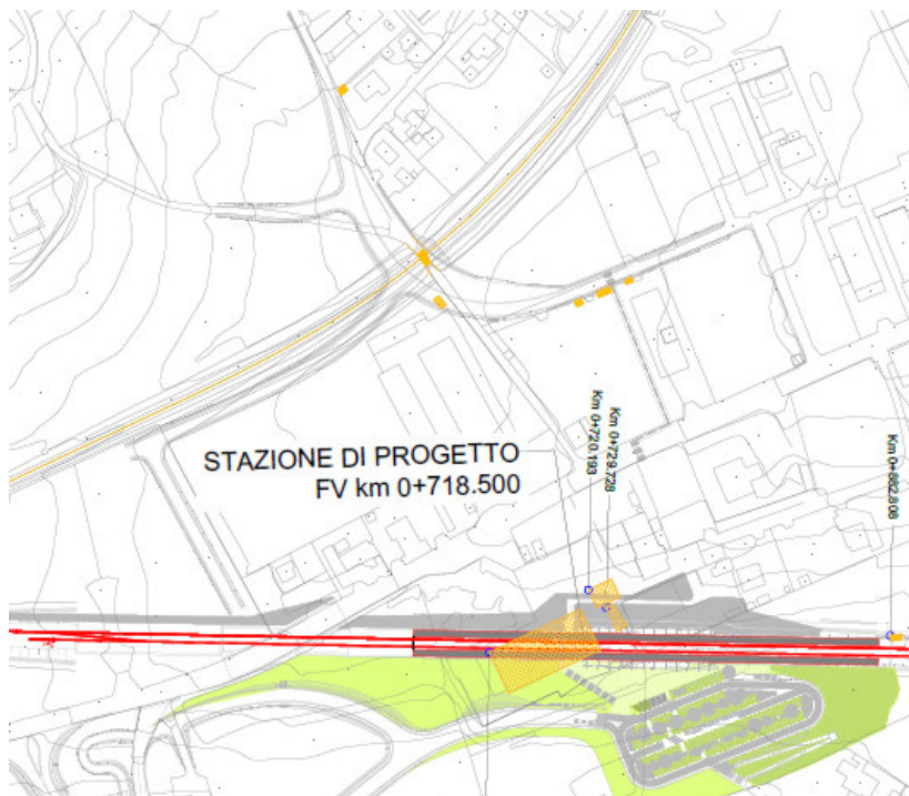
Figura 16 - Configurazione di Progetto
