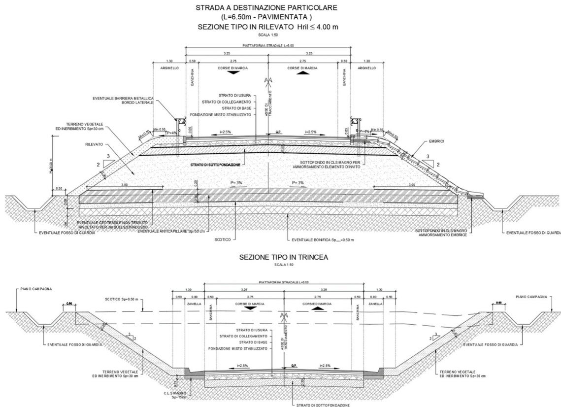
Figura 30 - Sezione tipo NV02 e NV05
