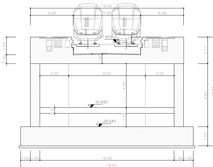
Figura 2-5 Scatolare di stazione – FV01: Sezione tipo
