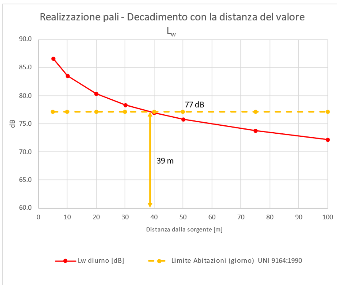
Figura 6-31 Realizzazione pali – decadimento con la distanza del valore L_w e confronto con i limiti previsti dalla normativa UNI 9614
