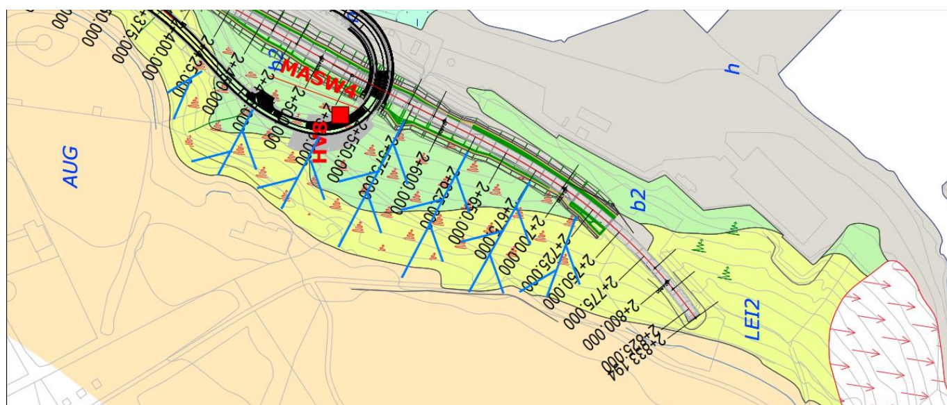
Figura 5-19 Ubicazione delle trincee drenanti previste per la stabilizzazione dei versanti soggetti a dissesti
