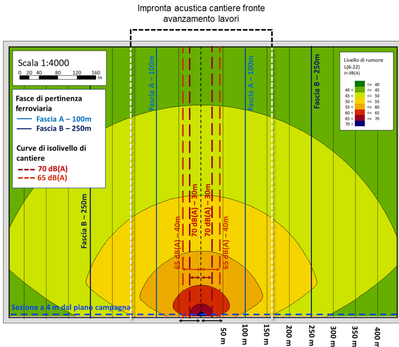
Figura 6-24 Scenario B: Confronto tra le distanze che intercorrono tra le curve di isolivello relative alle attività di cantiere ed i limiti previsti per le fasce di pertinenza acustica ferroviaria
