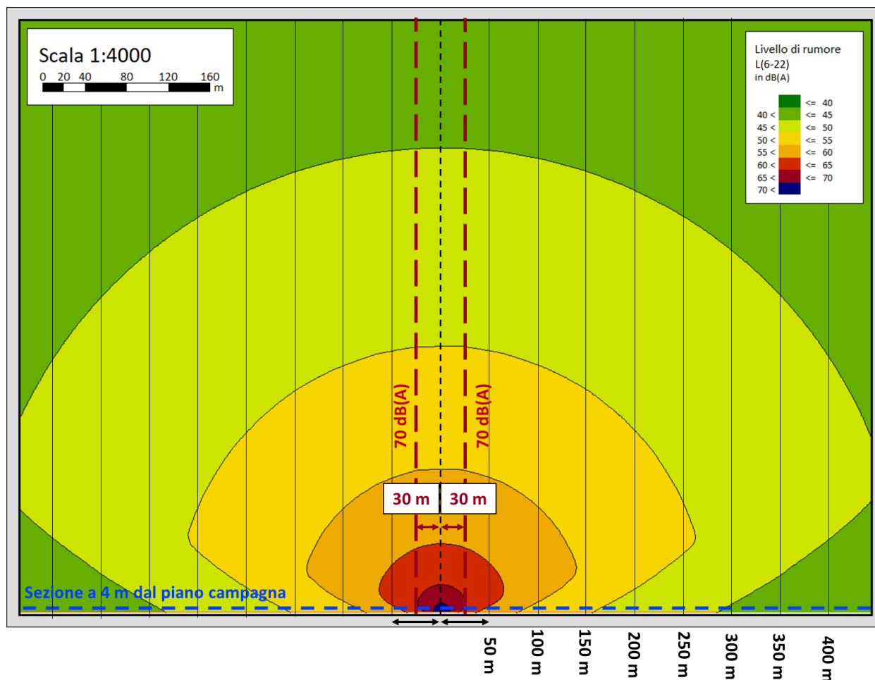
Figura 6-23 Scenario B: Stralcio dell’output del modello di simulazione in sezione verticale: curve di isolivello acustico in Leq(A) diurno
