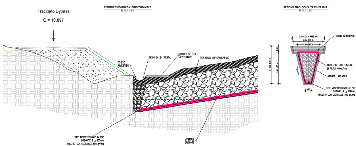
Figura 5-20 Sezioni delle trincee drenanti
