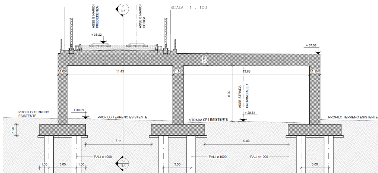
Figura 2-3 GA01: Sezione trasversale
