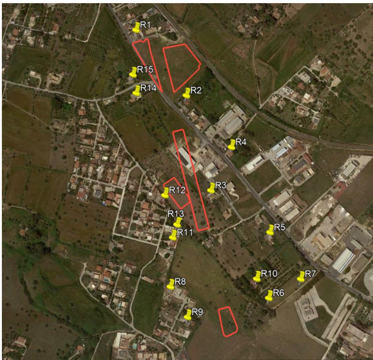
Figura 6-54 Scenario A: Schematizzazione aree di cantiere e relativi ricettori per lo scenario di simulazione
