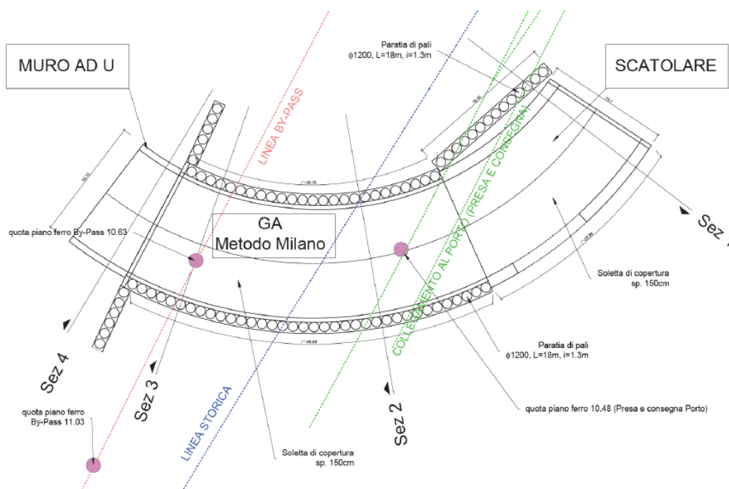
Figura 2-4 SL02: Pianta
