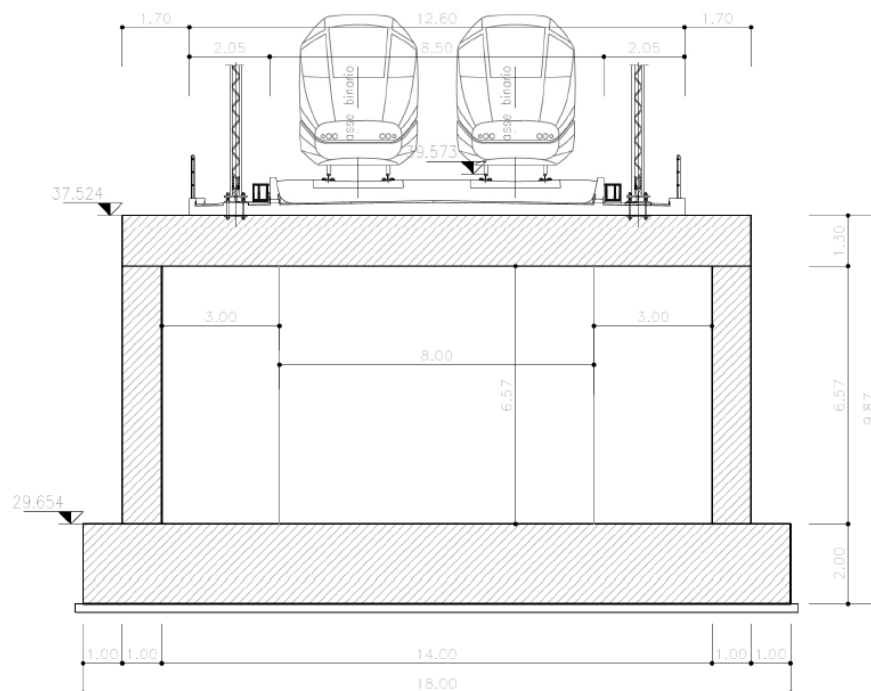
Figura 2-2 SL01: Sezione trasversale
