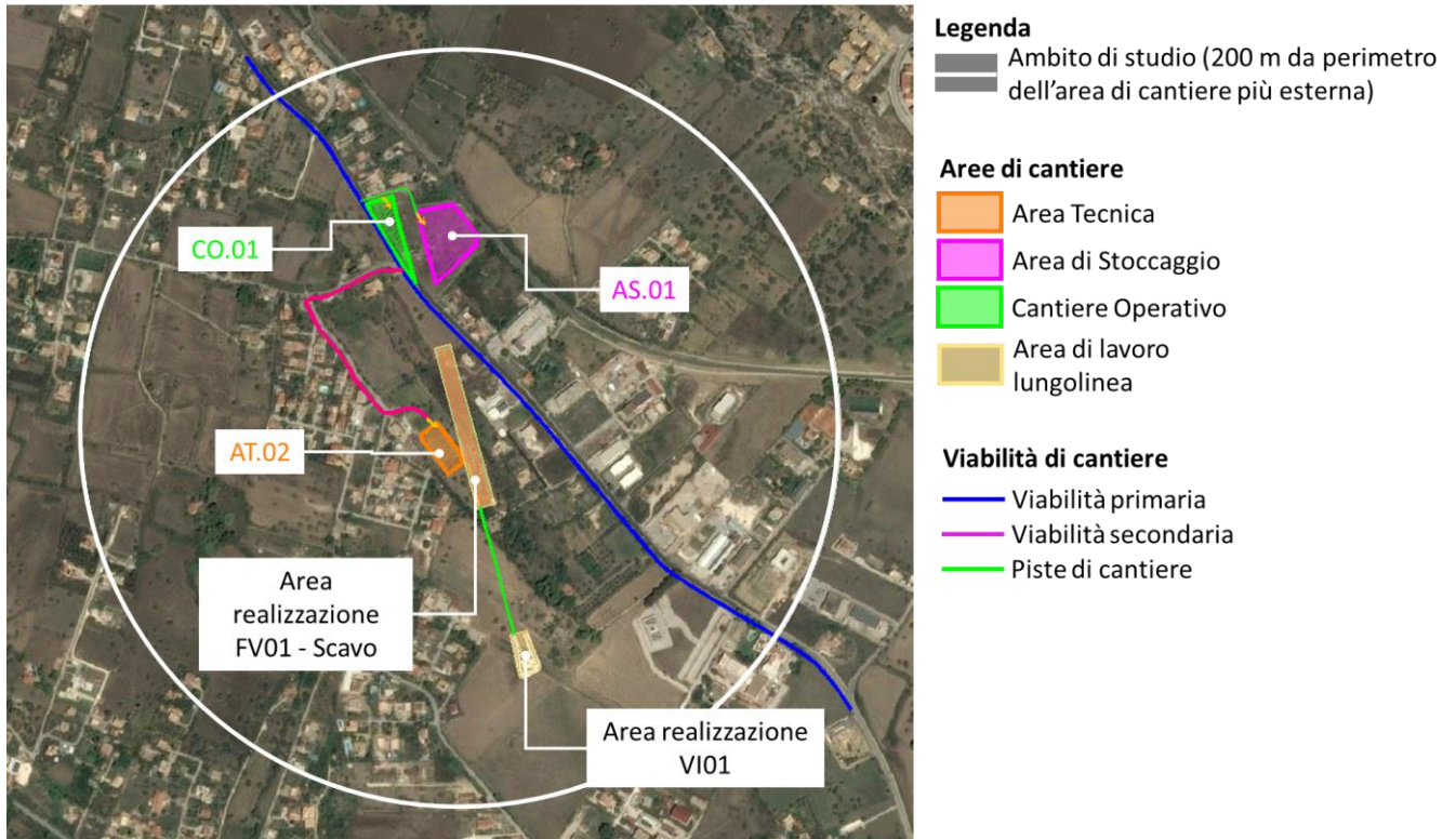
Figura 6-9 Scenario A - Localizzazione delle aree di cantiere, attività di lavorazione e flussi di traffico relativi allo scenario di simulazione
