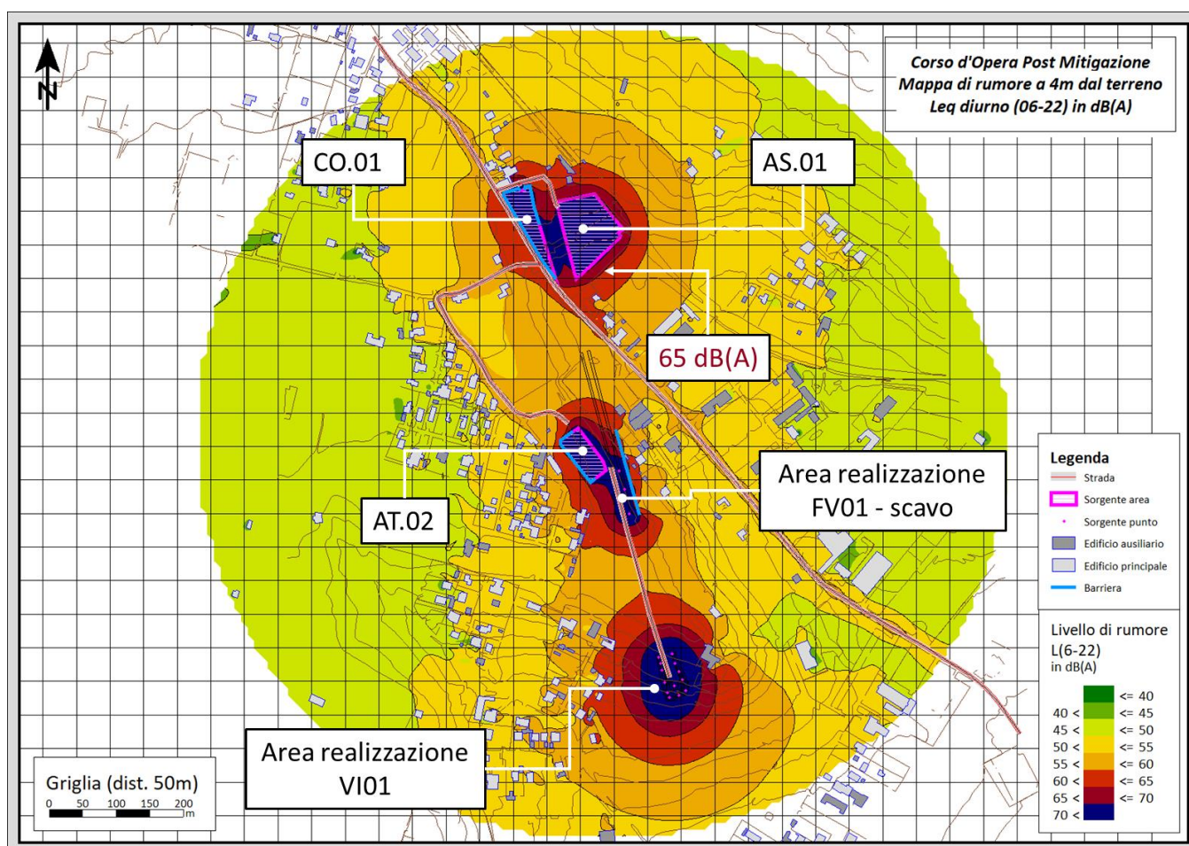
Figura 6-19 Scenario A: Output del modello di simulazione in planimetria con presenza di mitigazioni: curve di isolivello acustico in Leq(A) diurno
