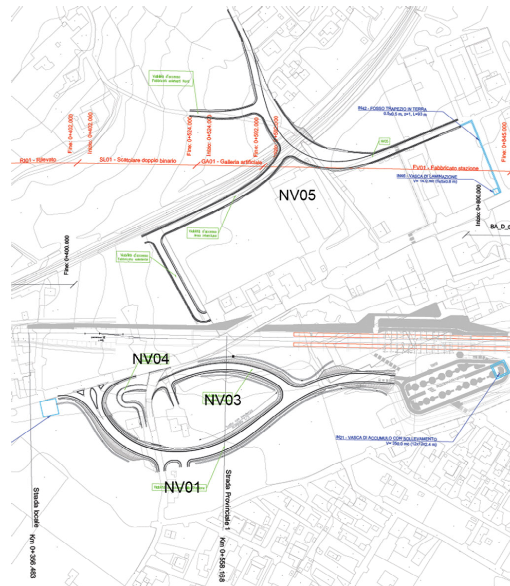
Figura 4-2 Inquadramento viabilità NV01, NV03, NV04 e NV05
