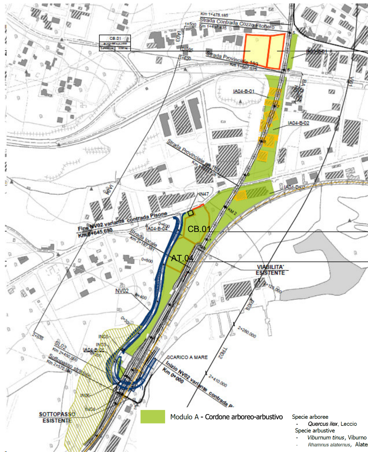
Figura 5-7 Planimetria delle opere a verde (RS6000R22P5IA0000001A)
