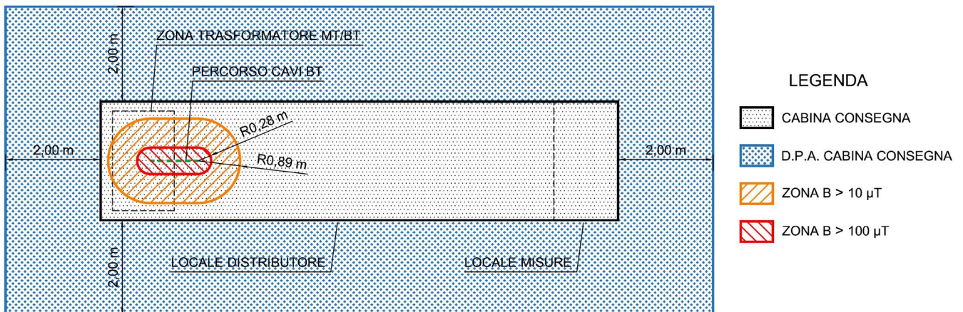
Figura 2 - Zone induzione magnetica cabina di consegna
