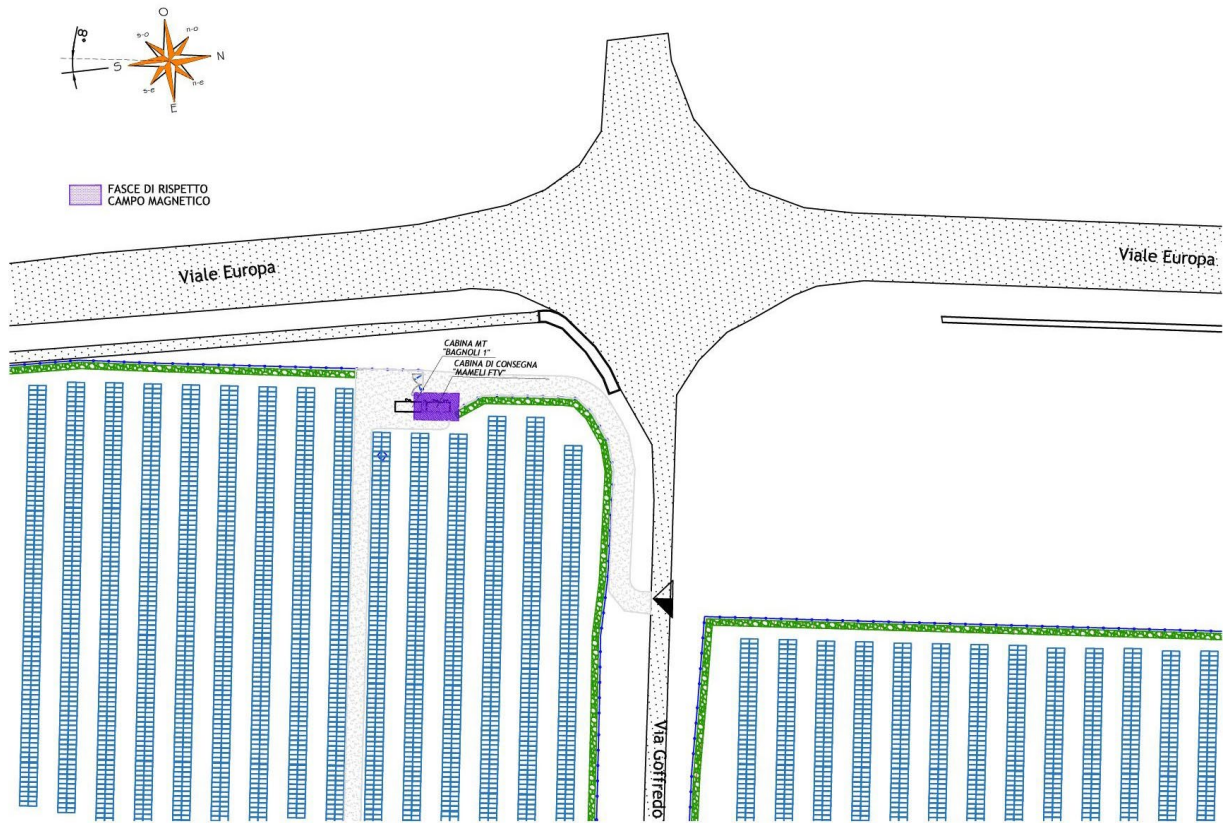
Figura 4 - Particolare cabina di consegna "MAMELI FTV"
