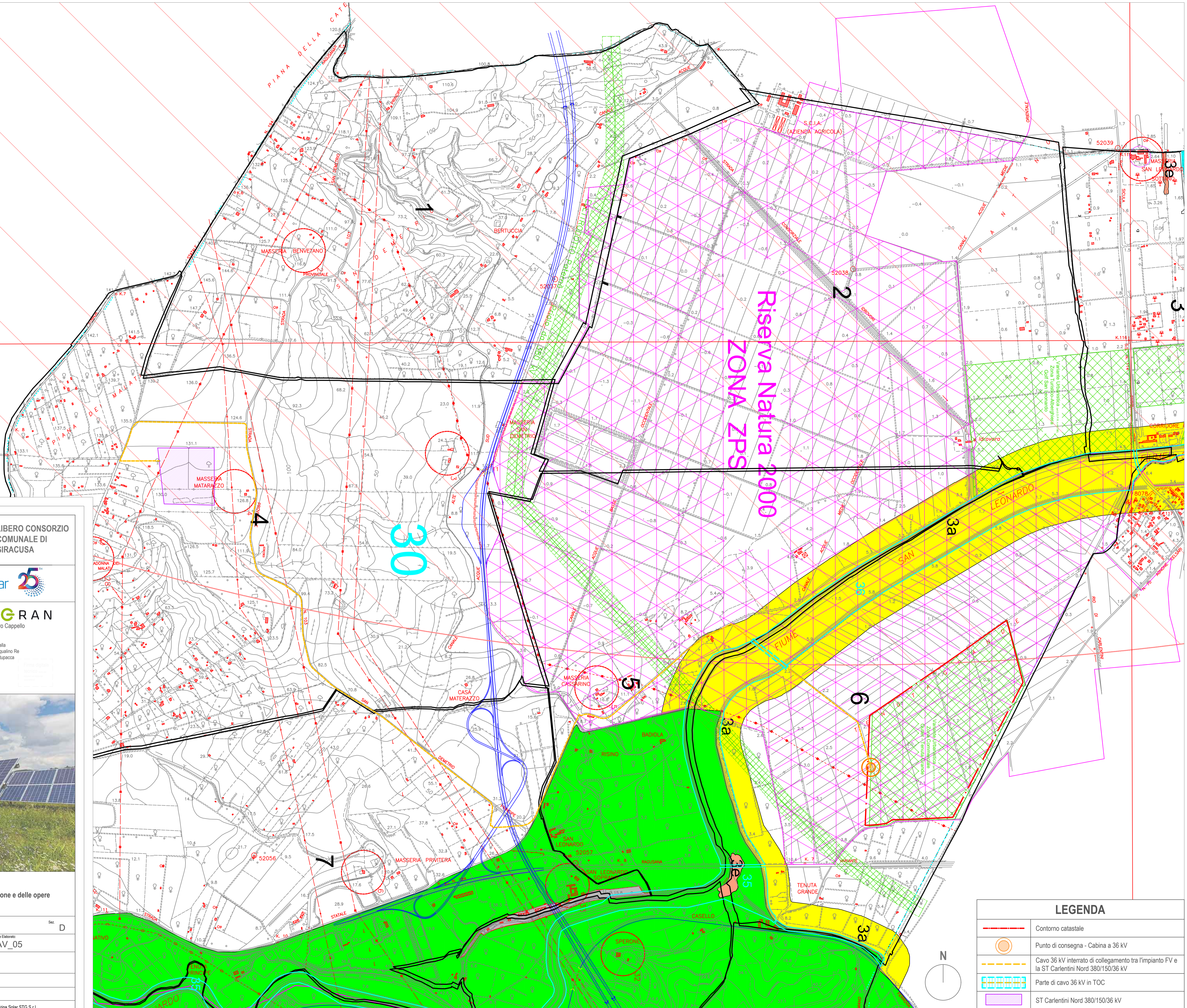
PLANIMETRIA IMPIANTO FOTOVOLTAICO SU P.R.G. - COMUNE DI CARLENTINI (SR) - TAV. 3A "ZONIZZAZIONE CARLENTINI - SETTORE CENTRO ORIENTALE" | SCALA 1:10.000
