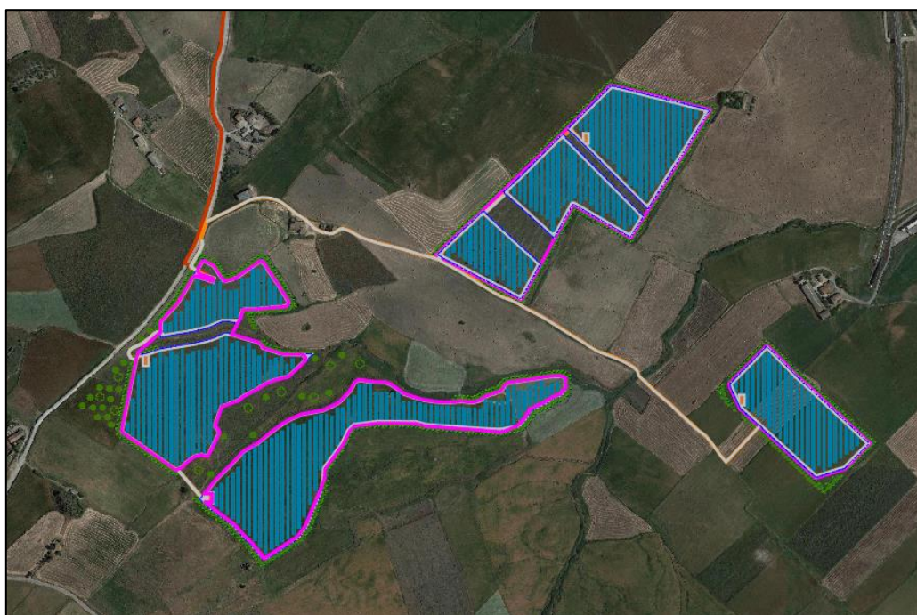
Figura 4: Layout del campo Agro-fotovoltaico e suddivisione in sottocampi.
