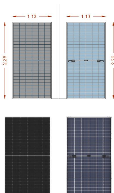
Figura 6: Dettaglio modulo FV.
