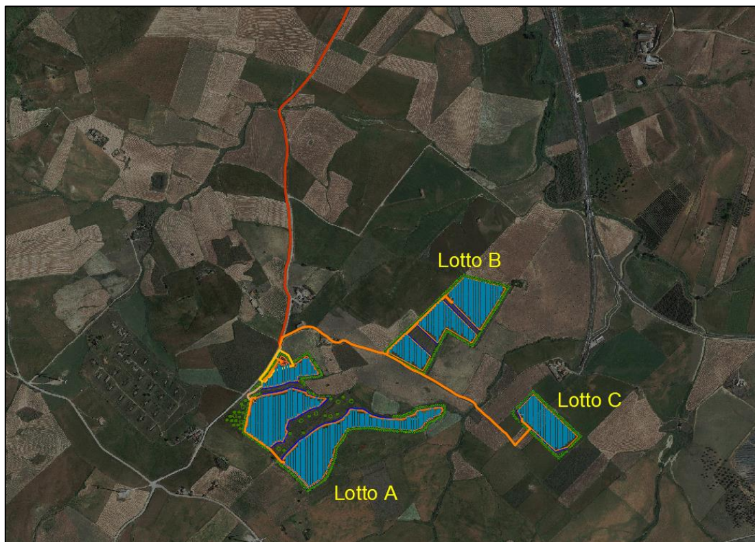
Figura 1: Corografia generale dell'area di impianto ed opere connesse su ortofoto (Rif. FV.CST01.PD.B.02)
