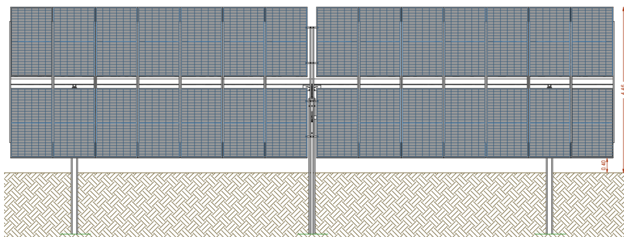
Figura 8. Tracker 2P con Moduli FV - Vista Longitudinale
