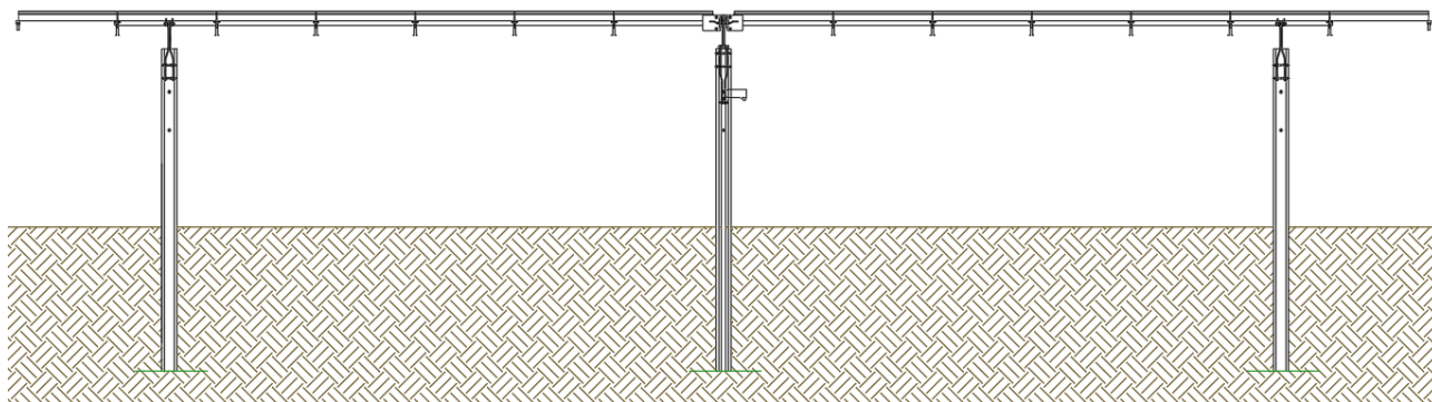
Figura 7: Tracker 2P - Vista Longitudinale in condizione di riposo
