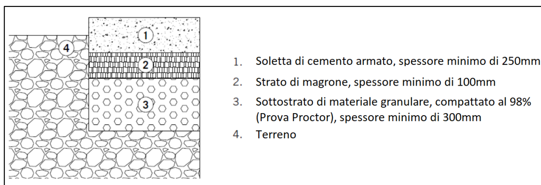
Figura 9: Indicazioni minime degli spessori del basamento, valori forniti dalla casa produttrice
