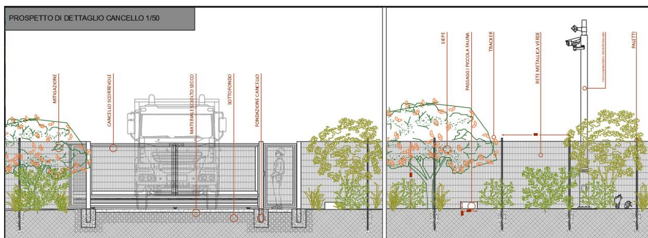
Figura 4: Particolari recinzione, cancelli e impianto di videosorveglianza (rif. Elaborato FV.CST01.PD.F.02)
