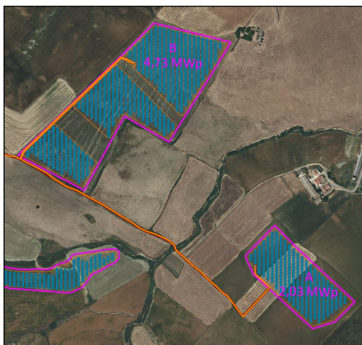
Figura 2: Layout del campo Agro-fotovoltaico e suddivisione in sottocampi –Sottocampo A - B
