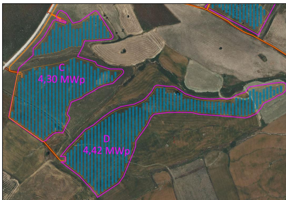
Figura 3: Layout del campo Agro-fotovoltaico e suddivisione in sottocampi –Sottocampo C - D
