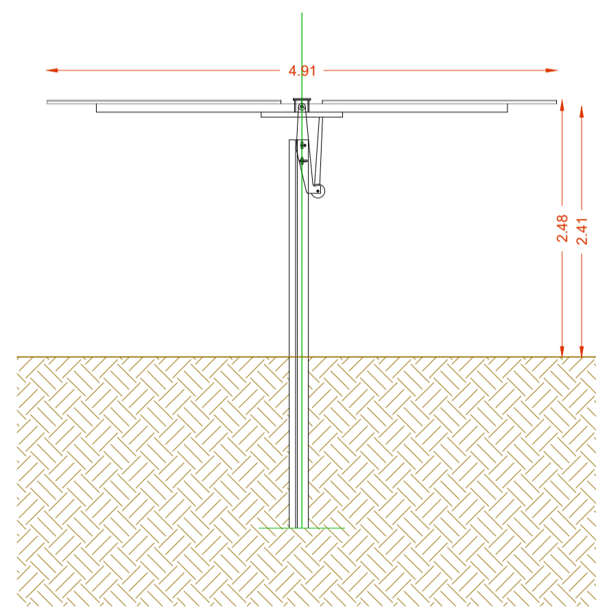
TRACKER SEZIONE TRASVERSALE - RIPOSO SCALA 1:50
