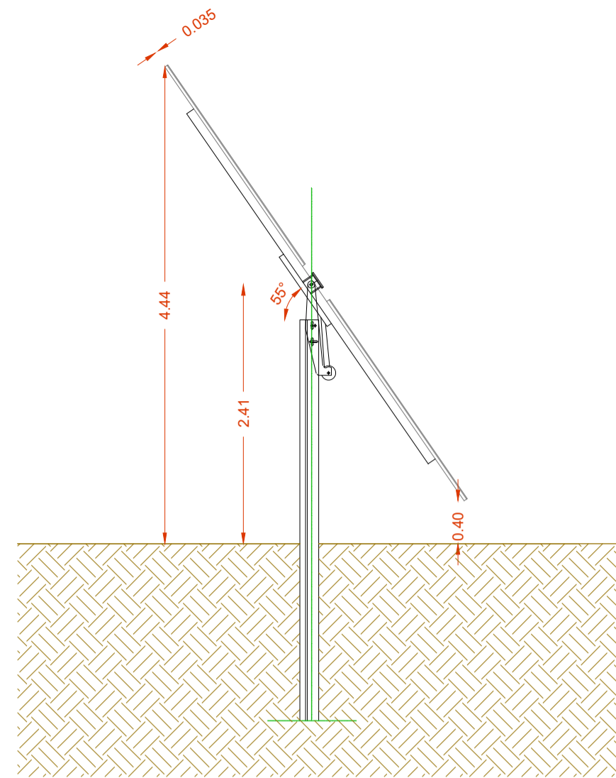
TRACKER SEZIONE TRASVERSALE - TILT SCALA 1:50
