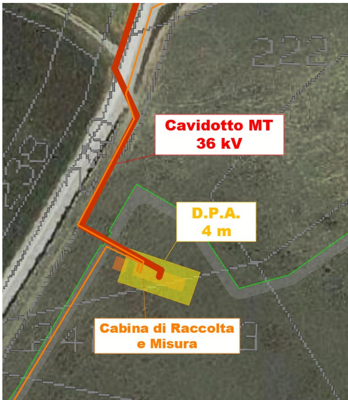
Figura 6. Rappresentazione grafica delle DPA dell'impianto considerato – Cabina di Raccolta e Misura a 36 kV
