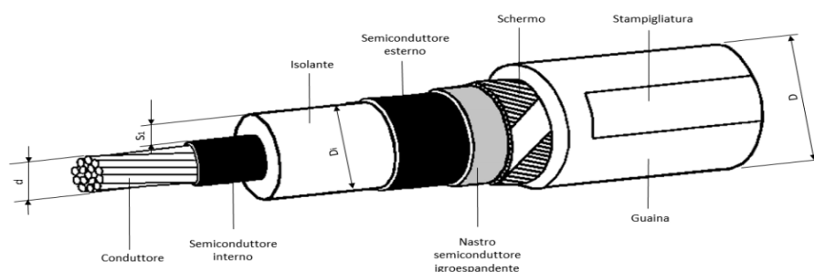
Figura 2. Rappresentazione cavo ARE4H5E
