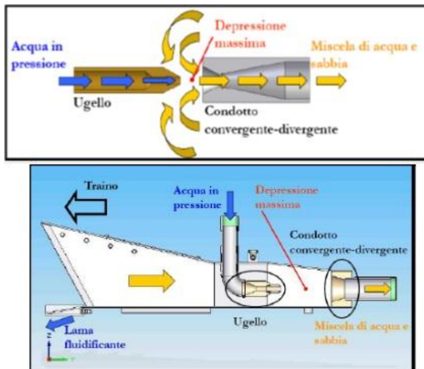
Figura 3.46 – Schema eiettore
