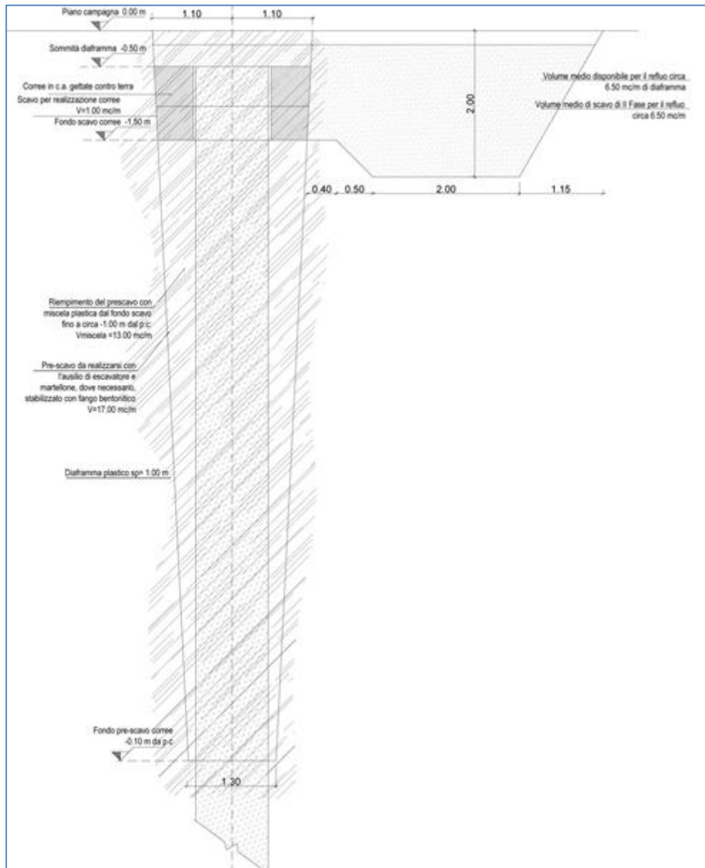
Figura 3.77 – Diaframma (spessore 100 cm) con prescavo
