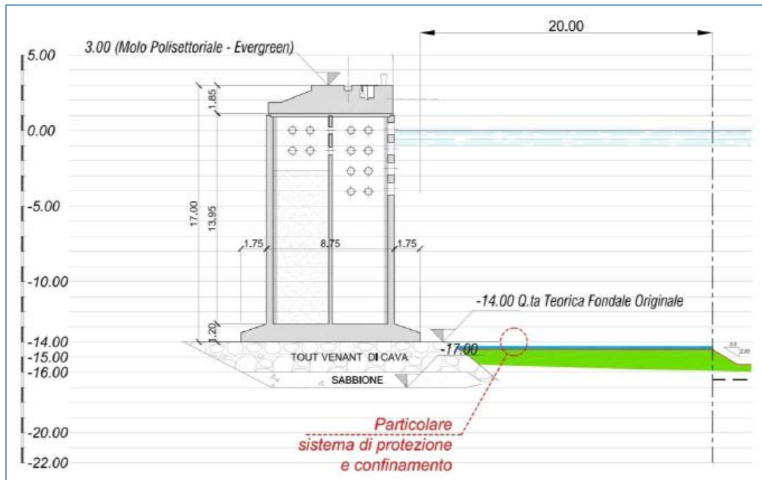
Figura 3.90 - Sezione del Molo Polisetoriale (Fonte Relazione Tecnica allegata al progetto, Codice Elaborato PUG102_PDED008)
