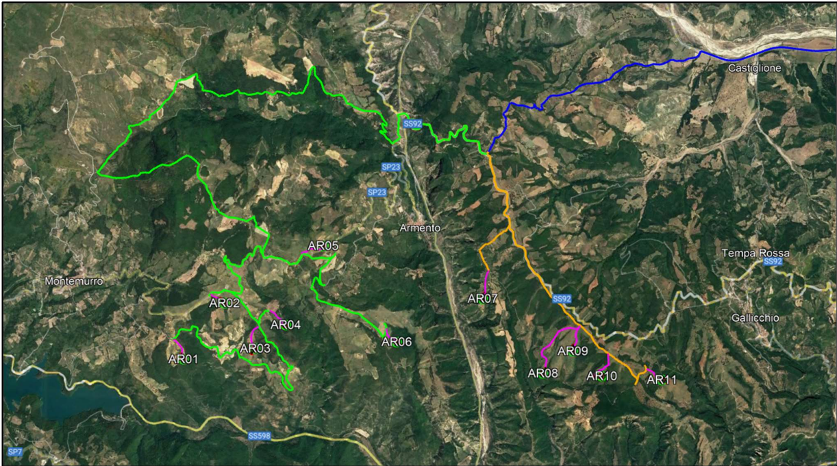
Figura 6.5: Layout di impianto con viabilità di accesso su immagine satellitare
