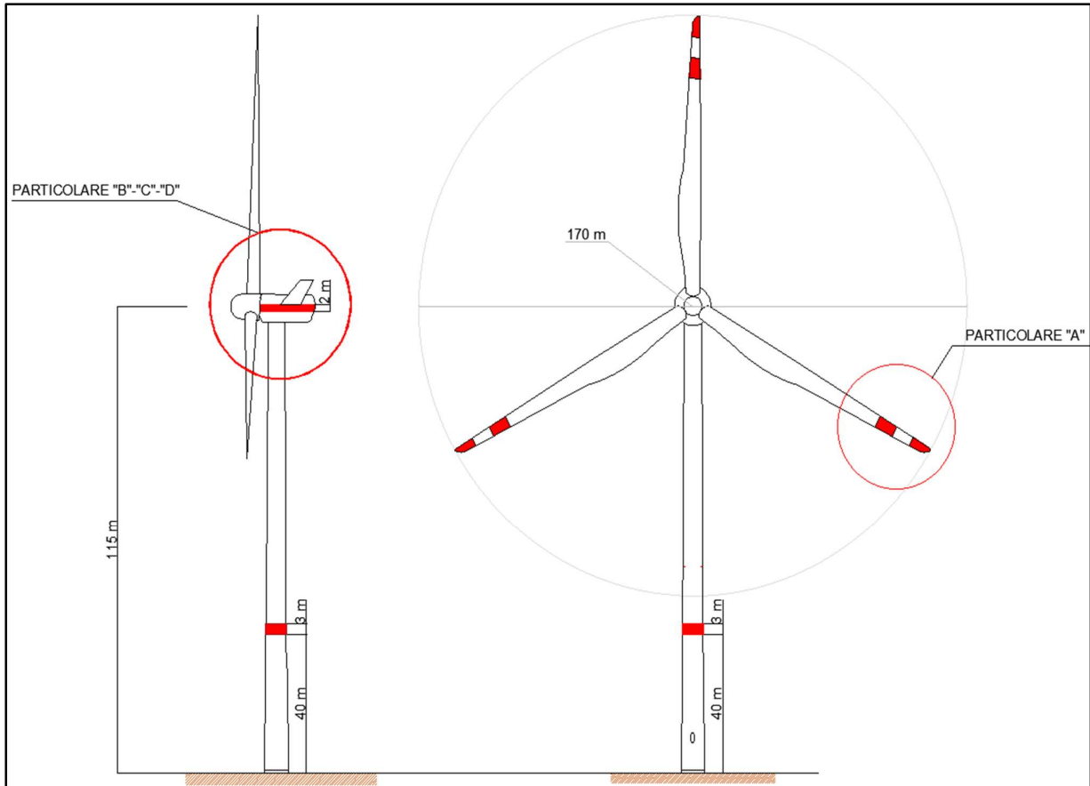
Figura 6.1.1: Profilo aerogeneratore SG170 – 6,2 MWp – HH= 115 m – D=170 m
