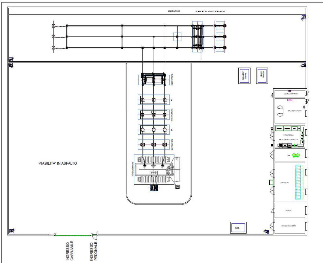
Figura 6.3.2.3: Planimetria elettromeccanica della Stazione Elettrica Utente 150/33 kV
