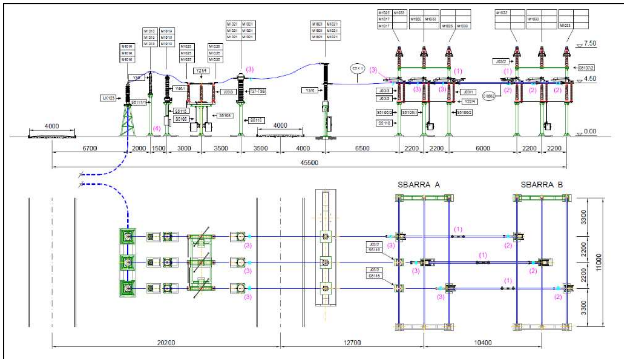
Figura 6.3.6.3: Planimetria e sezione elettromeccanica relativa alle apparecchiature dello stallo 150 kV nella stazione Terna
