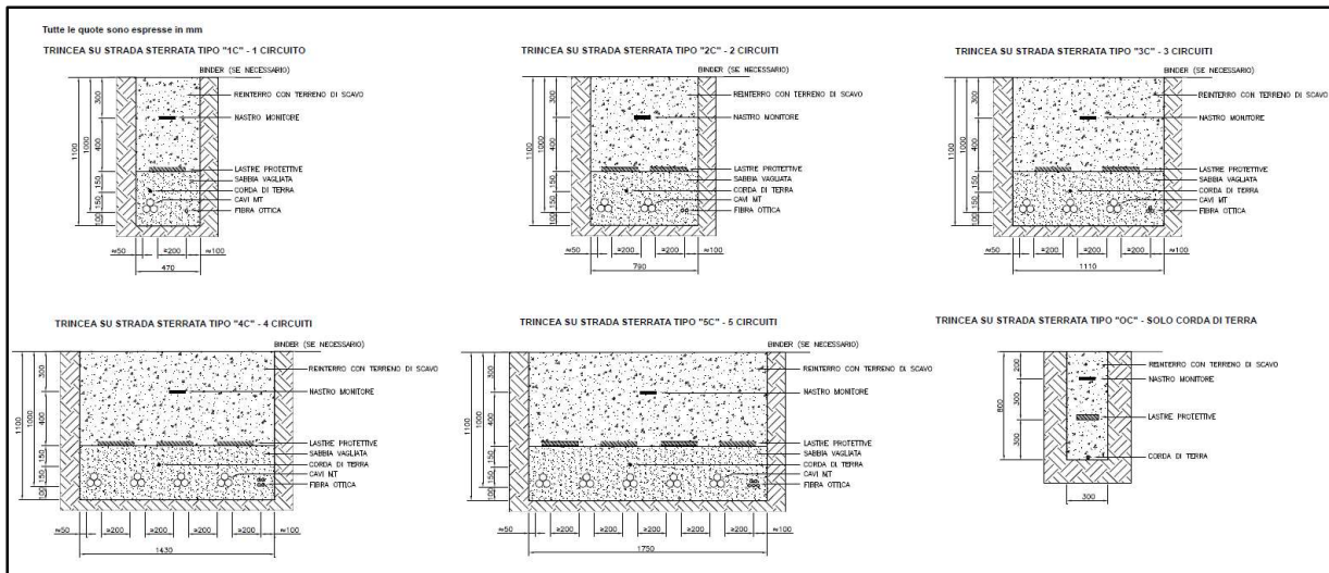
Figura 6.3.3.2: Sezioni tipiche delle trincee cavidotto per le terne di cavi in parallelo su strada sterrata
