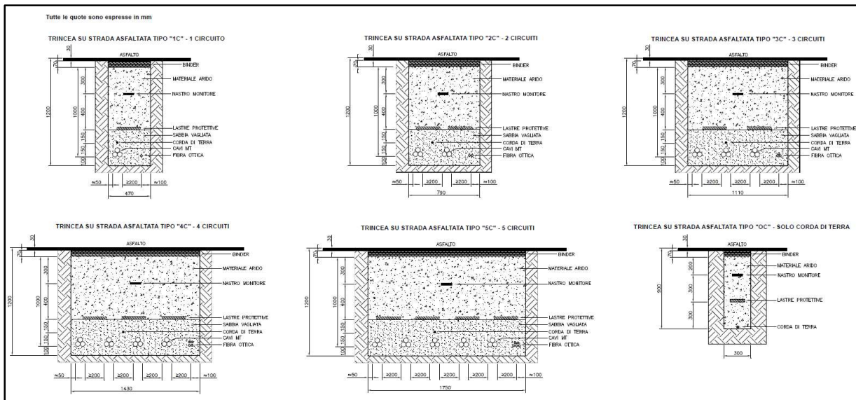
Figura 6.3.3.3: Sezioni tipiche delle trincee cavidotto per le terne di cavi in parallelo su strada asfaltata
