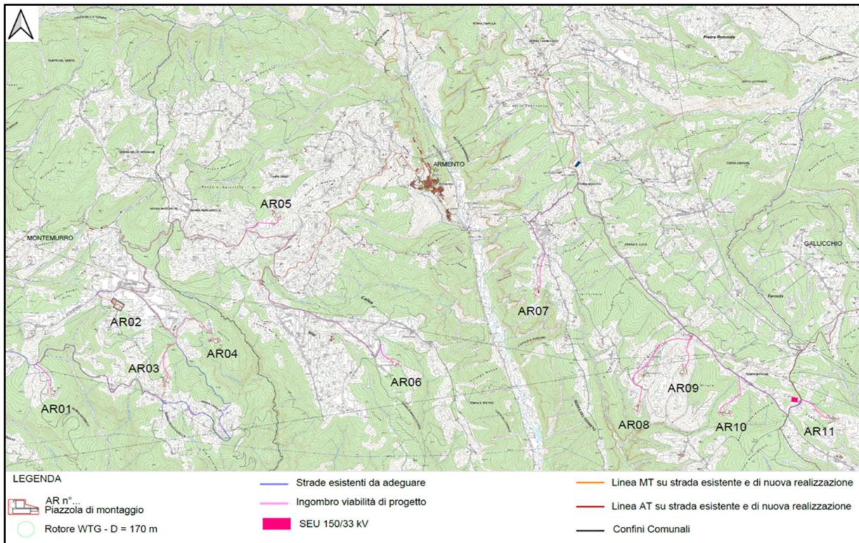
Figura 6.3: Layout d'impianto con viabilità di progetto e linee elettriche MT su CTR
