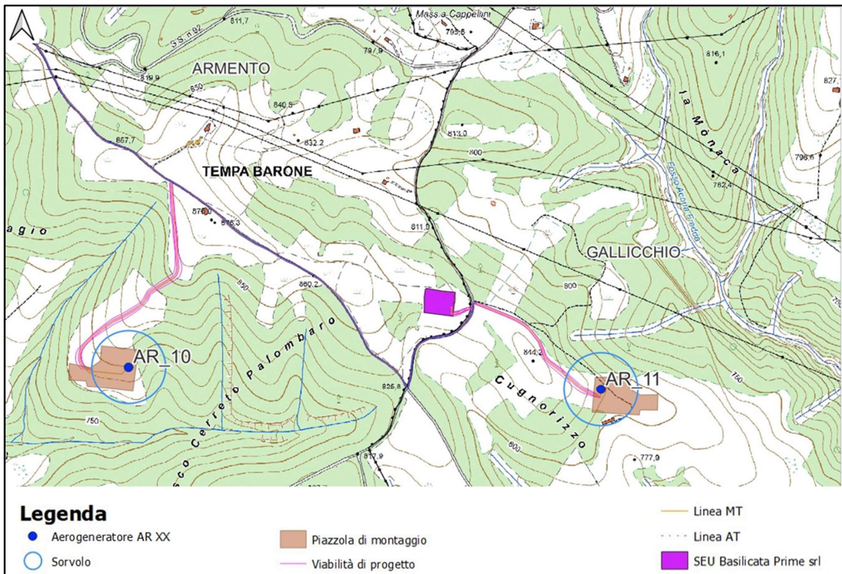
Figura 6.3.2.1: Localizzazione della SEU 150/33 Kv
