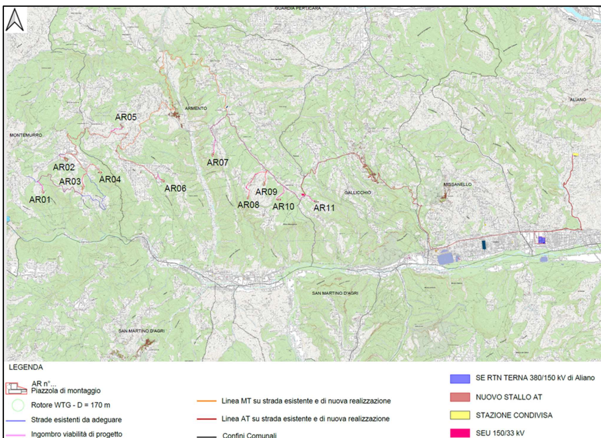
Figura 6.1: Inquadramento territoriale dell'impianto eolico Val d'Agri con i limiti amministrativi dei comuni interessati
