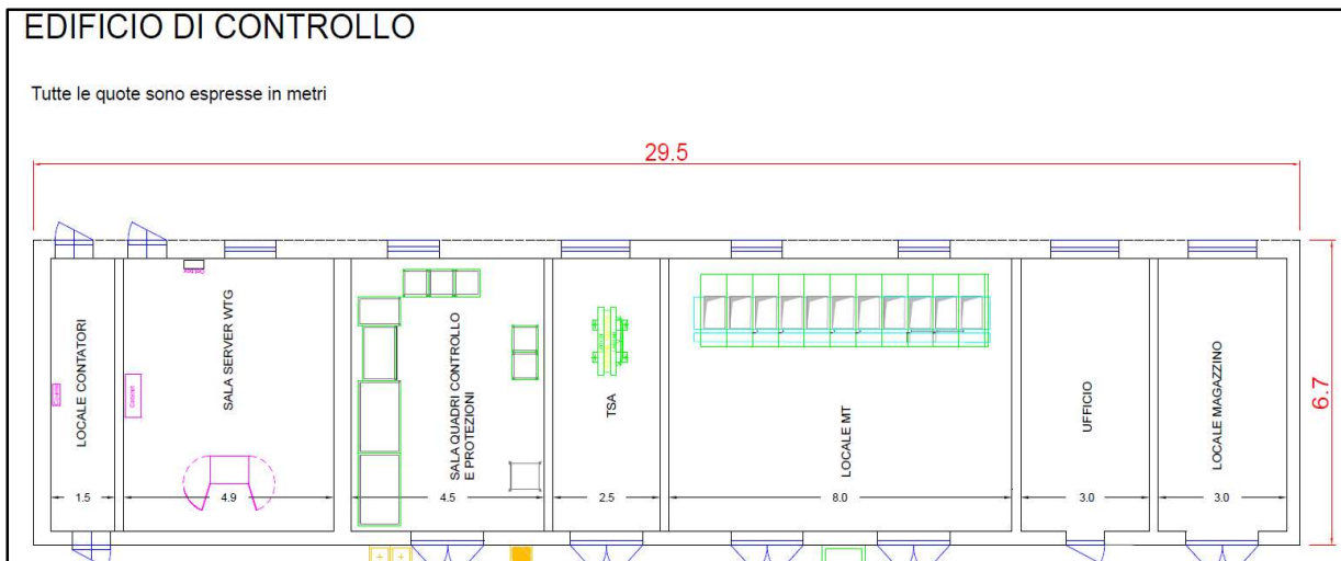
Figura 6.3.2.4: Pianta edificio di controllo SEU 150/33 kV
