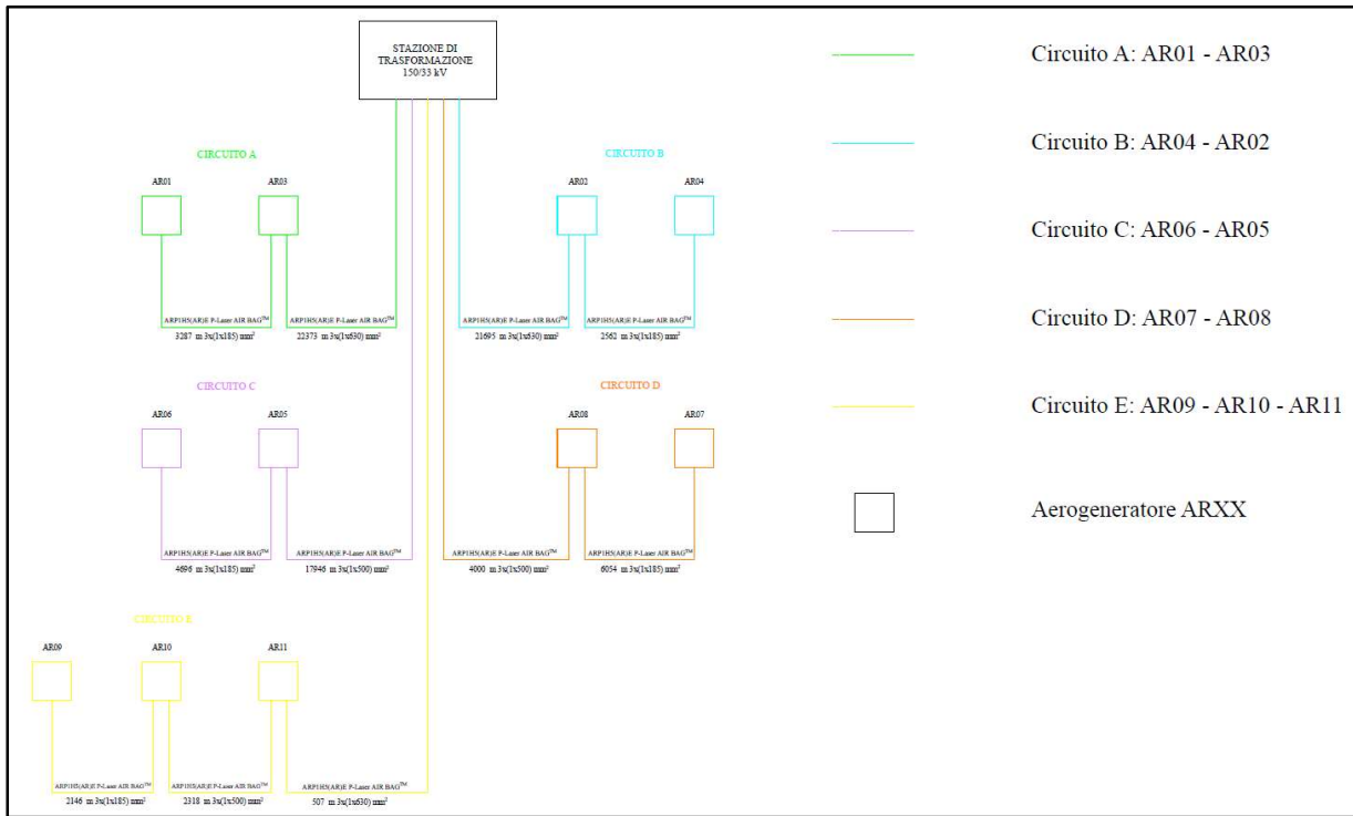
Figura 6.3.3.1: Schema a blocchi del Parco Eolico Val d'Agri
