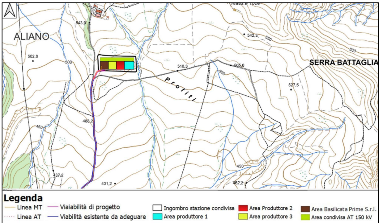
Figura 6.3.4.1: Area Sottostazione di condivisione Aliano
