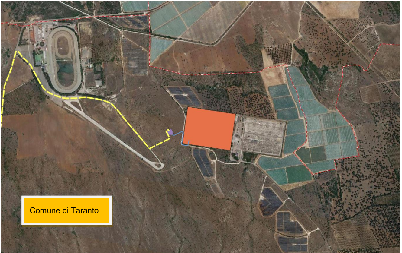
Figura 1-2: Inquadramento territoriale su Ortofoto dell'area interessata dalla Stazione Elettrica TERNA "Taranto N2" (arancione) e dalla Sottostazione Utente (viola)
