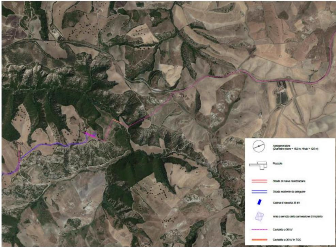
Figura 2: Inquadramento su base ortofoto del layout di impianto
