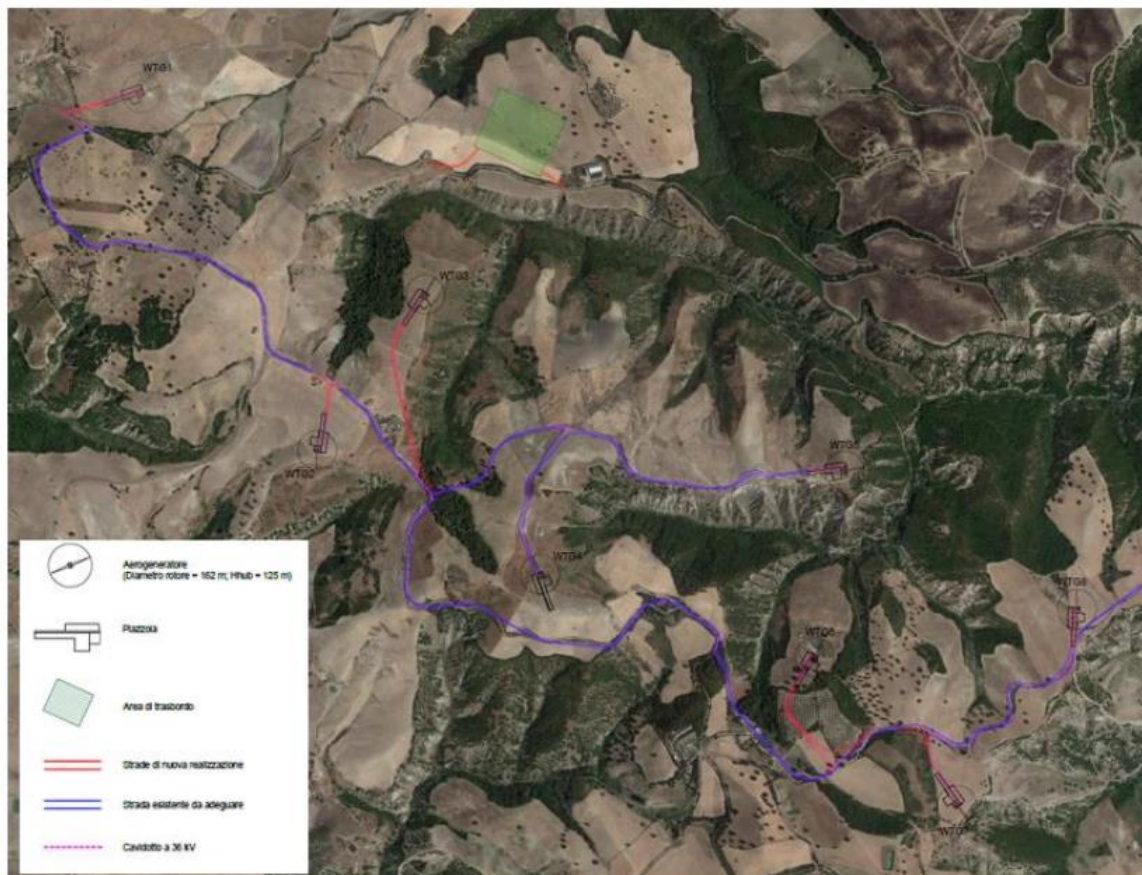
Figura 1: Inquadramento su base ortofoto del layout di impianto
