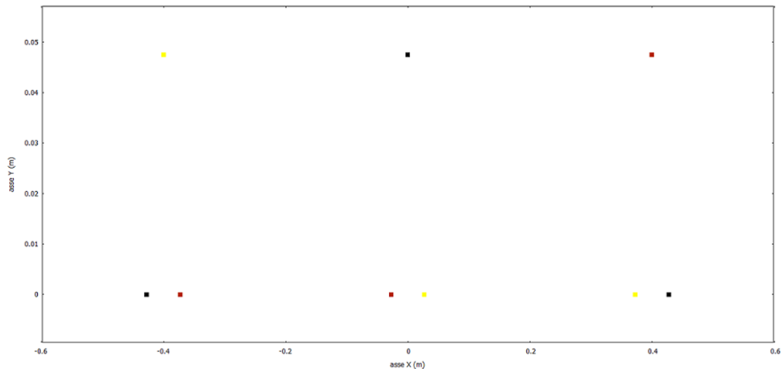
Figura 6 – Geometria disposizione cavi AT
