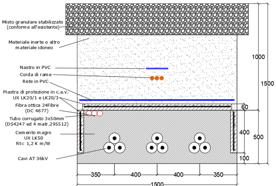
Figura 5 – Sezione cavidotto di connessione AT a 36kV su strada sterrata
