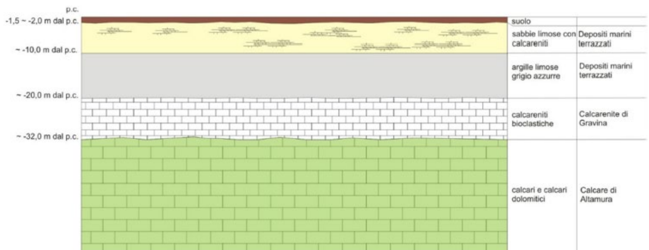
Figura 18 – Sezione geologica schematica
