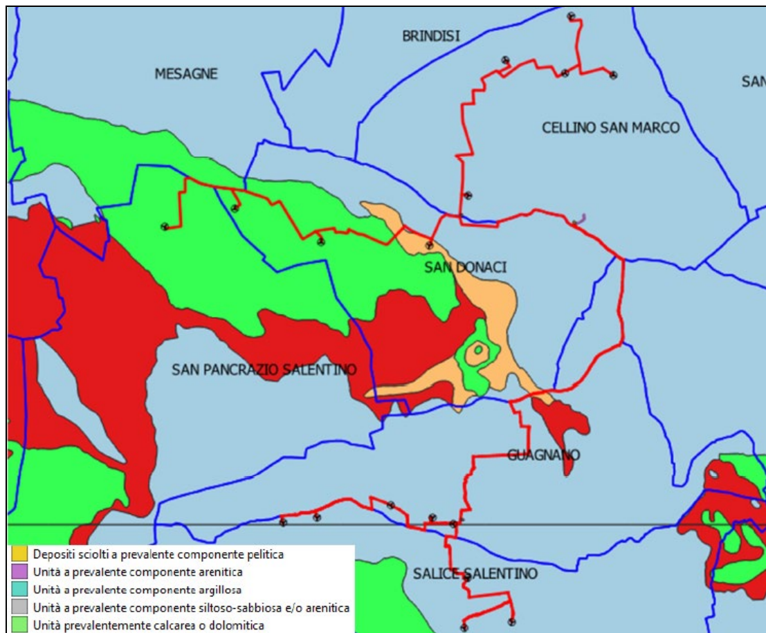
Figura 17 - Carta Geolitologica
