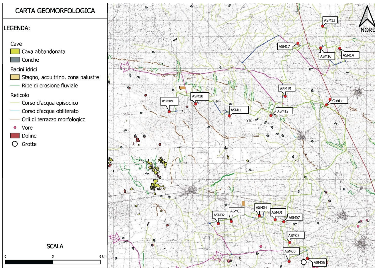
Figura 16 - Carta Geomorfologica
