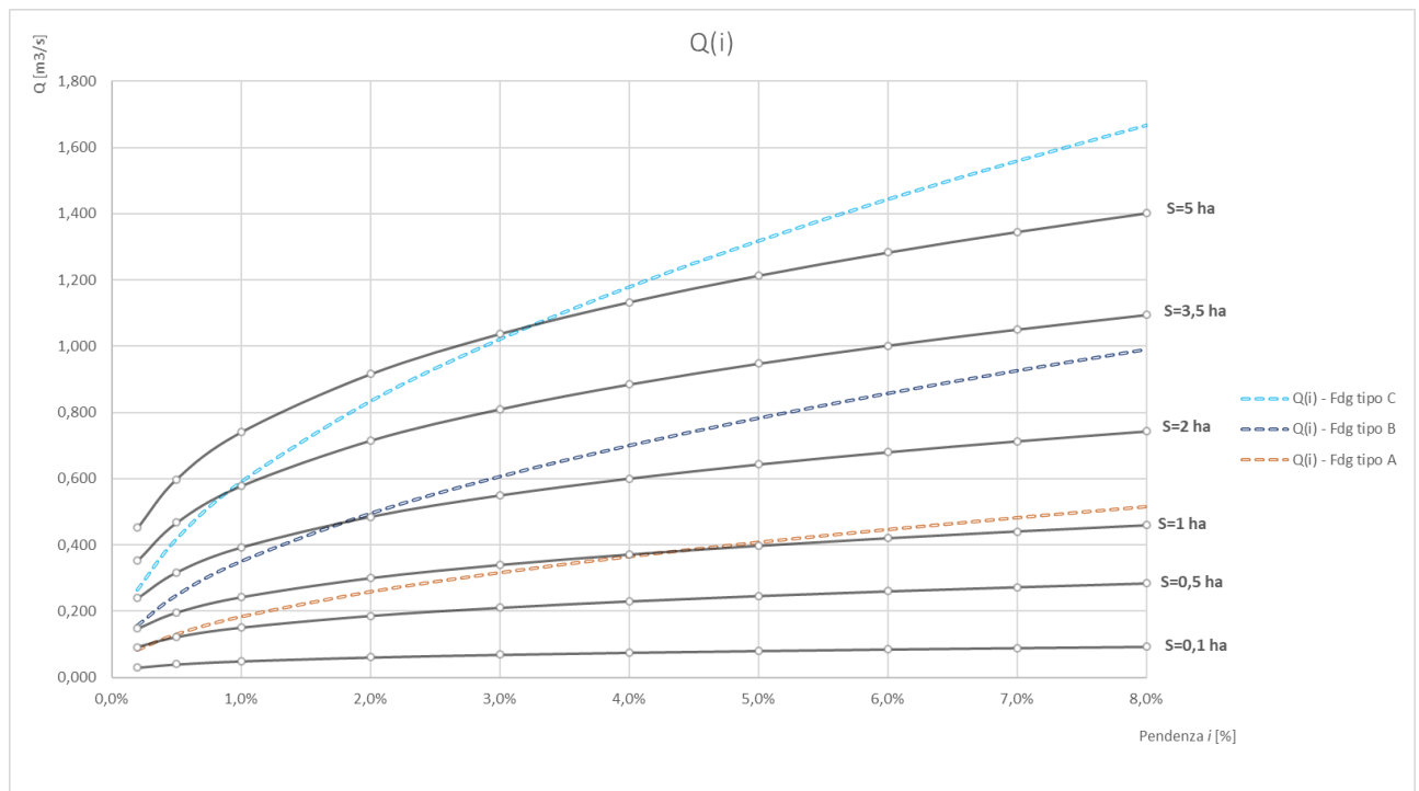
Fig. 12: Definizione del grafico Q(i) per il caso in studio, con riferimento ad un tempo di ritorno T pari a 50 anni.
