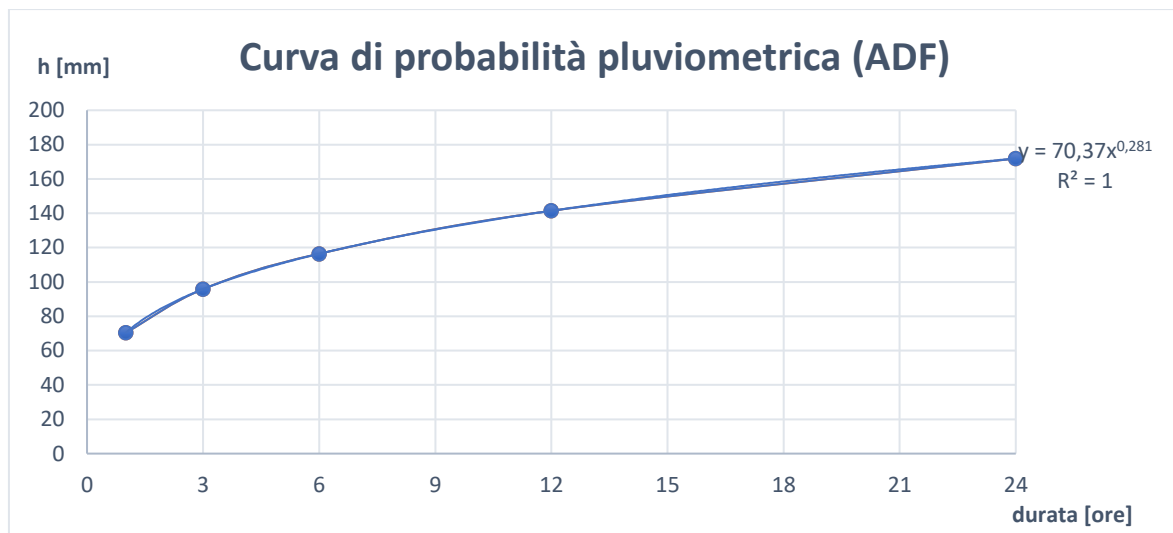
Fig. 9 Curva di probabilità pluviometrica ADF (Altezza-Durata-Frequenza) relative all'area oggetto di studio e per il tempo di ritorno di progetto ( T=50 anni).
