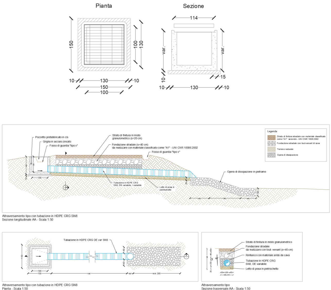
Figura 5: Sezioni longitudinali, trasversali e pianta dell'attraversamento tipo.
