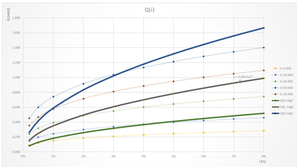
Fig. 11 Tipologia di grafico Q(i) con individuazione delle zone omogenee per il pre-dimensionamento dei fossi di guardia.
