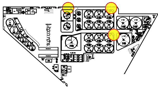
PLANIMETRIA GENERALE
