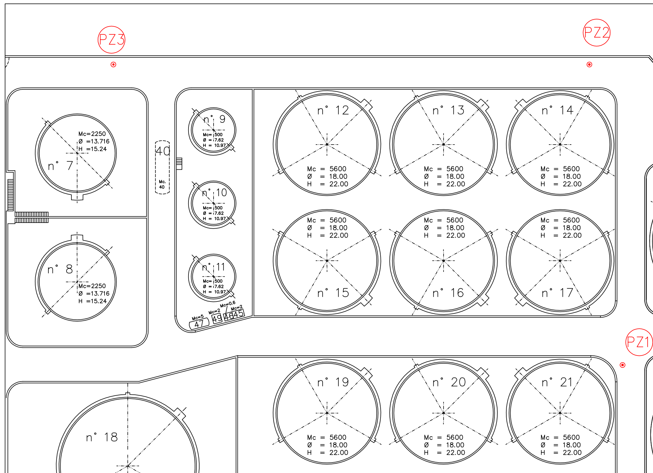
PIANTA PARTICOLARE - 1:200
