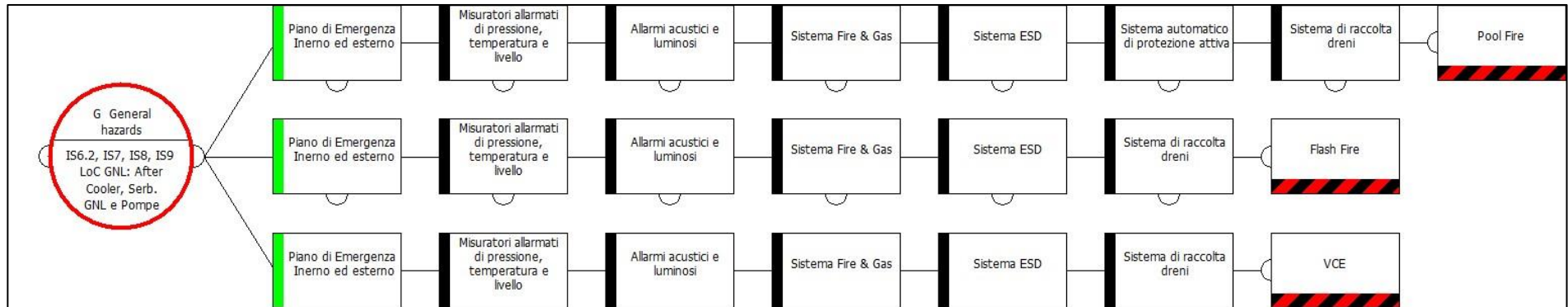
Bow Tie Misure Mitigative per IS6.2, IS7, IS8, IS9 Perdita di contenimento di GNL da After cooler, Serbatoi o Pompe
