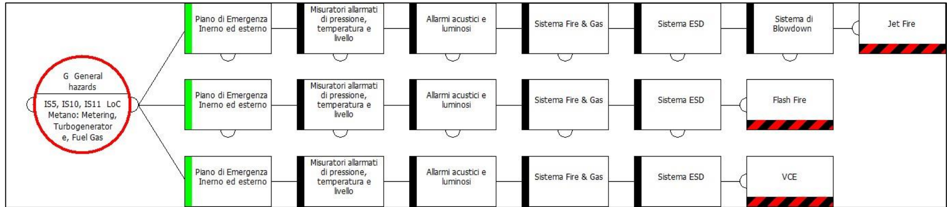
Bow Tie Misure Mitigative per IS5, IS10 e IS11, Perdita di contenimento di Metano da stazione di metering, turbogeneratore o Fuel Gas
