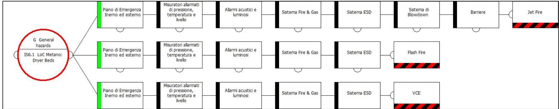
Bow Tie Misure Mitigative per IS6.1 Perdita di contenimento di Metano da Dryer beds
