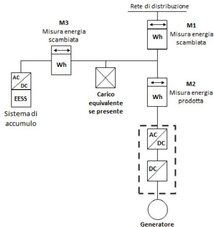
Figura 7: Misura dei flussi di energia con accumulo posizionato nella parte d'impianto in corrente alternata a monte del contatore dell'energia generata
