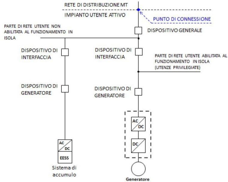
Figura 6: Schema di principio sistema di accumulo
