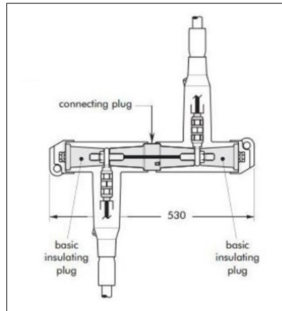
Figura 13: Dettaglio giunzione tra cavi MT all'interno del pozzettone di sezionamento
