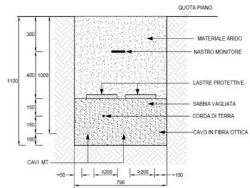
Figura 10: Sezione scavi su strada asfaltata e sterrata (2 terne di cavi MT)
