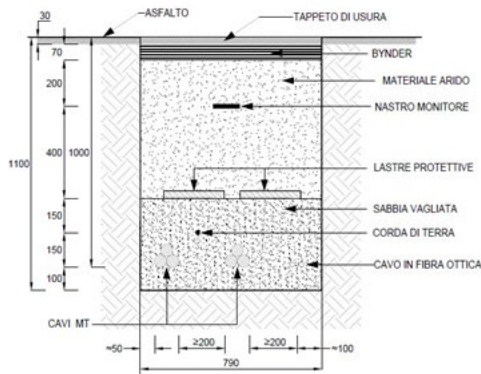
Figura 10: Sezione scavi su strada asfaltata e sterrata (2 terne di cavi MT)
