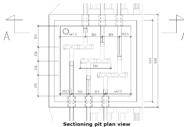
Figura 11: Vista in pianta dei giunti sconnettabili all'interno dei pozzettoni di sezionamento
