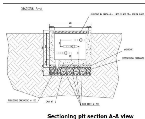
Figura 12: Vista in sezione dei giunti sconnettabili all'interno dei pozzettoni di sezionamento
