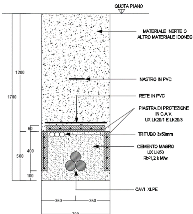
Figura 15: Sezione tipo cavi AT
