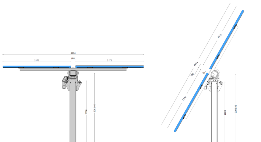
Figura 3: Schema della struttura - sezione
