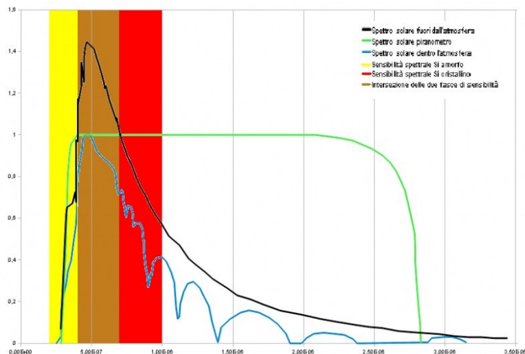
Figura 4: La misura dell'irraggiamento solare
