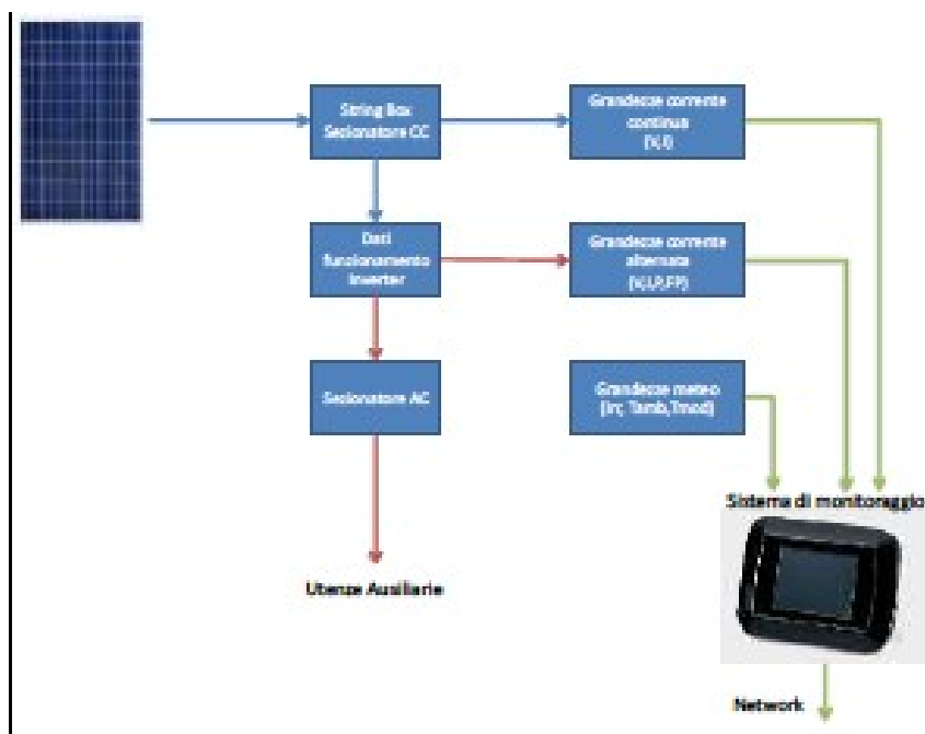
Figura 11: Architettura sistema di monitoraggio
