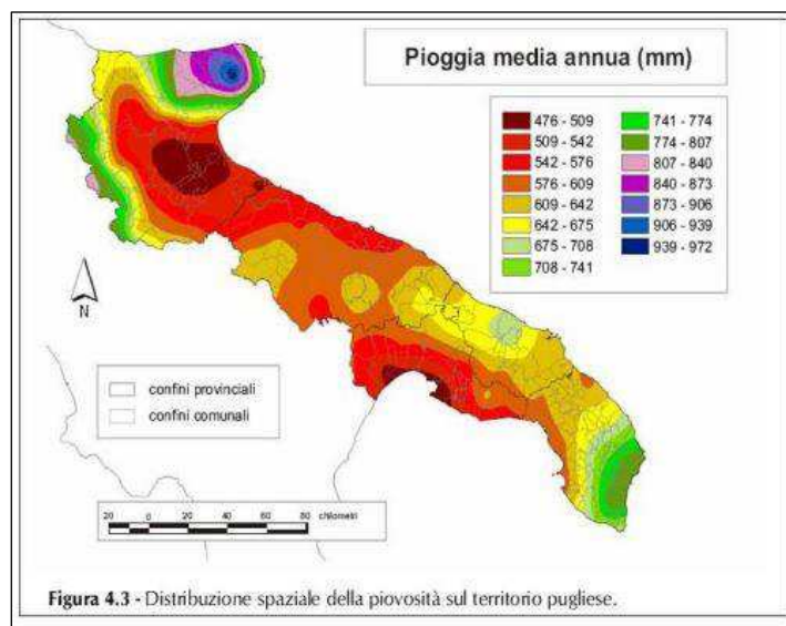
Tav.7 - Distribuzione precipitazioni
