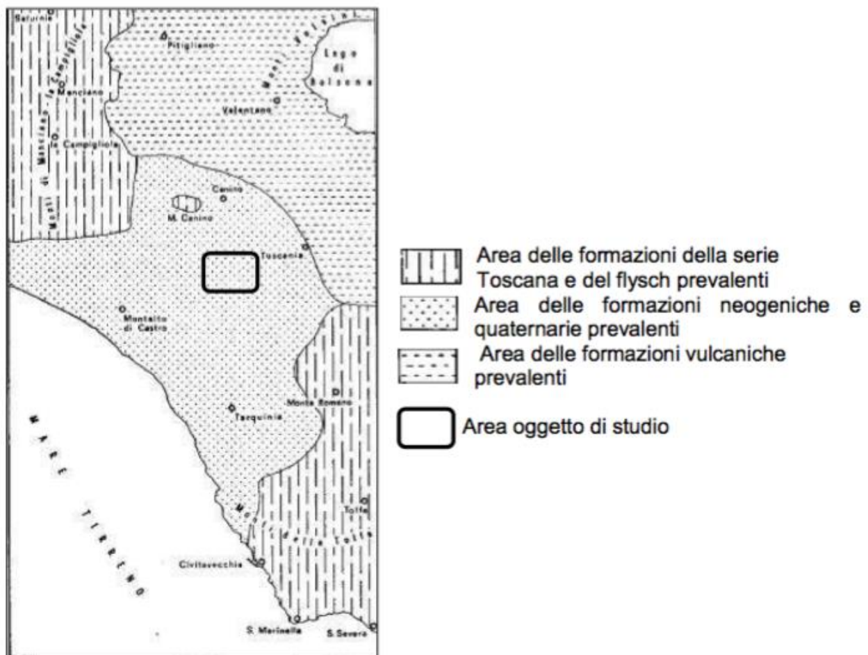
Figura 5 – Inquadramento geologico
