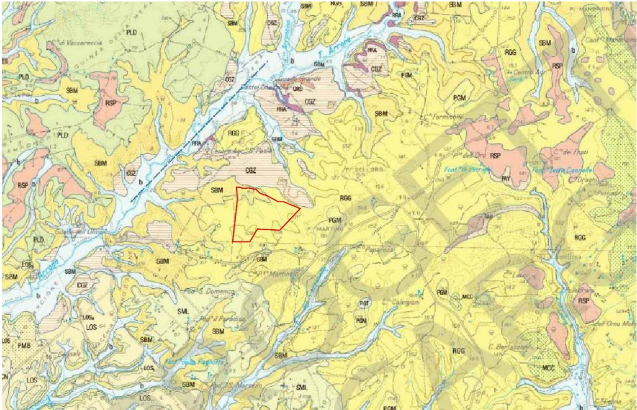
Figura 6 – CARTA GEOLOGICA
