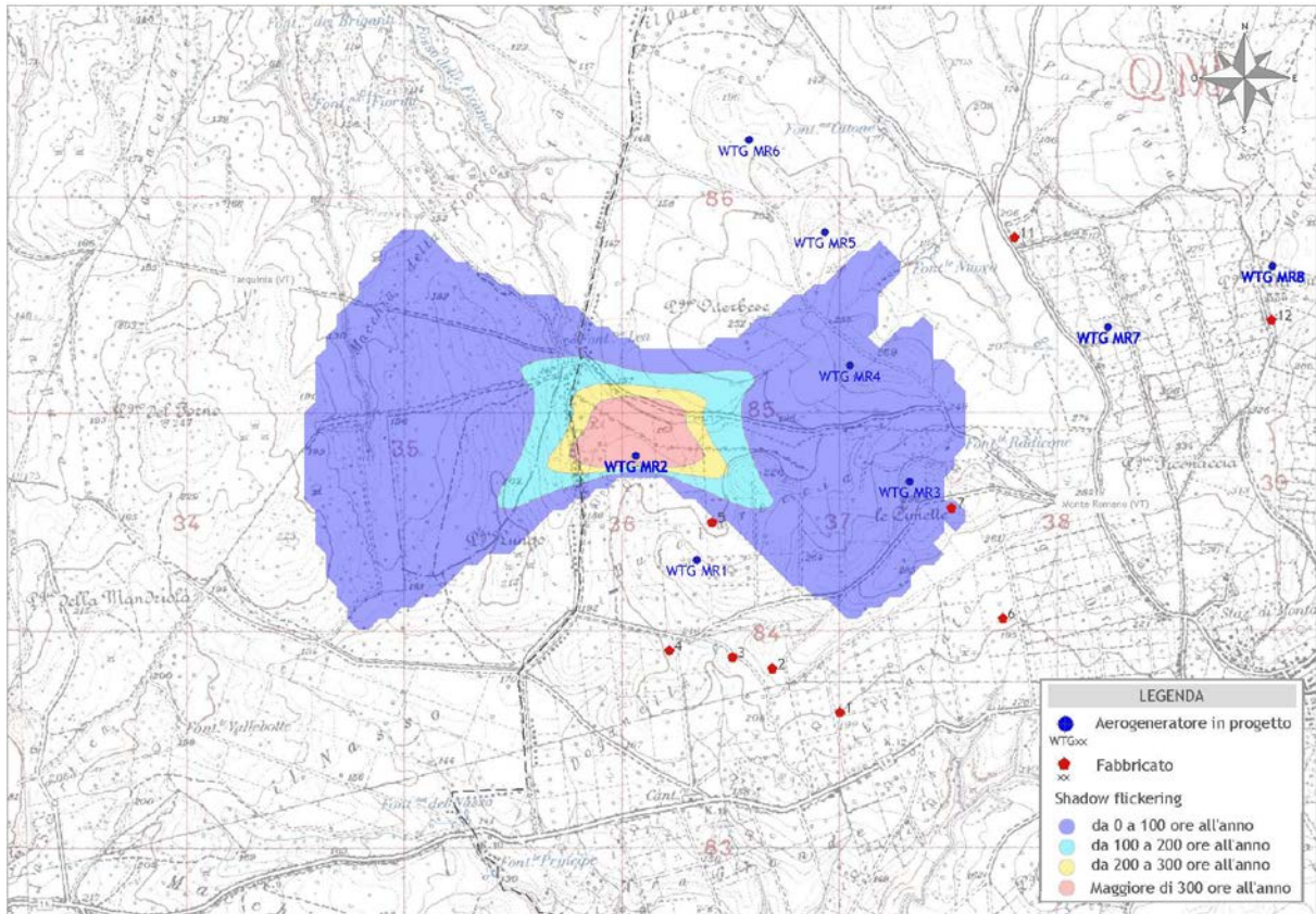
Figura 3 - Mappa di impatto potenziale per l'aerogeneratore WTG MR2
