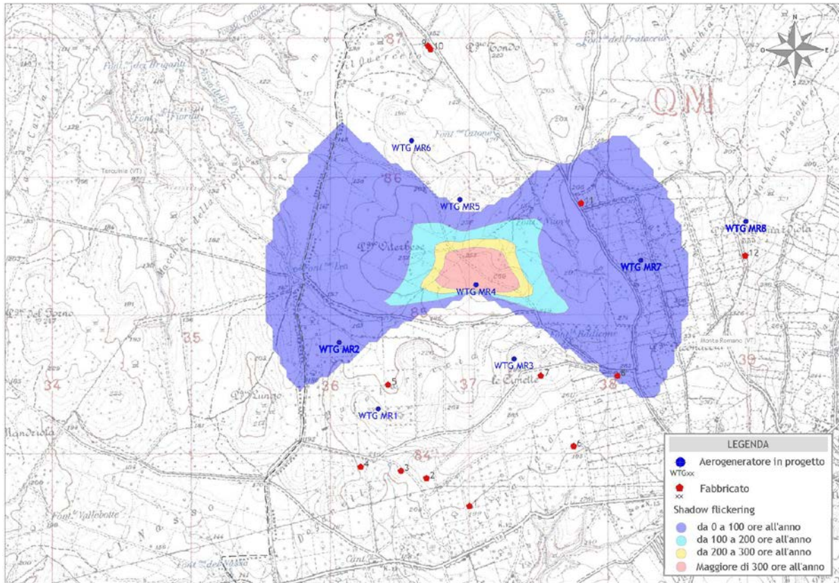
Figura 5 - Mappa di impatto potenziale per l'aerogeneratore WTG MR4
