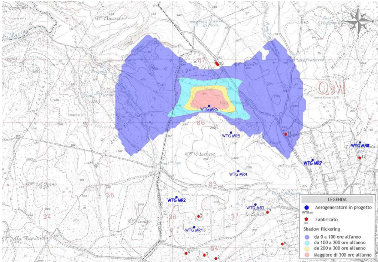
Figura 7 - Mappa di impatto potenziale per l'aerogeneratore WTG MR6
