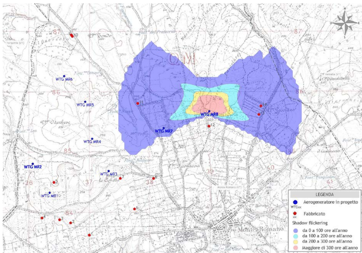
Figura 9 - Mappa di impatto potenziale per l'aerogeneratore WTG MR8
