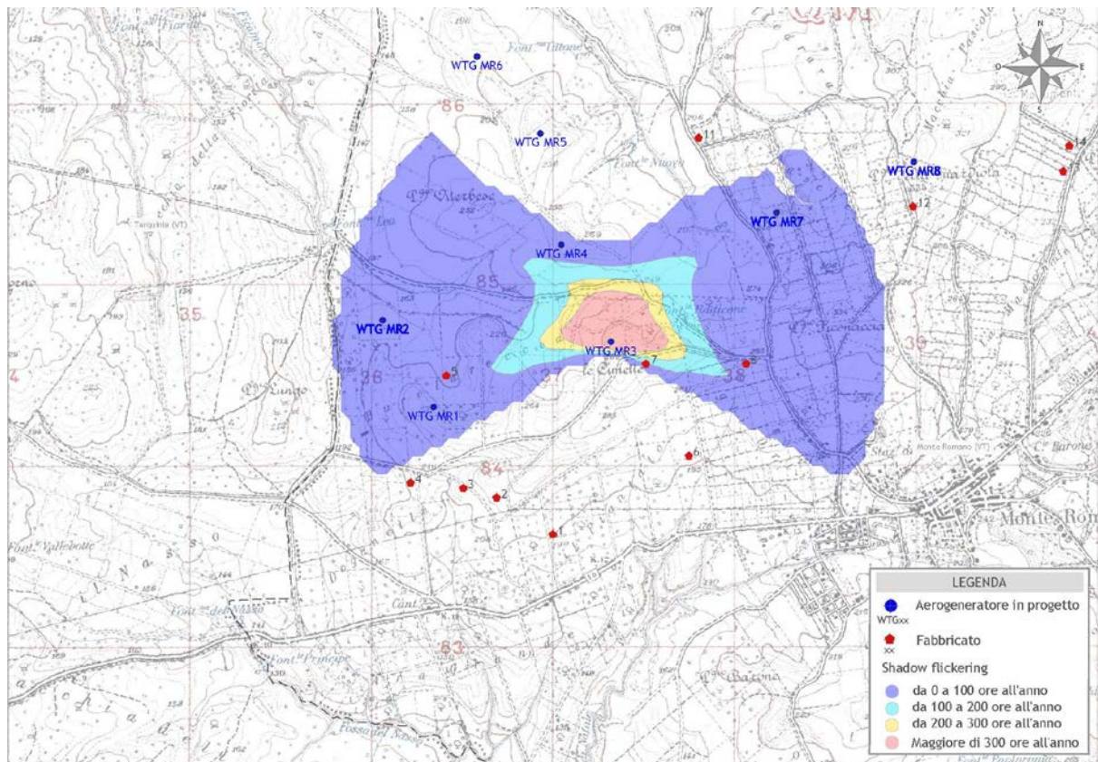
Figura 4 - Mappa di impatto potenziale per l'aerogeneratore WTG MR3
