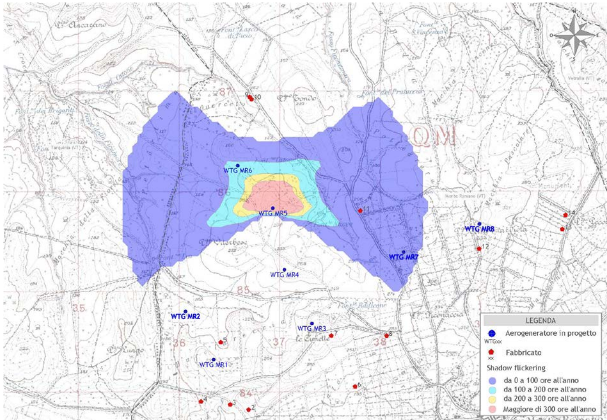
Figura 6 - Mappa di impatto potenziale per l'aerogeneratore WTG MR5
