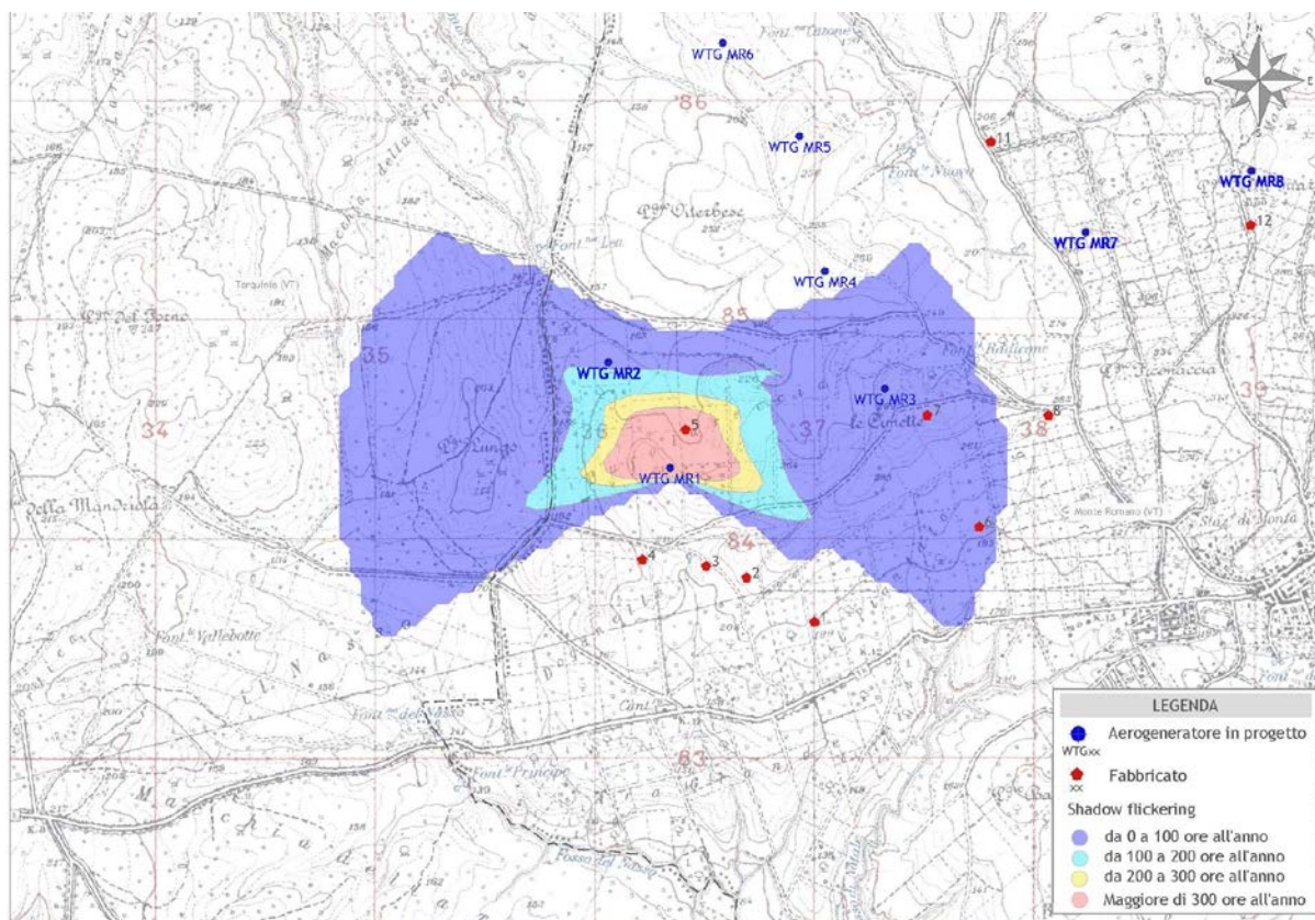
Figura 2 - Mappa di impatto potenziale per l'aerogeneratore WTG MR1
