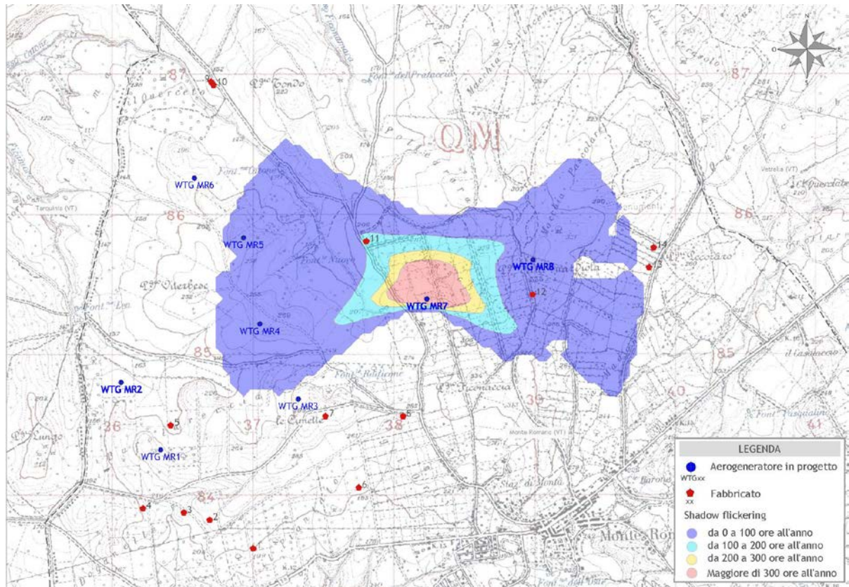
Figura 8 - Mappa di impatto potenziale per l'aerogeneratore WTG MR7
