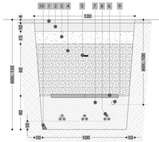
Figura 2: Sezione tipo cavidotto M.T. composta da tre terne da 630 mm 2
