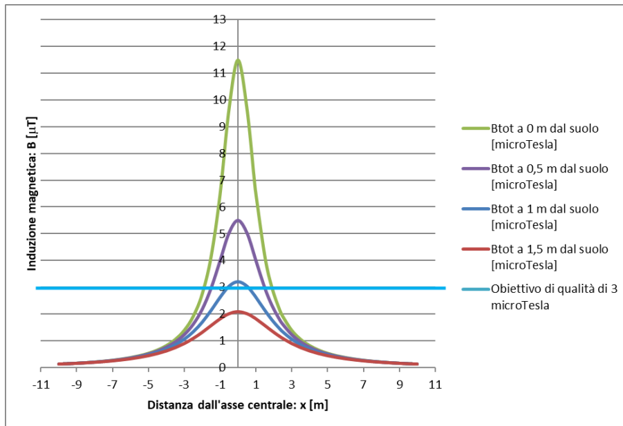
Figura 3: Andamento del campo magnetico generato dal cavidotto M.T., composta da tre terne da 630 mm 2
