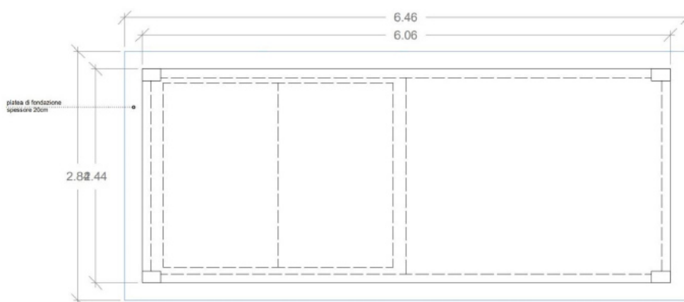
Figure 9 – Layout Cabina di sottocampo
