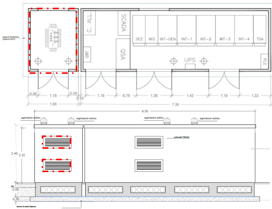
Figure 11 – Cabina di centrale - layout
