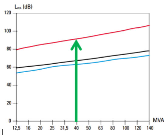
Figure 14 – Potenza sonora del trasformatore – L_w(A) in dB(A)
