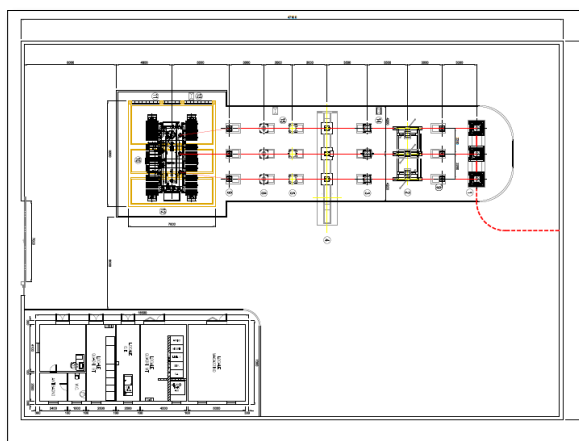
Figure 13 – Layout Sottostazione elettrica
