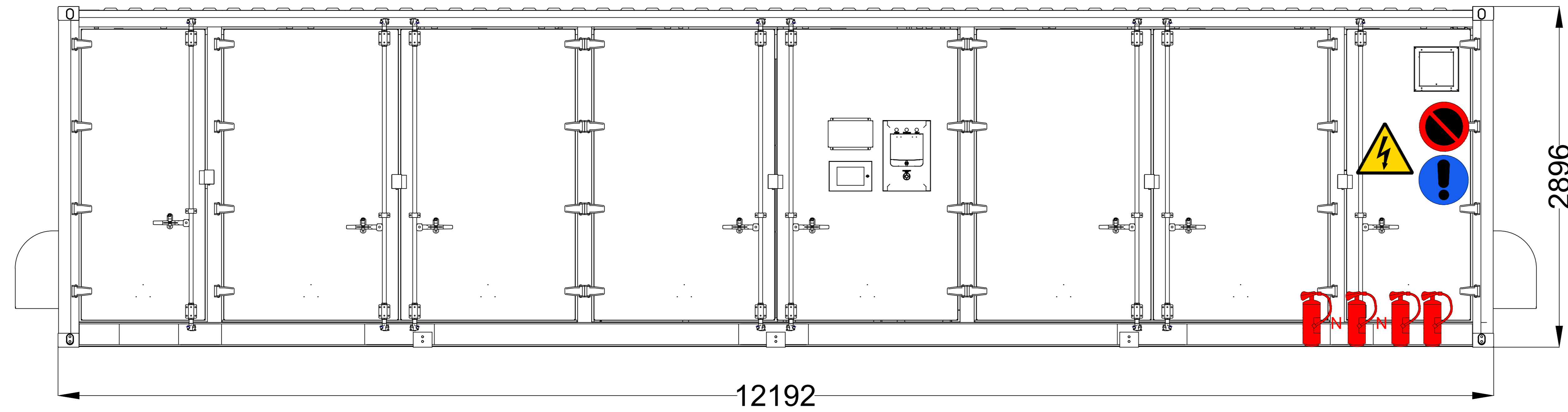
VISTA FRONTALE
