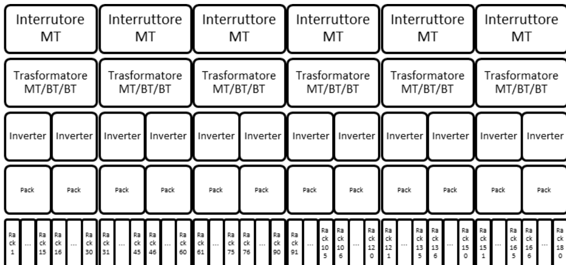
Configurazione BESS
