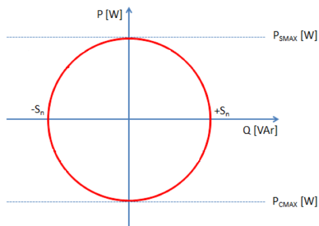
Figura 10: Capability del PCS a tensione nominale
