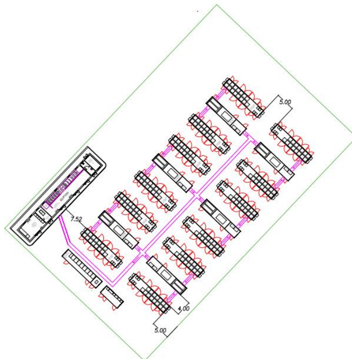
Figura 5: Area Sistema di Accumulo – Pianta
