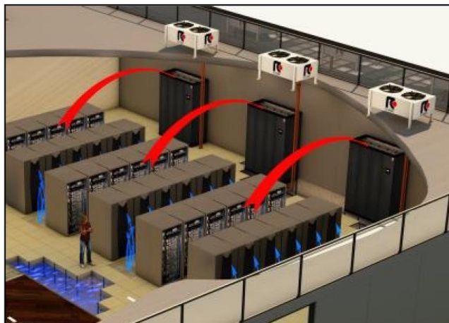
Figura 11: Esempio di installazione di impianto HVAC in container batterie
