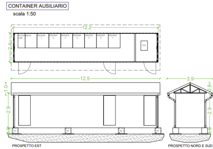
Figura 6: Container ausiliari - Pianta e Prospetto
