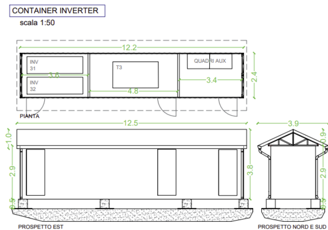
Figura 7: Container inverter - Pianta e Prospetto
