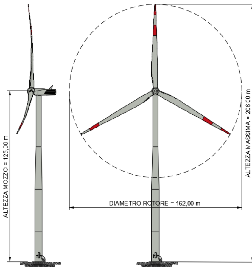
Figura 1: dimensioni delle parti che costituiscono l'aerogeneratore
