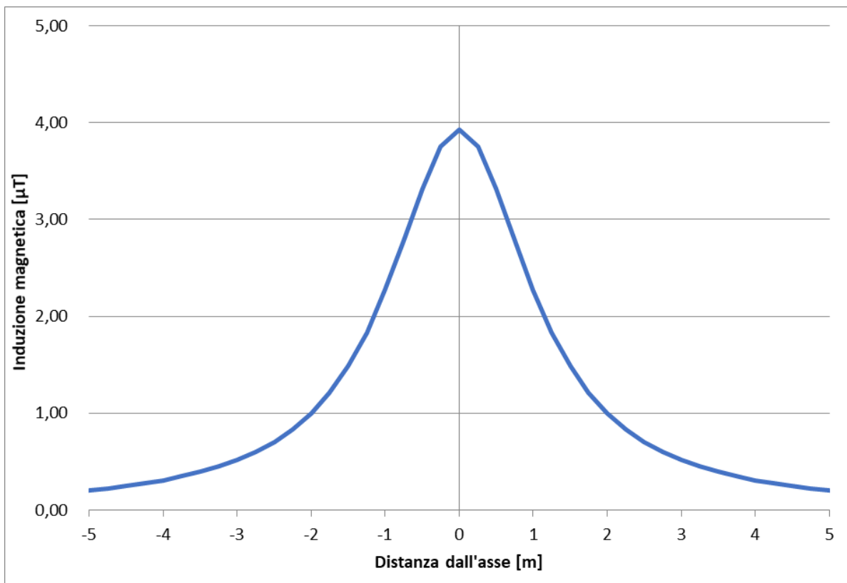
Figura 5-17 – Andamento campo magnetico – Sezione 13
