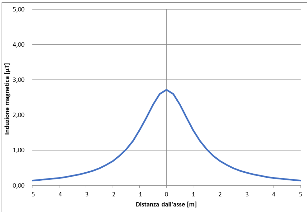
Figura 5-7 – Andamento campo magnetico – Sezione 3
