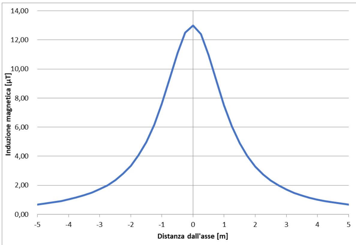
Figura 5-15 – Andamento campo magnetico – Sezione 11
