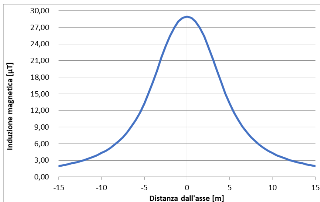
Figura 5-21 – Andamento campo magnetico sbarre AT stallo condiviso
