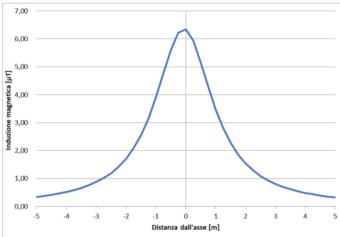
Figura 5-12 – Andamento campo magnetico – Sezione 8
