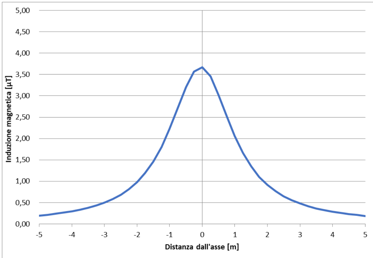
Figura 5-8 – Andamento campo magnetico – Sezione 4
