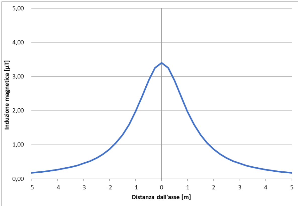
Figura 5-10 – Andamento campo magnetico – Sezione 6
