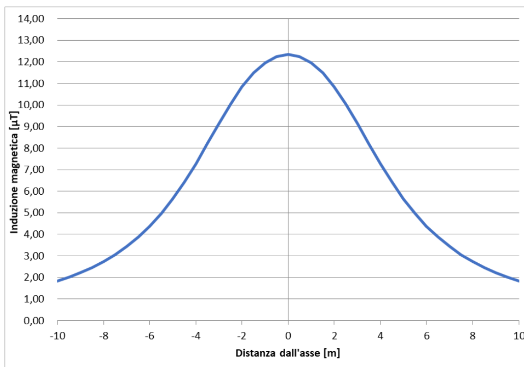
Figura 5-20 – Andamento campo magnetico sbarre AT stazione utente
