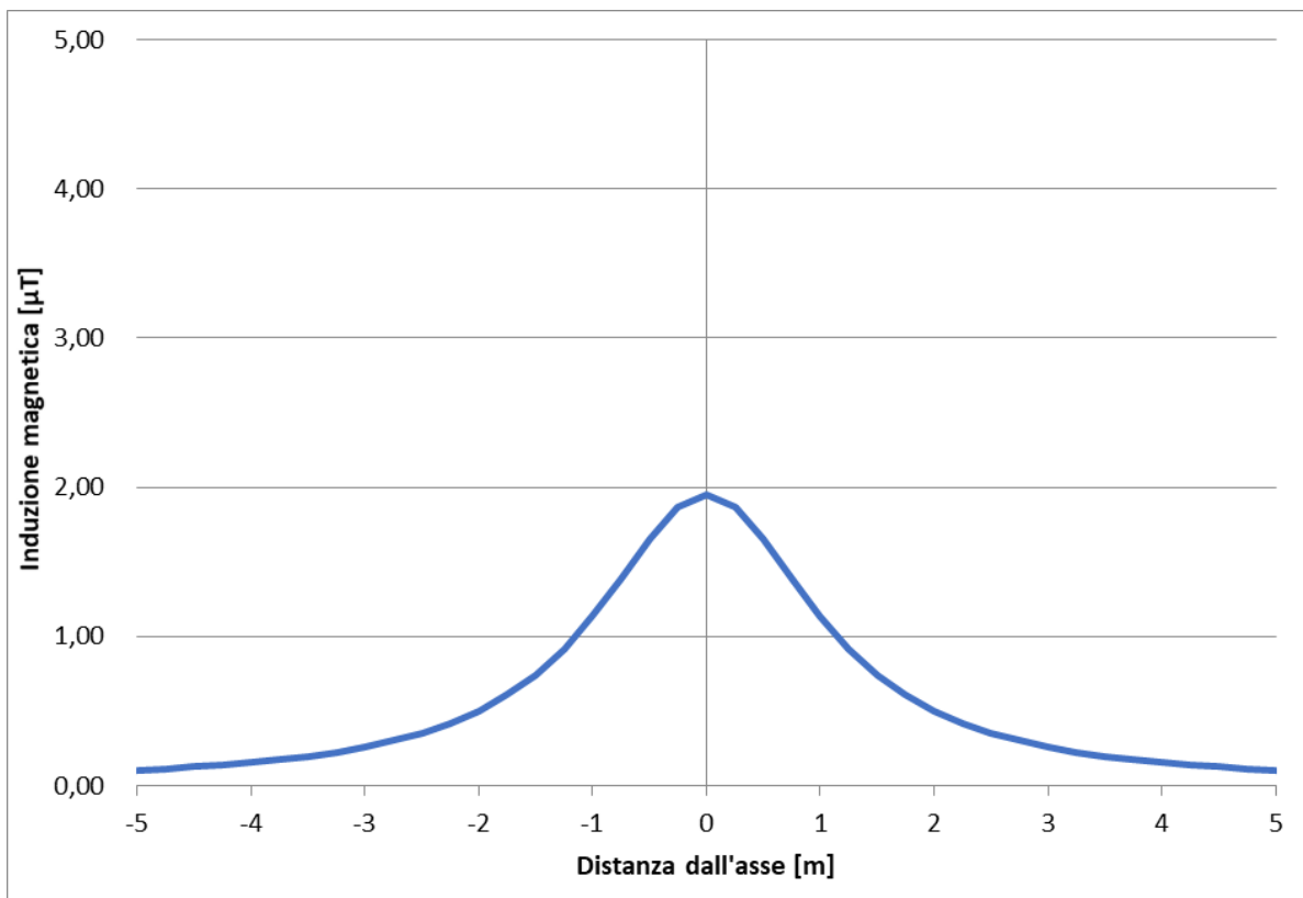
Figura 5-9 – Andamento campo magnetico – Sezione 5
