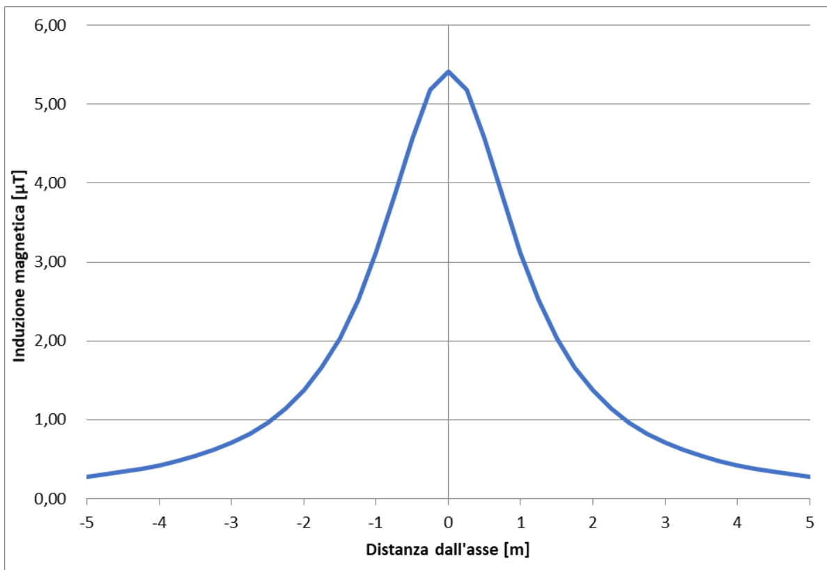
Figura 5-11 – Andamento campo magnetico – Sezione 7
