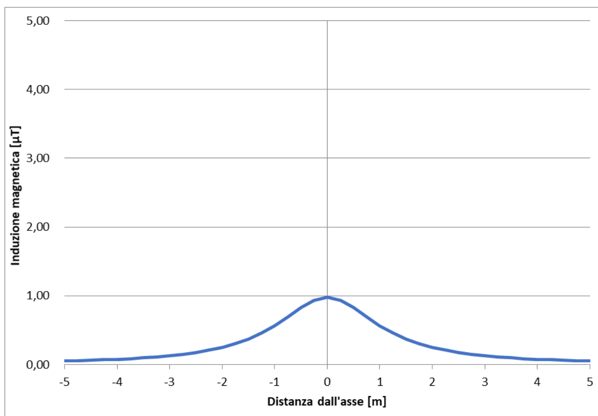
Figura 5-5 – Andamento campo magnetico – Sezione 1
