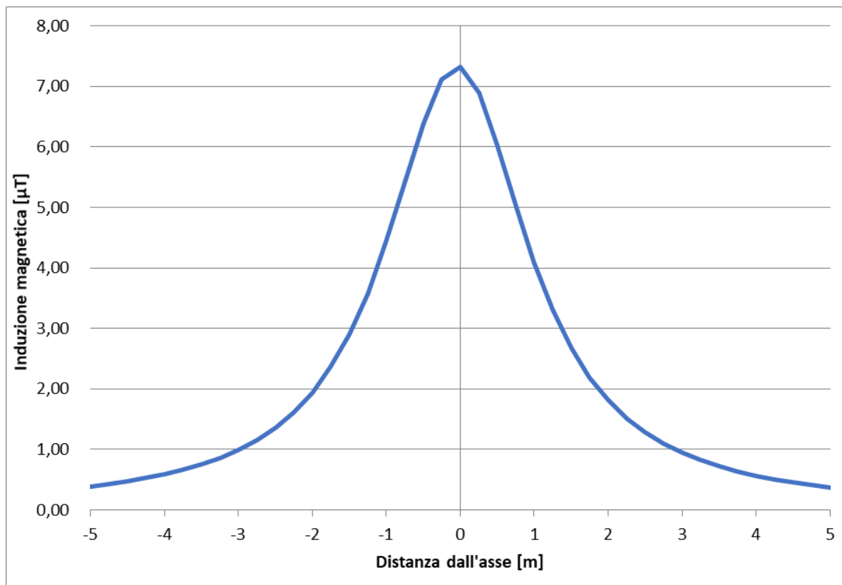
Figura 5-13 – Andamento campo magnetico – Sezione 9
