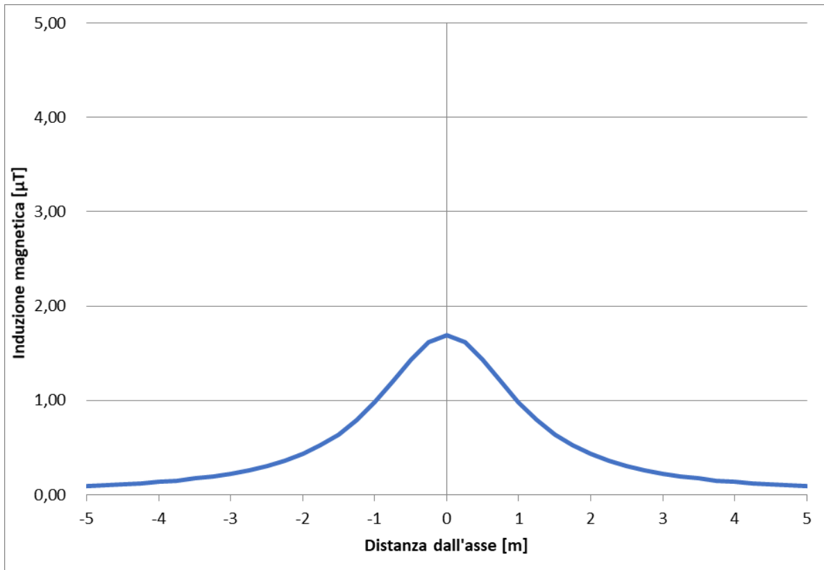
Figura 5-16 – Andamento campo magnetico – Sezione 12
