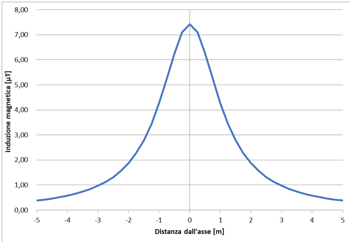
Figura 5-18 – Andamento campo magnetico – Sezione 14
