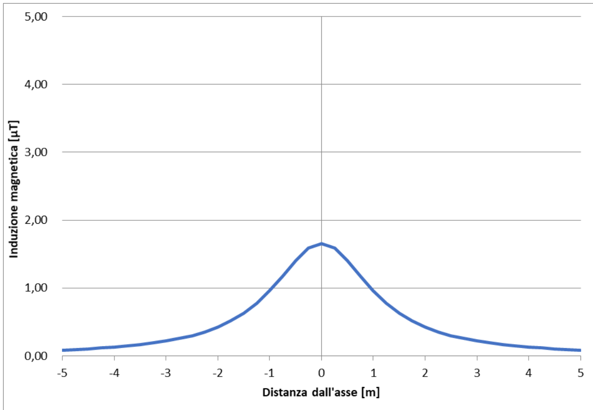
Figura 5-6 – Andamento campo magnetico – Sezione 2
