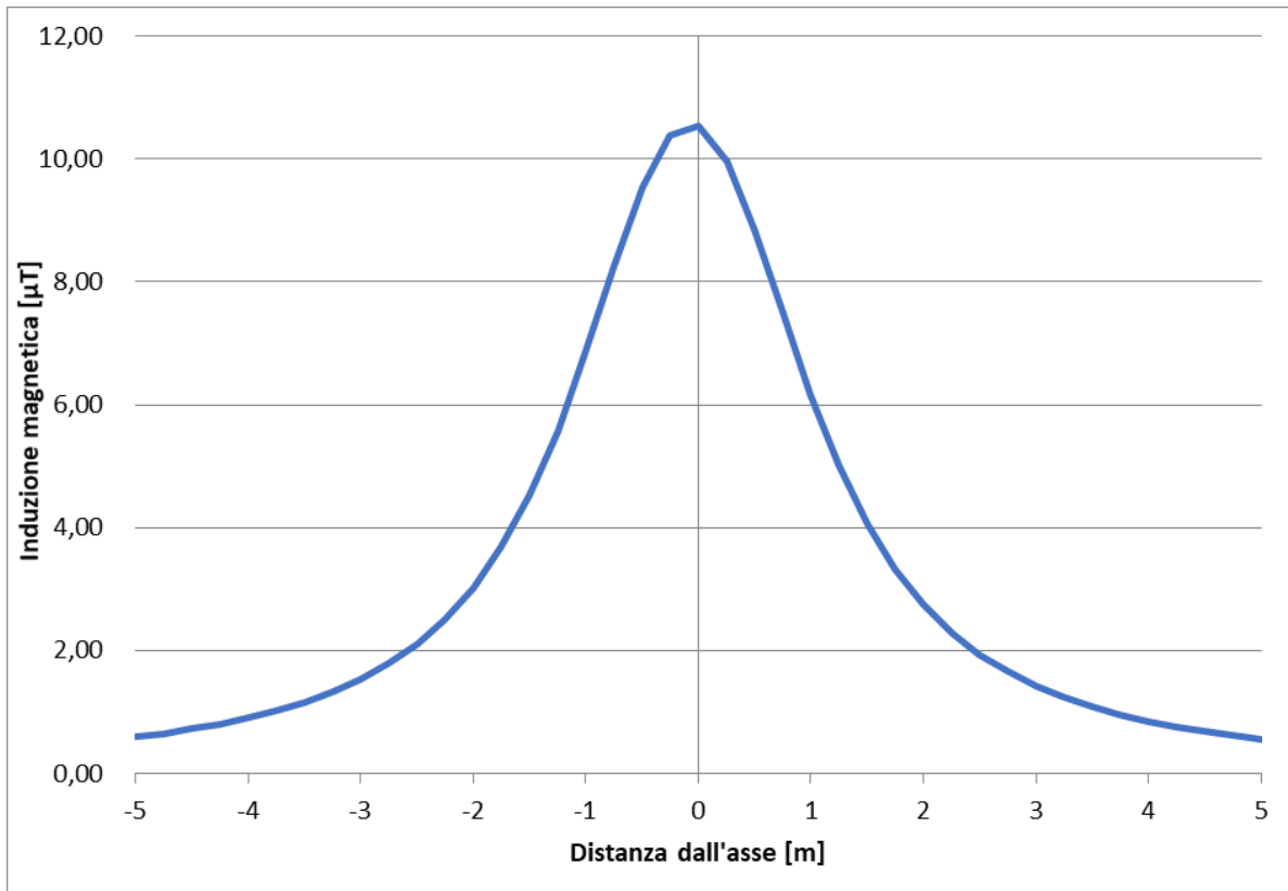
Figura 5-14 – Andamento campo magnetico – Sezione 10
