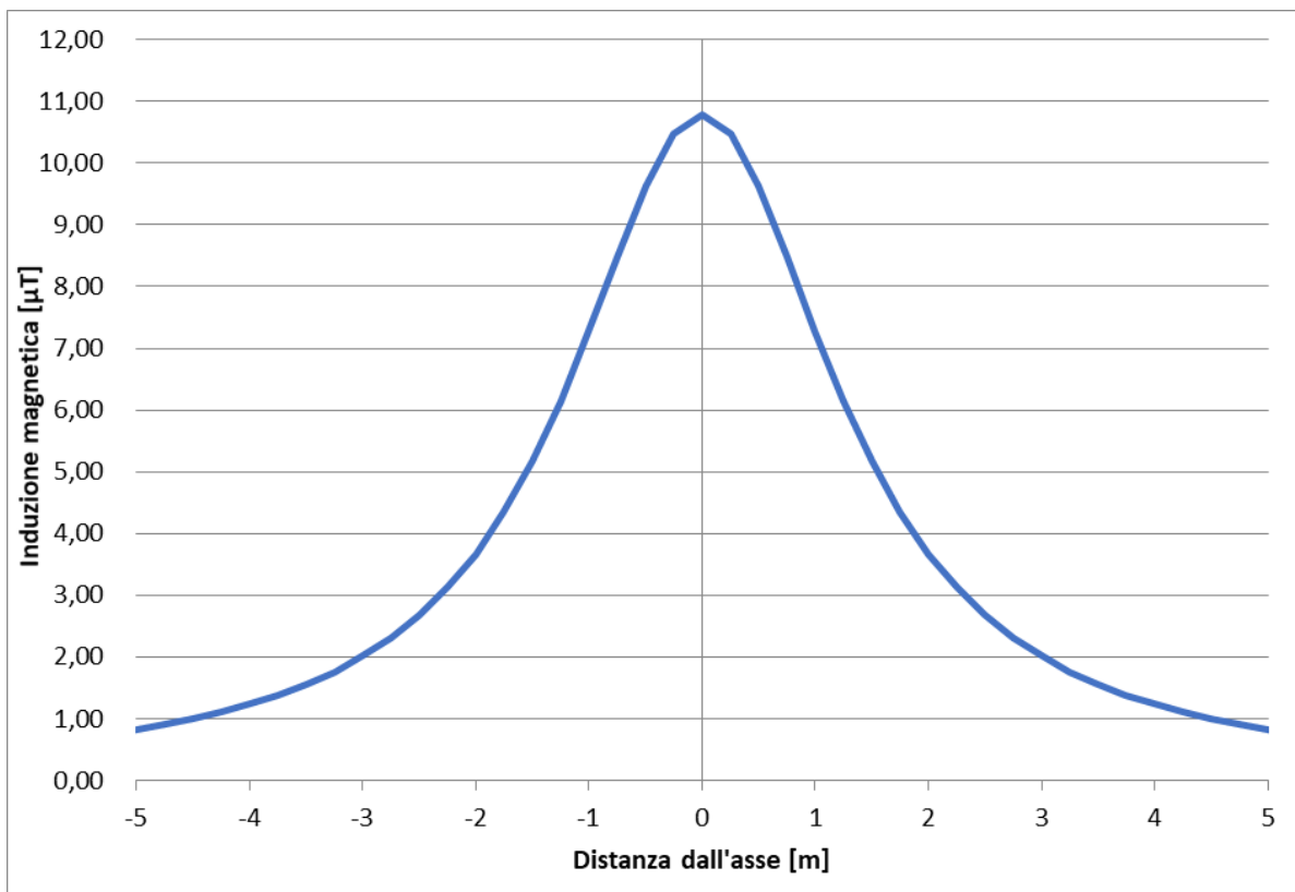
Figura 5-19 – Andamento campo magnetico – Sezione 15
