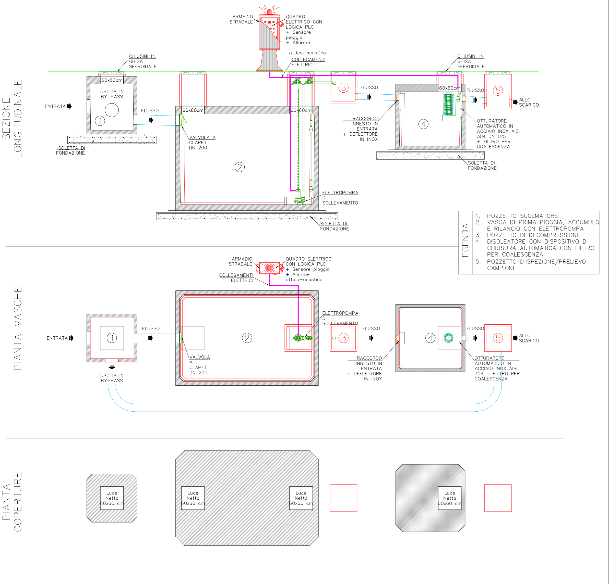
Dettaglio sistema di trattamento prima pioggia - Impianto di Storage - Scala 1:50
