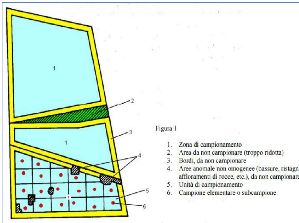
Figura 6-1 – Schema tipo per la definizione delle zone di campionamento. Fonte "Linee guida per il campionamento dei suoli e per l'elaborazione del piano di concimazione aziendale" Regione Sicilia
