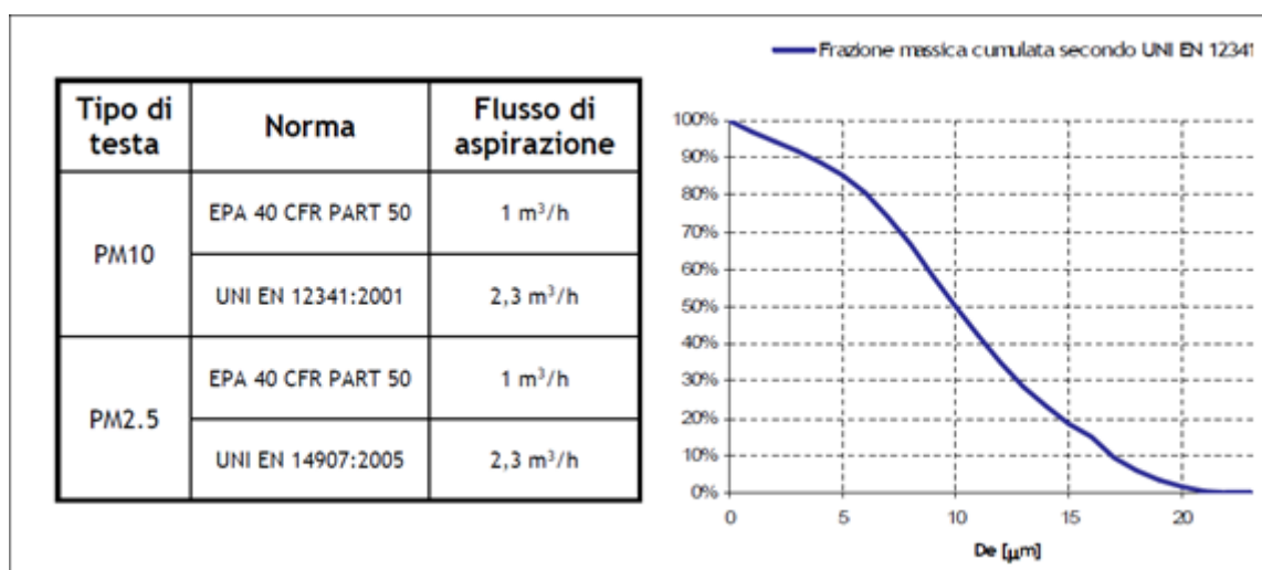
Figura 5-3 – Tipologia di Teste di Campionamento – Normativa di riferimento
