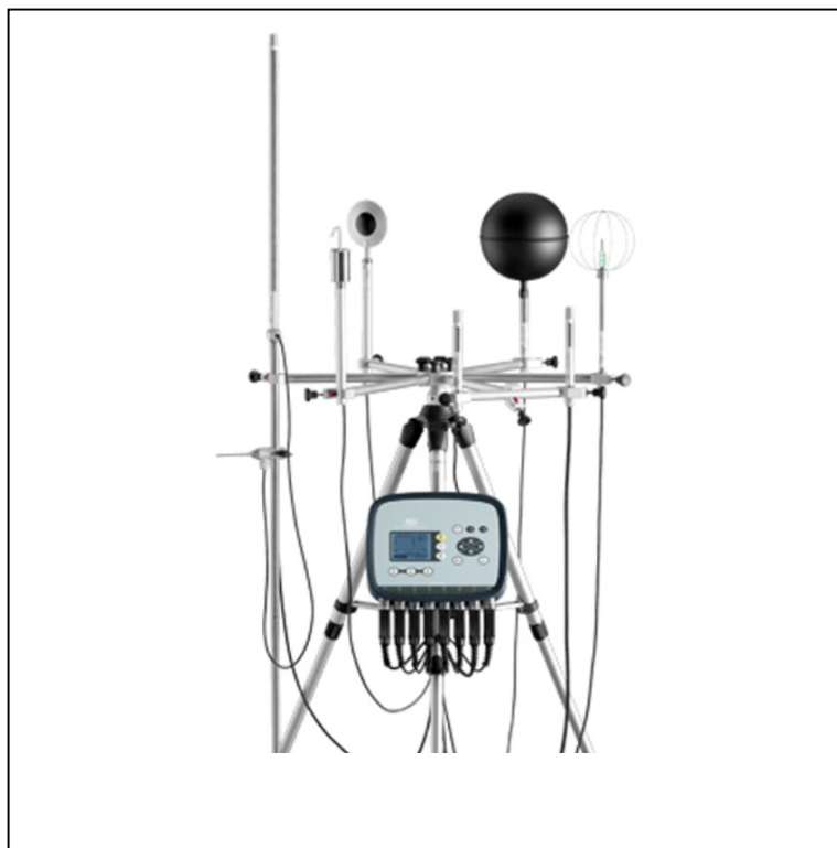
Figura 5-6 – Strumentazione modulare per la misurazione del microclima
