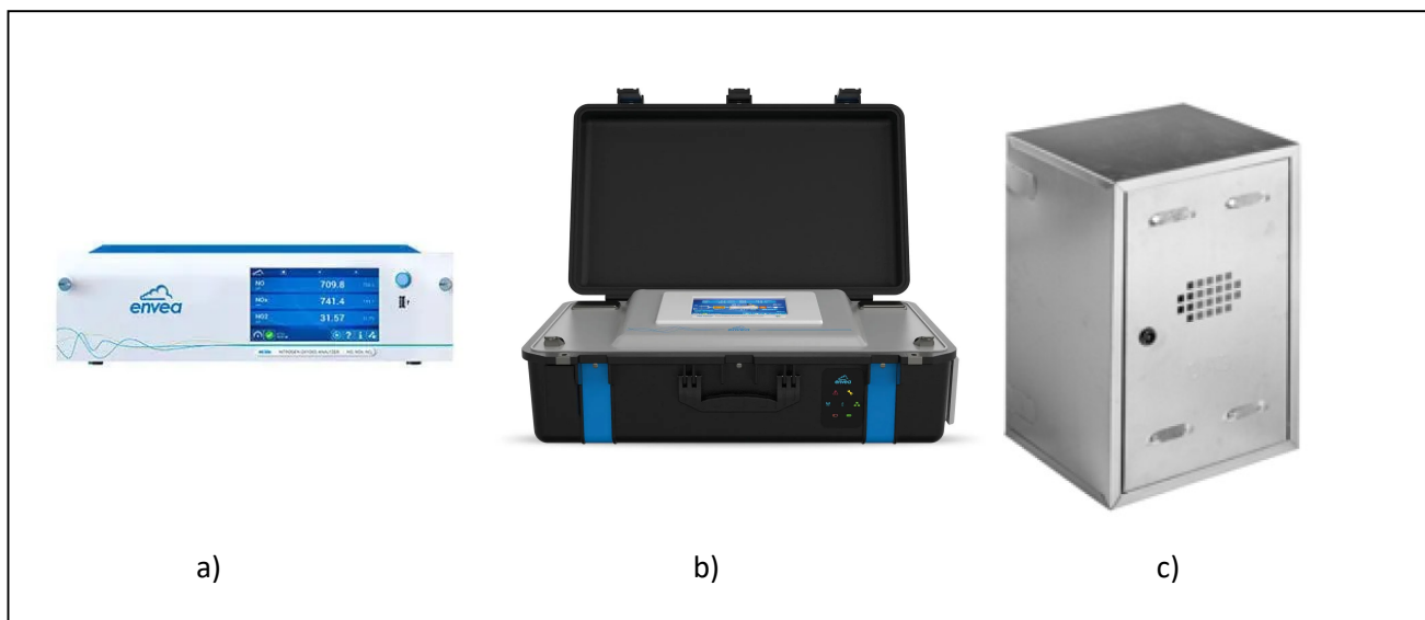
Figura 5-5 – Stazione mobile per il monitoraggio degli inquinanti da traffico veicolare. a) Misuratore ossidi di azoto a chemiluminescenza; b) Misuratore CO a infrarossi; c) cassetta zincata protezione sonde
