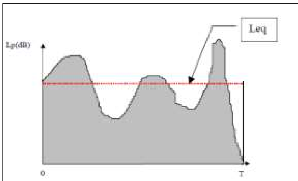
Figura 8-1 – Schema rappresentativo del L_{eq}
