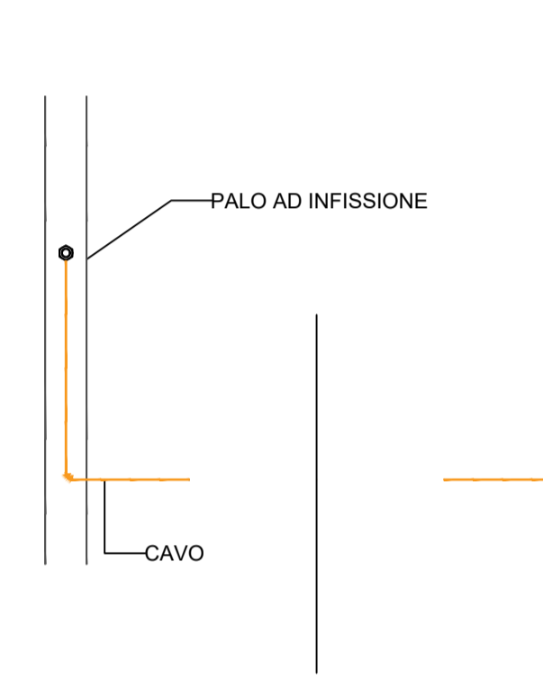
Schema collegamento strutture adiacenti
