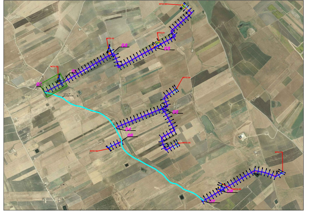
Sezione S6 - 00-WTG03
