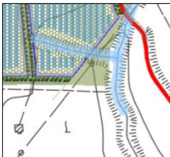
Figura 3: Planimetria su Ortofoto, Indicazione Accesso al Cantiere
