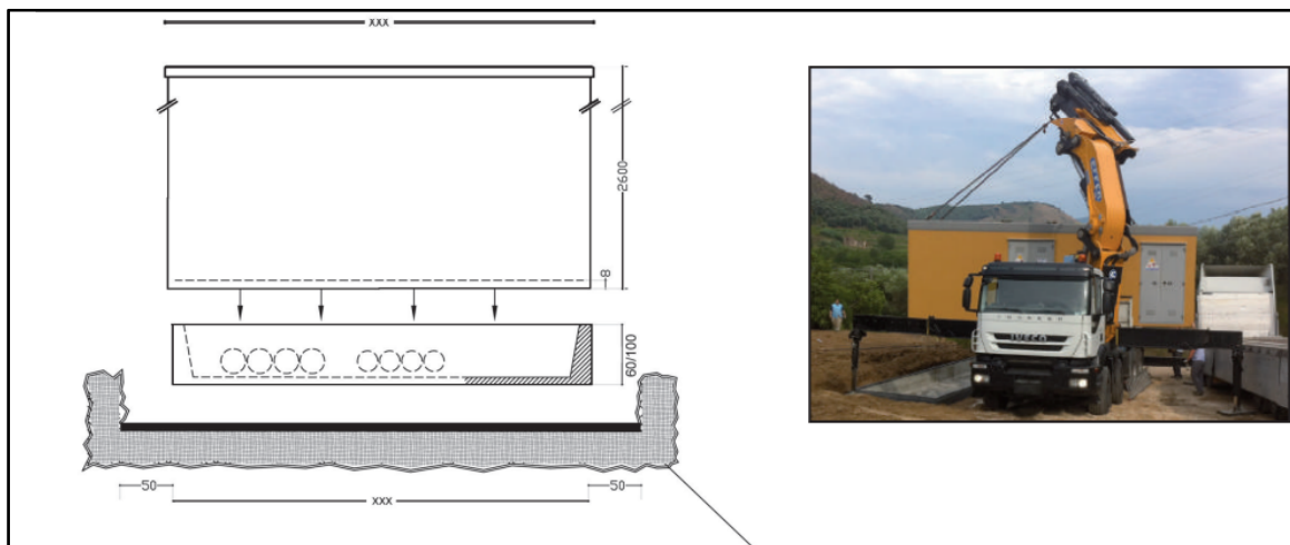
Figura 10: Esempio monobox cabina di raccolta
