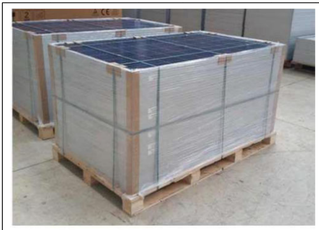
Figura 6: Impilamento e reggiatura dei pannelli fotovoltaici
