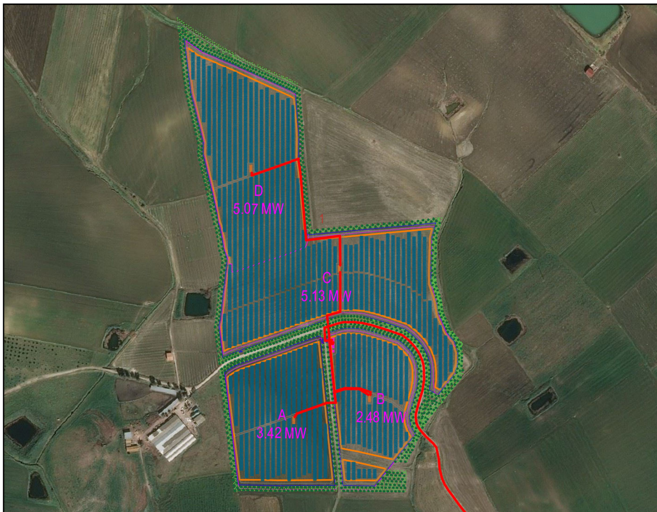
Figura 2: Layout del campo Agro-fotovoltaico e suddivisione in sottocampi
