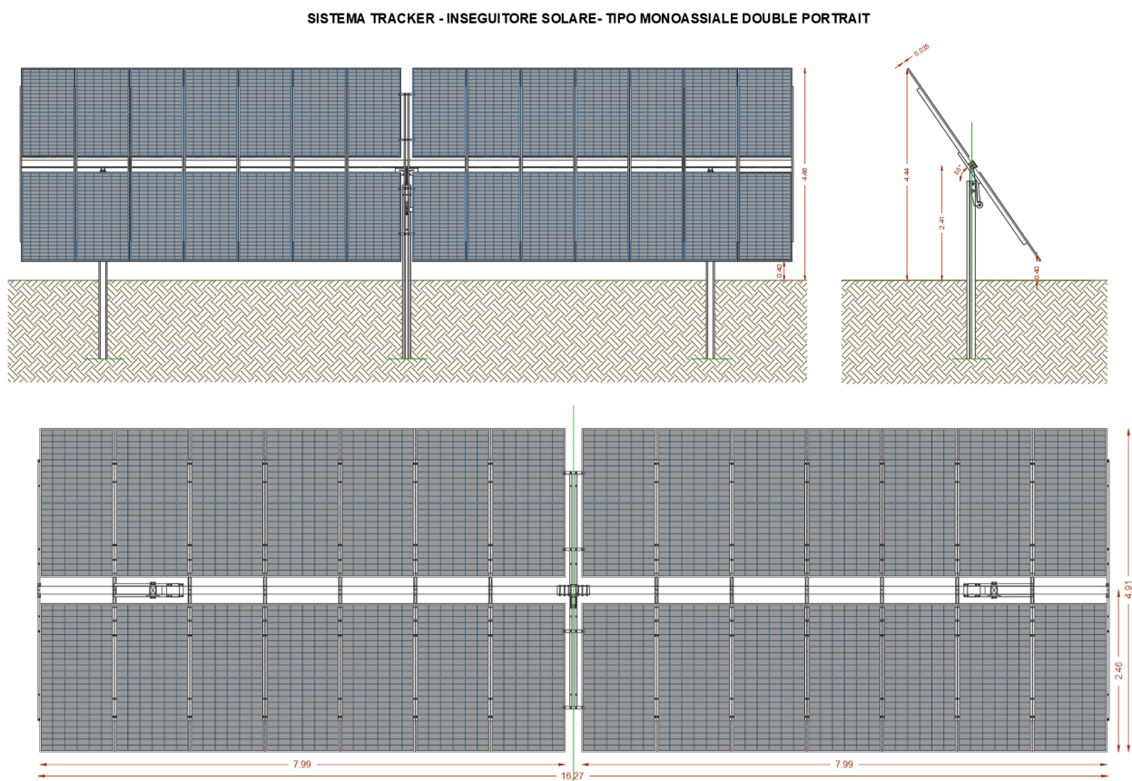
Figura 1: Pianta e prospetti quotati del tracker e dei moduli.
