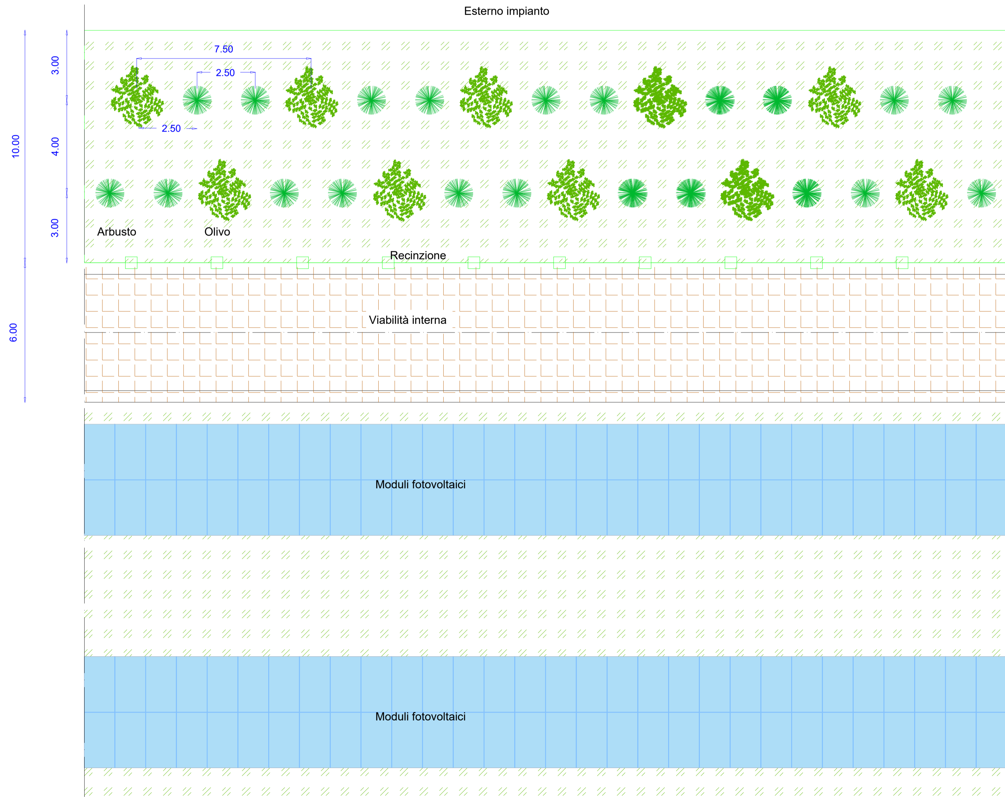
PIANTA
