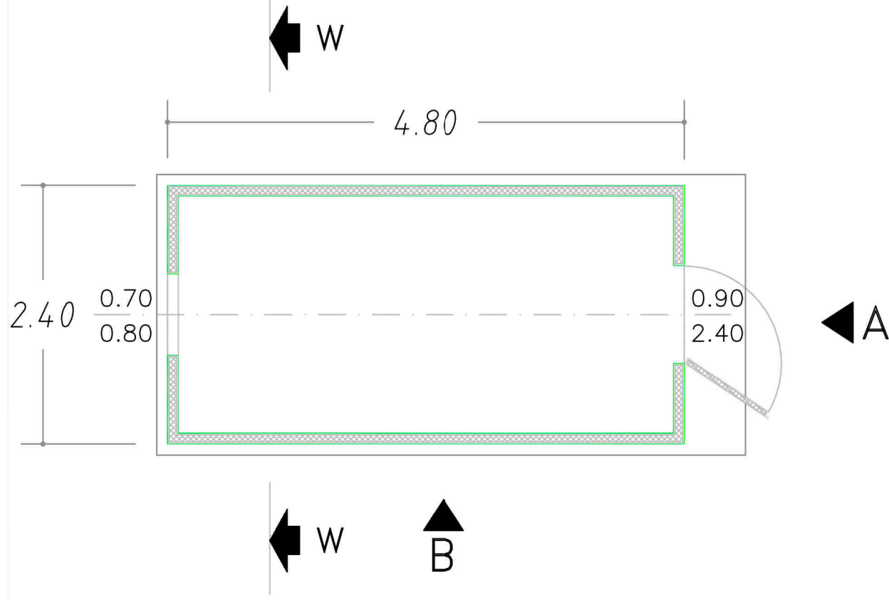
PIANTA
