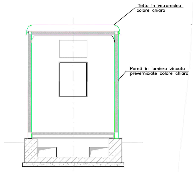
SEZIONE W-W
