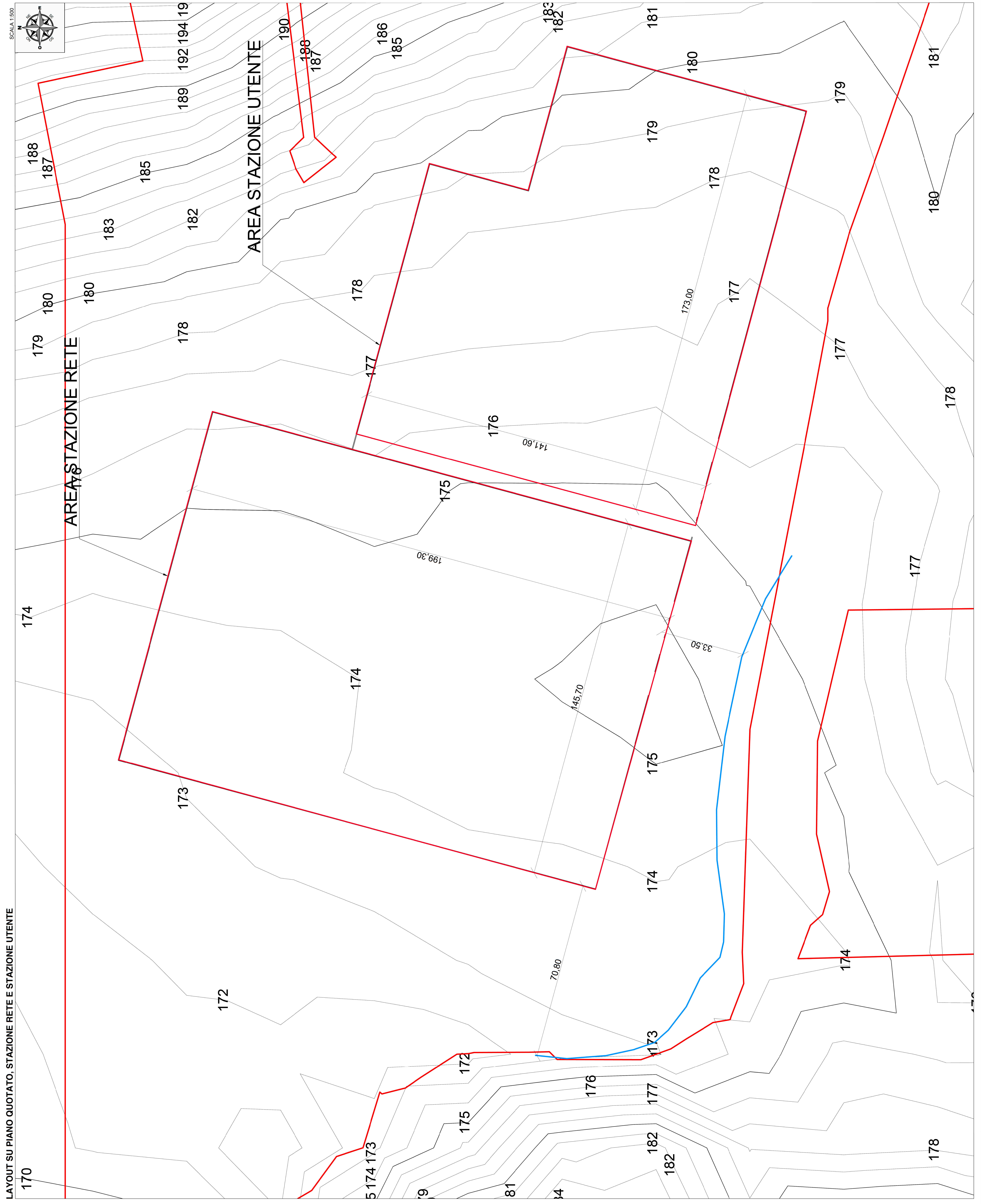
LAYOUT SU ORTOFOTO. STAZIONE RETE E STAZIONE UTENTE
