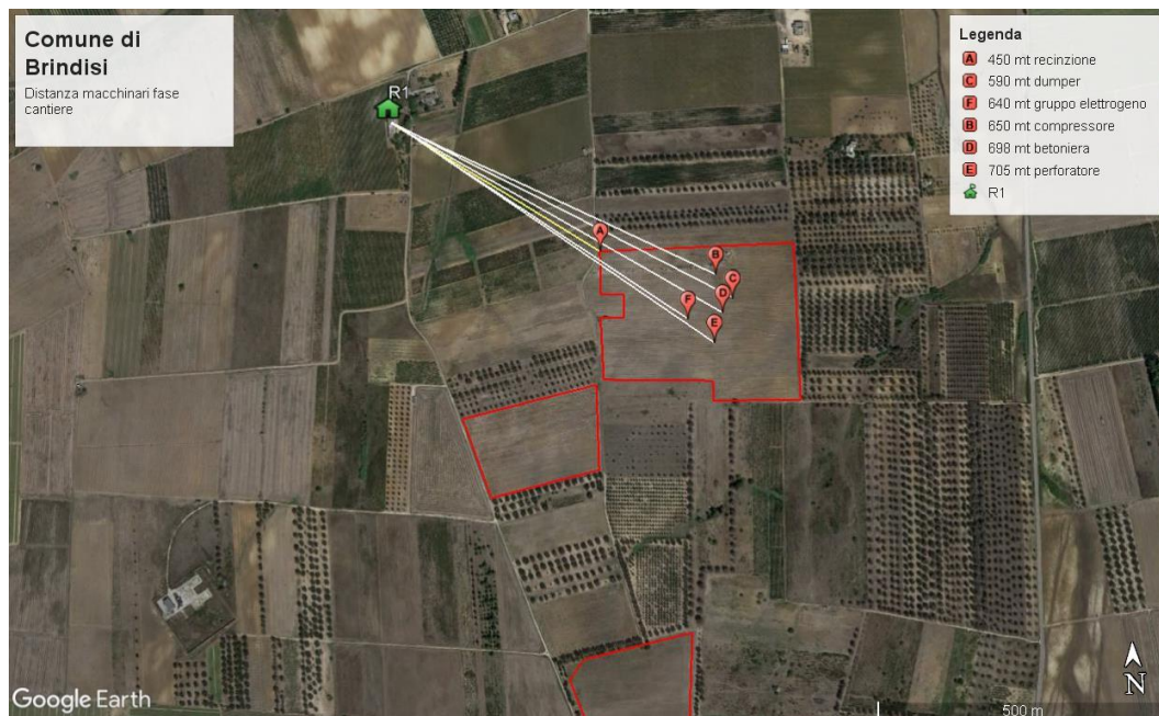
Figura 3 - distanziamento medio macchinari dal recettore sensibile più vicino
