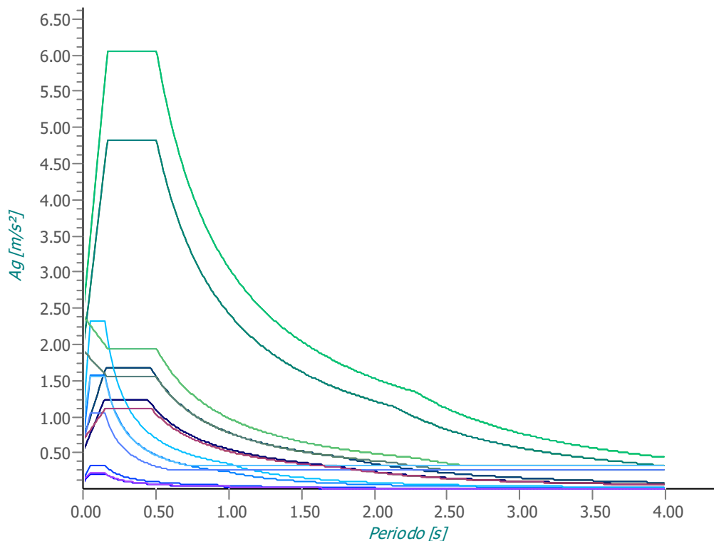
Grafico degli Spettri di Risposta
