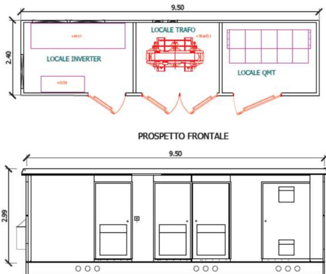
Figure 1: Pianta e prospetto Cabina Inverter e Trasformatore BT/MT
