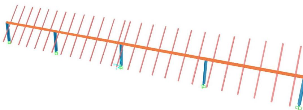
Figura 1 – Vista configurazione 55°_tracker 2x28 moduli
