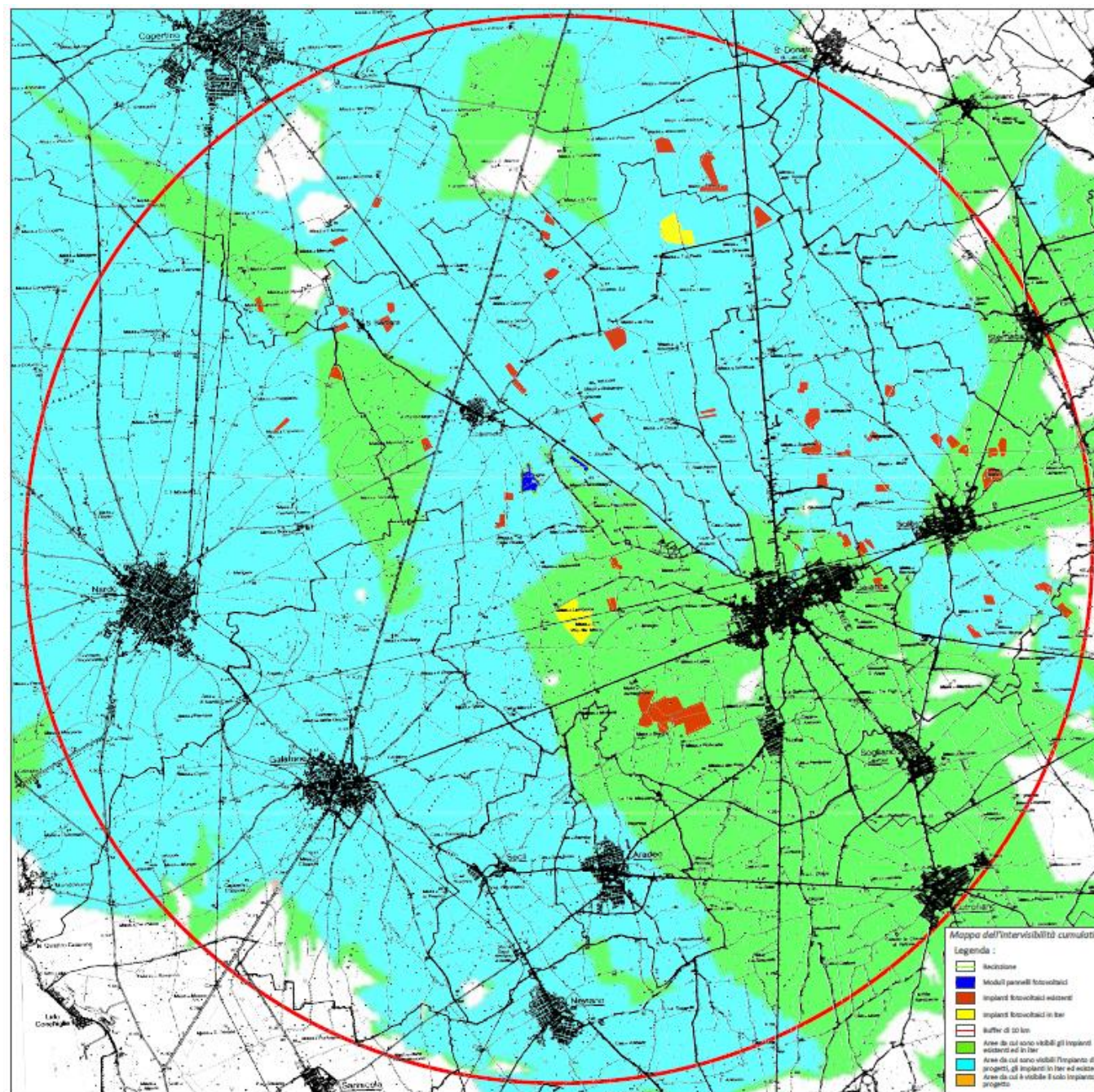
Mapa schematica dell'intervisibilità teorica generata dall'impianto di progetto rispetto a quelli esistenti, autorizzati e in iter autorizzativo.
