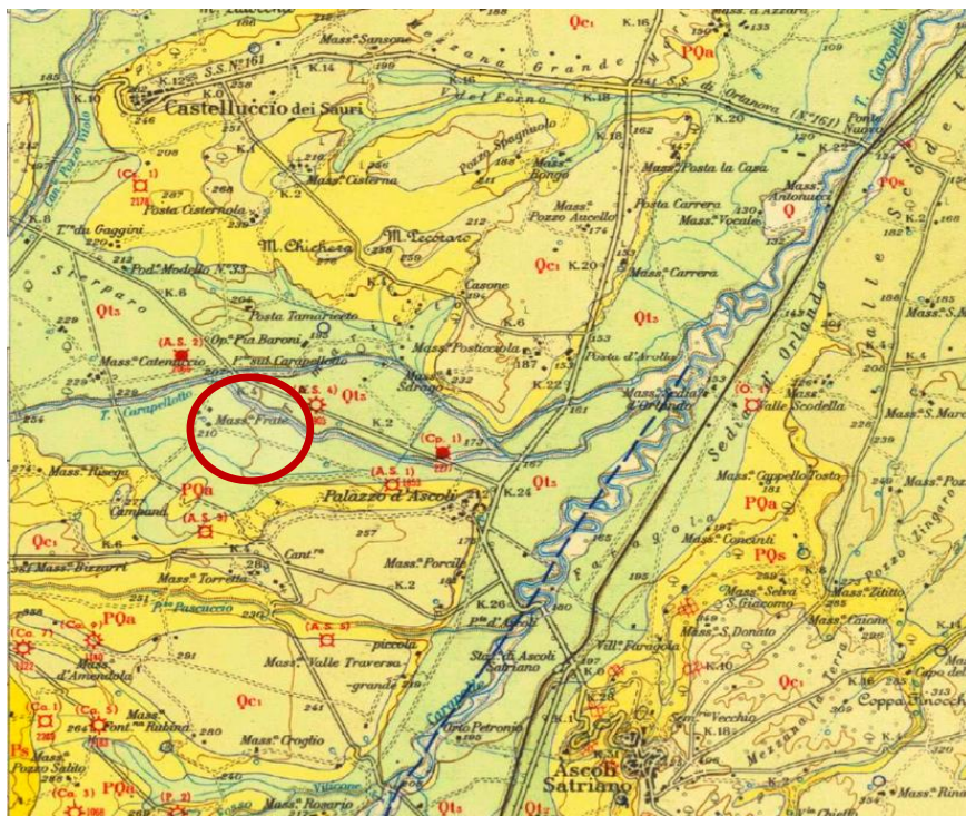
Area di progetto su Carta Geologica d'Italia, in scala 1.100.000, Foglio n. 175 Cerignola
