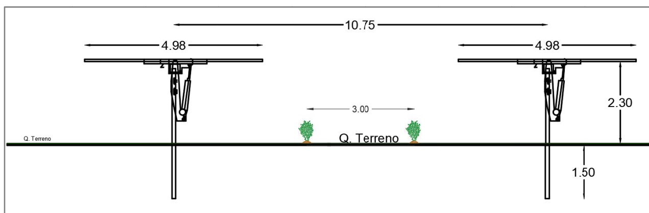
Figura 7: Rappresentazione in sezione di una fascia interfilare, con individuazione della superficie a cielo libero (circa 5 m).
