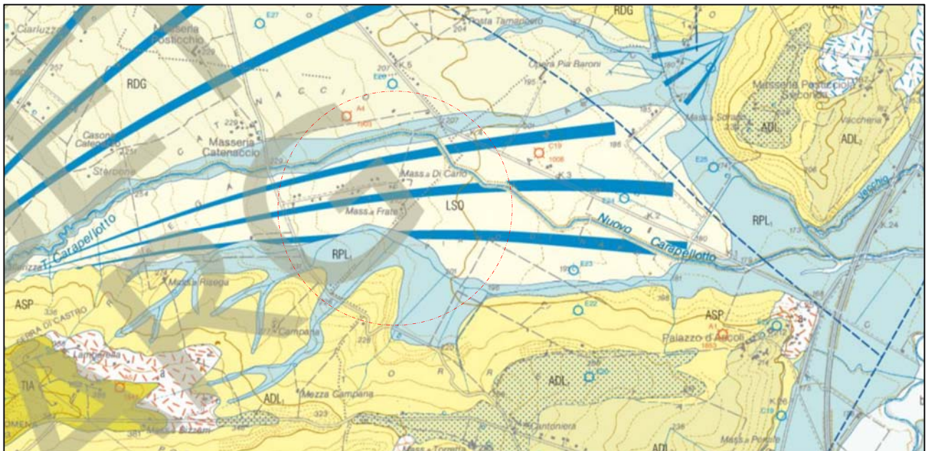
Stralcio della carta geologica d'Italia 1:50.000 "ASCOLI SATRIANO" N°421
