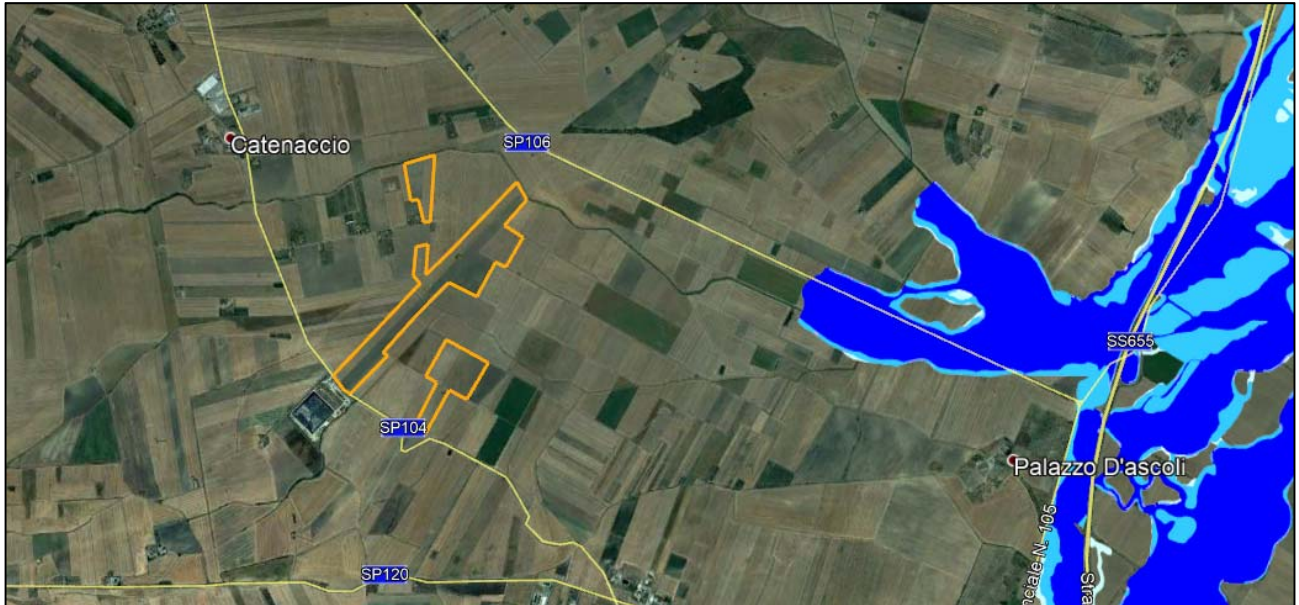
Stralcio pericolosità idraulica Autorità di Bacino Puglia su ortofoto
