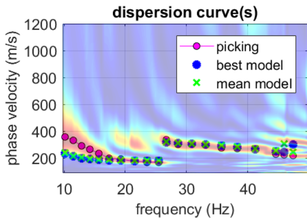
Fig. a - Spettro di velocità base sismica con picking.
